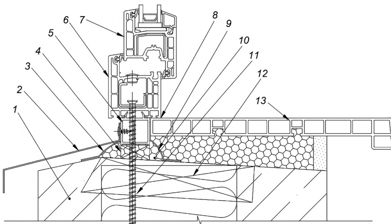
1 — стена; 2 — отлив; 3 — гидроизоляционная лента; 4 — опорная колодка; 5 — подставочный профиль; 6 — профиль коробки оконного блока; 7 — профиль створки оконного блока; 8 — герметик; 9 — пароизоляционная лента; 10 — монтажный шов; 11 — элемент крепления; 12 — закладной элемент стены; 13 — подоконная доска
