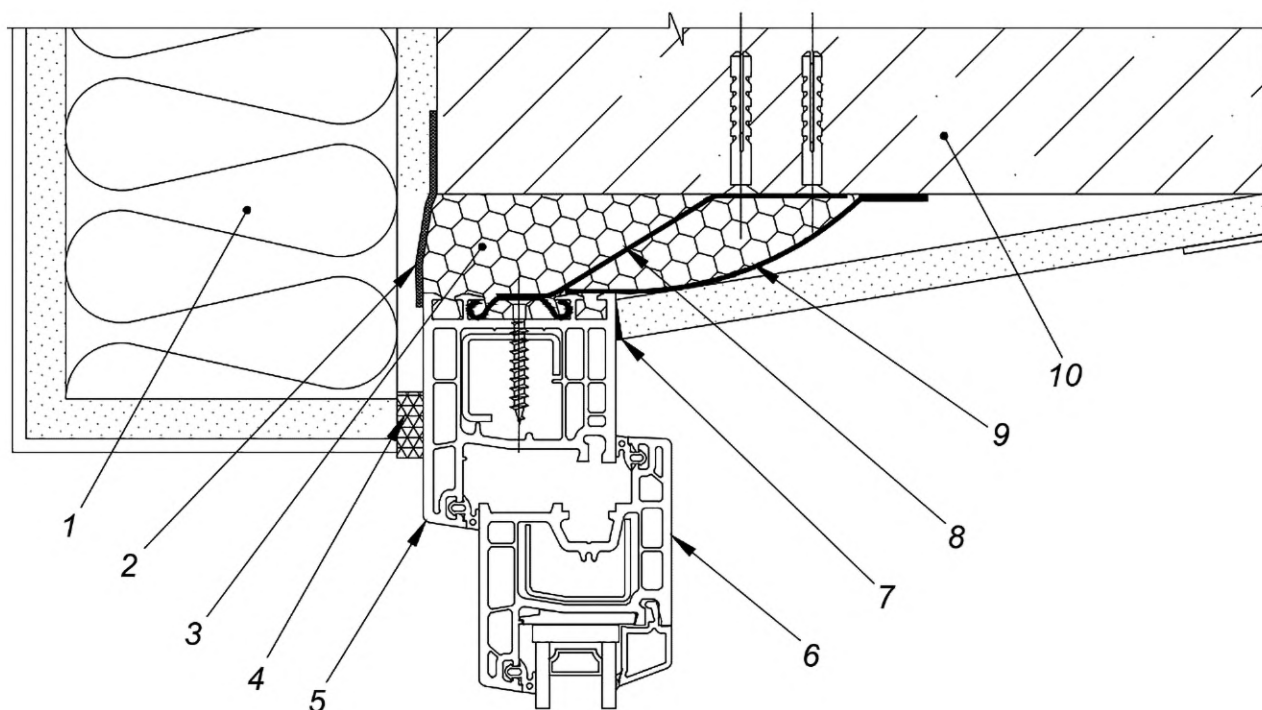
1 — теплоизолирующий слой; 2 — гидроизоляционная лента; 3 — монтажный шов; 4 — демпфирующая прокладка; 5 — профиль коробки оконного блока; 6 — профиль створки оконного блока; 7 — герметик; 8 — элемент крепления; 9 — пароизоляционная лента; 10 — стена
