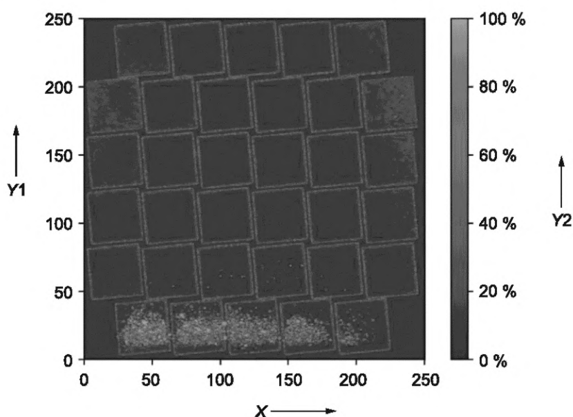
Рисунок 1 — Пример ультразвукового испытания при оценке поверхности построения
