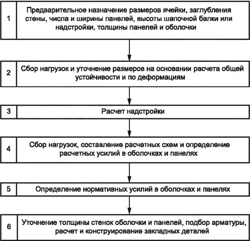
Рисунок 7 — Состав и рекомендуемая последовательность поверочных расчетов ячеистых подпорных стен и набережных
