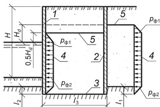
Рисунок 8 — Схема нагрузок от фильтрующей воды для расчета набережных ячеистых из плоских панелей и оболочек большого диаметра
