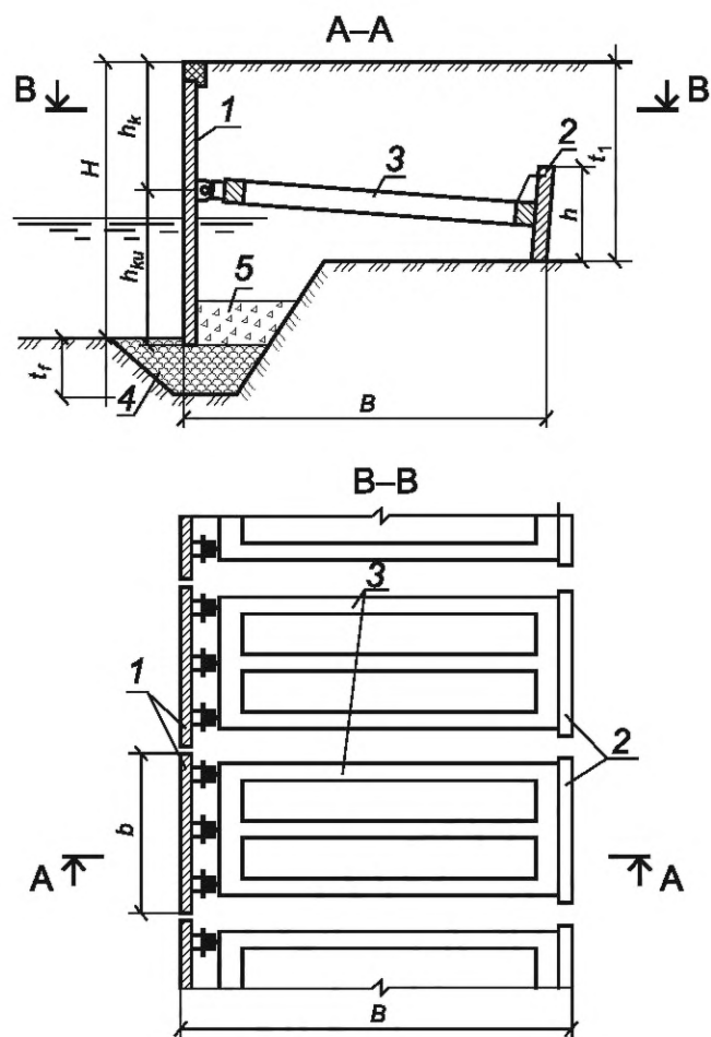
1 — лицевой элемент; 2 — анкерная плита; 3 — анкерная рама; 4 — каменная постель; 5 — обратный фильтр
