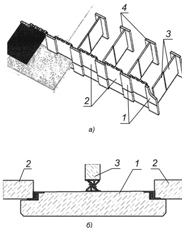
а) — общий вид; б) — конструкции вертикальных замков; 1 — железобетонная плита лицевая (опорная); 2 — железобетонная плита лицевая (забирка); 3 — железобетонная плита-перегородка (контрфорс); 4 — железобетонная анкерная плита
