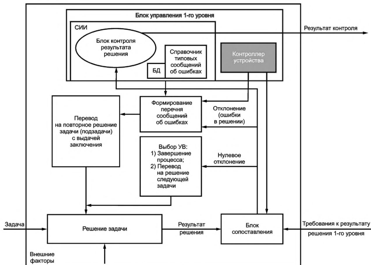
Рисунок 1 — Блок-схема требуемой последовательности решения задач (ТП) СИИ для СУ светолучевого устройства на первом уровне
