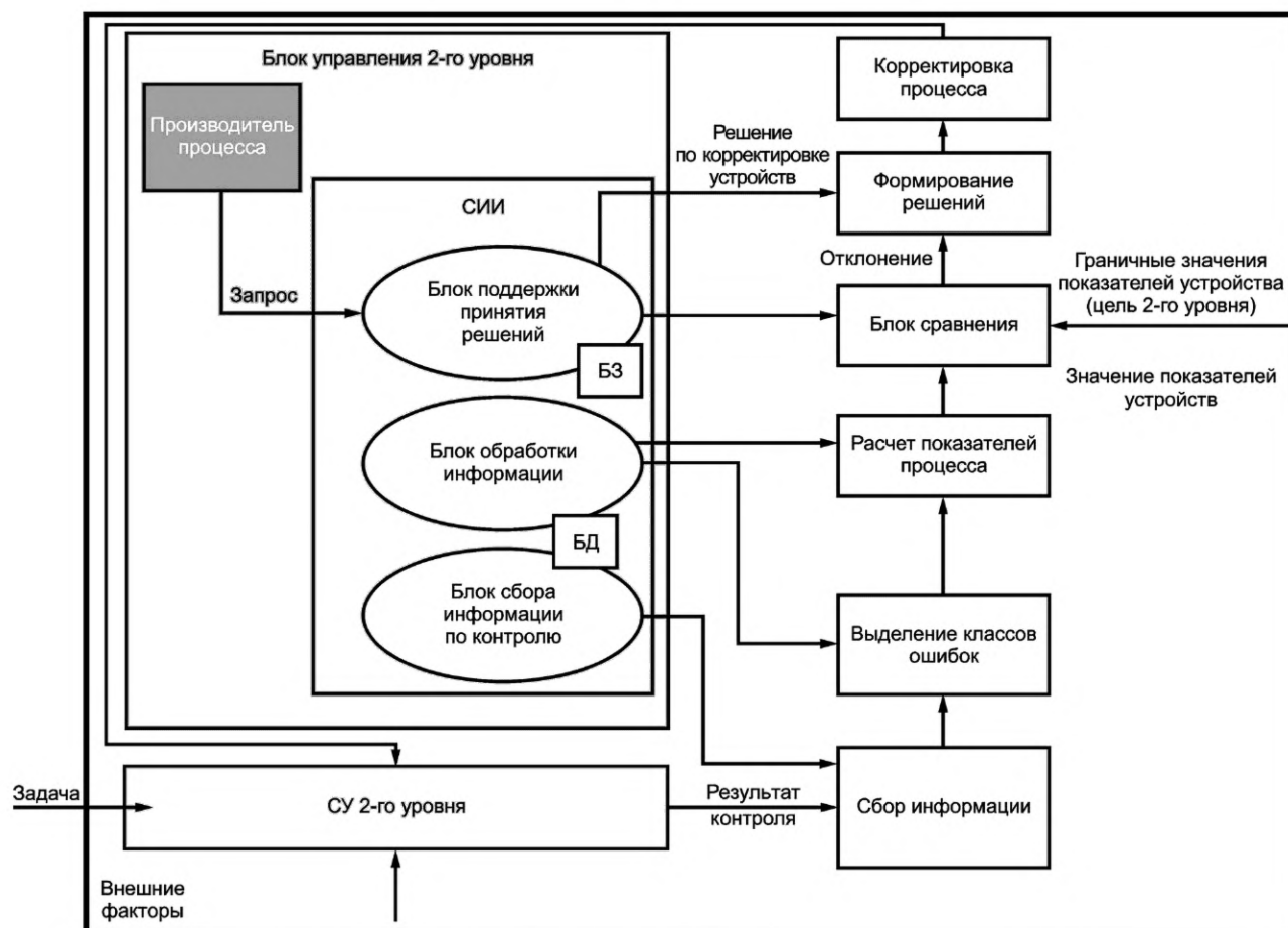
Рисунок 2 — Блок-схема требуемой последовательности решения задач (ТП) СИИ для СУ светолучевого устройства на втором уровне
