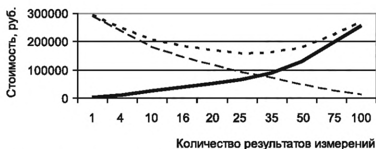
Рисунок А.1 — Соотношение цены и точности водного контроля
