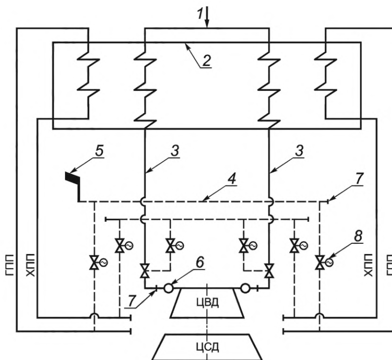
Рисунок 1 — Источники и схемы подачи пара к объекту очистки
