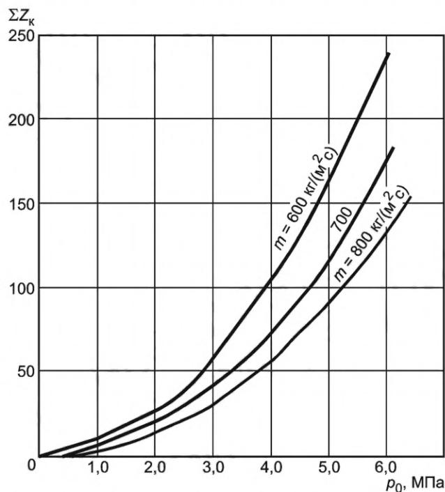
Рисунок 4 — Зависимость предельного коэффициента сопротивления Z_{\text{к}} очищаемого контура от давления и расхода пара ( p_0 ) на входе при температуре пара 450 °С
