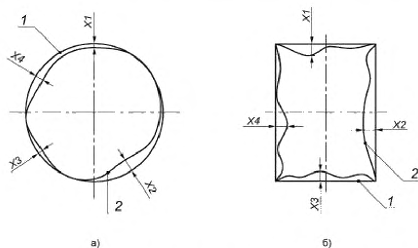
1 — воздуховод до теплового воздействия; 2 — воздуховод после теплового воздействия; а) — воздуховод круглого сечения; б) — воздуховод прямоугольного сечения; X1 , X2 , X3 , X4 — максимальные отклонения стенок воздуховода в результате деформации
