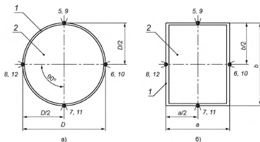
1 — огнезащитное покрытие воздуховода; 2 — воздуховод; D — диаметр поперечного сечения воздуховода круглого сечения; а) — воздуховод круглого сечения; б) — воздуховод прямоугольного сечения; a , b — размеры поперечного сечения воздуховода прямоугольного сечения; — ТЭП, установленные: - 5—8 — на необогреваемых поверхностях воздуховода на расстоянии 50 мм от узла пересечения ограждающей строительной конструкции огневой камеры; - 9—12 — то же, на расстоянии 1000 мм.
