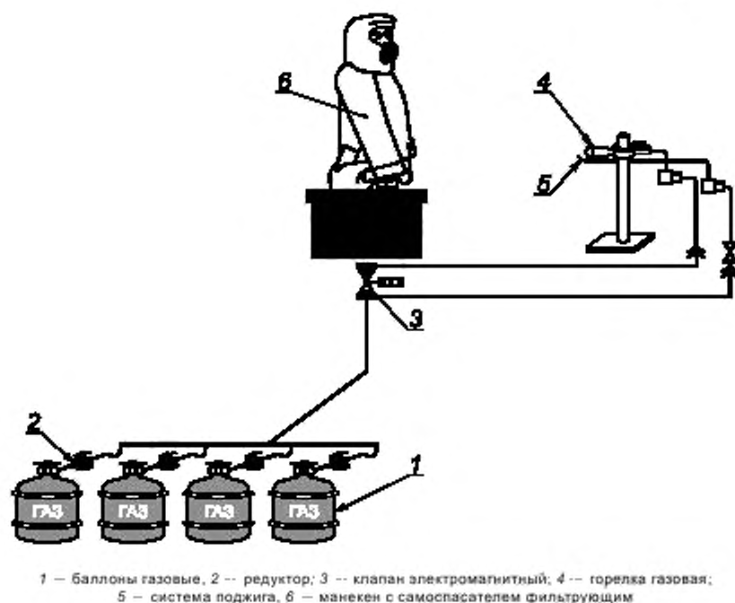
Рисунок А.1 — Схема стенда по определению устойчивости самоспасателя фильтрующего к воздействию пламени
