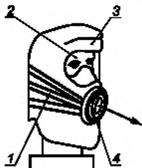
1 — система дополнительных ремней, снимающих нагрузку с капюшона, 2 — муляж головы человека; 3 — капюшон. 4 — фильтр
