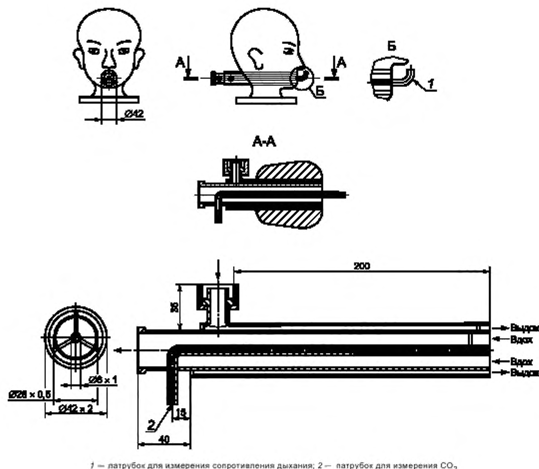
Рисунок 1 — Шеффилдский муляж головы человека
