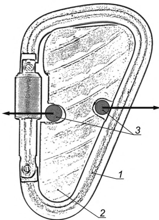
1 — карабин; 2 — оправка; 3 — силовые скобы
