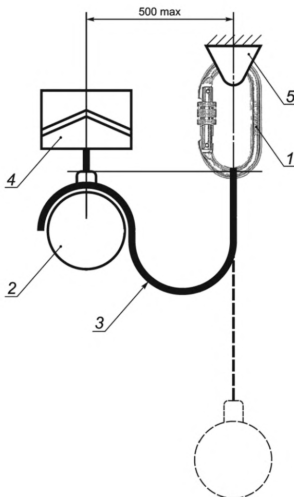
Рисунок 6 — Схема испытания карабина на динамическую прочность
