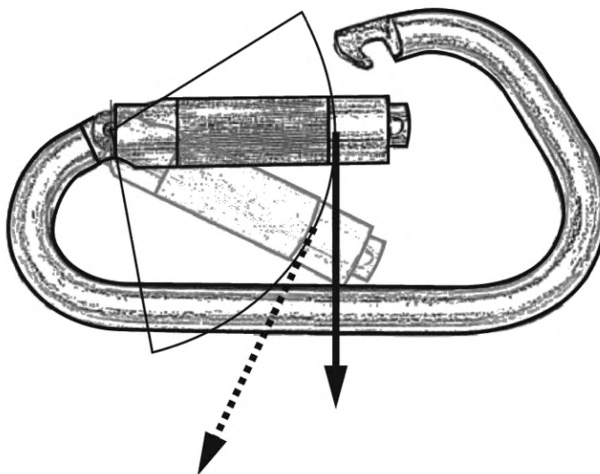
Рисунок 3 — Схема испытания усилия раскрытия затвора карабина
