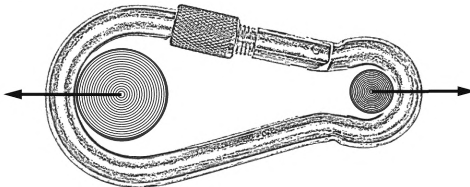
Рисунок 4 — Схема нагружения карабина по линии главной оси
