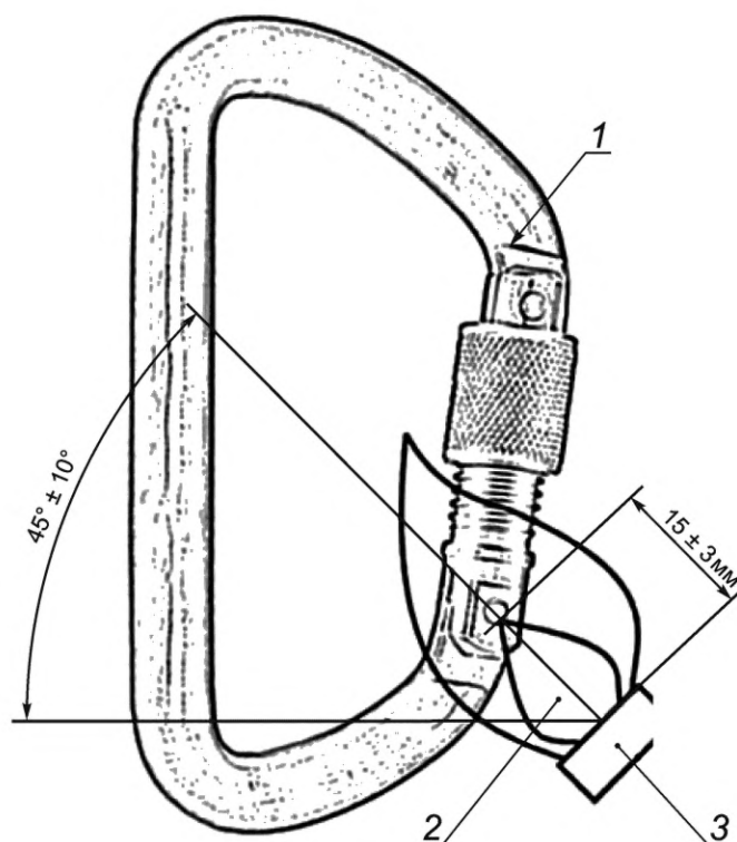
1 — карабин; 2 — голубой конус пламени; 3 — горелка Бунзена
