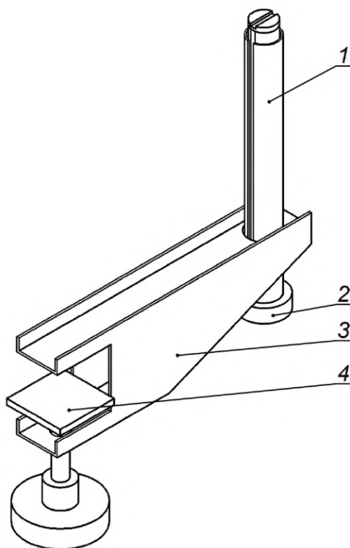
1 — вертикальная стойка; 2 — устройство регулировки высоты; 3 — горизонтальная часть; 4 — система крепления (хомут)
