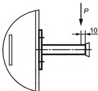
Рисунок 10 — Схема приложения статической нагрузки при испытаниях прочности крепления ножки стола
