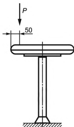
Испытуемый элемент — сиденье; масса груза P = 150 кг
