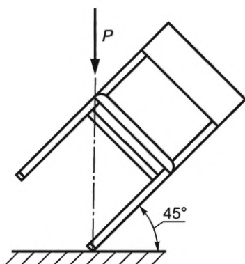
Испытуемый элемент – правые и левые боковые ножки; масса груза P = 120 кг
