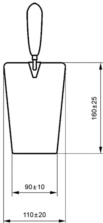
Рисунок 1 — Штукатурная лопатка
