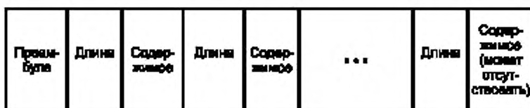
Рисунок 2 — Кодирование значения длинных данных
