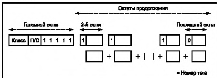
Рисунок 4 — Октет идентификатора (большой номер тега)
