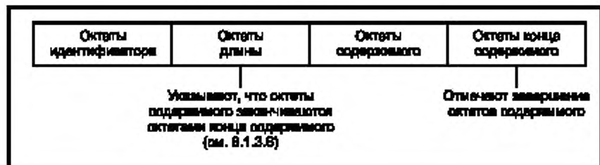
Рисунок 2 — Вариант составного кодирования
