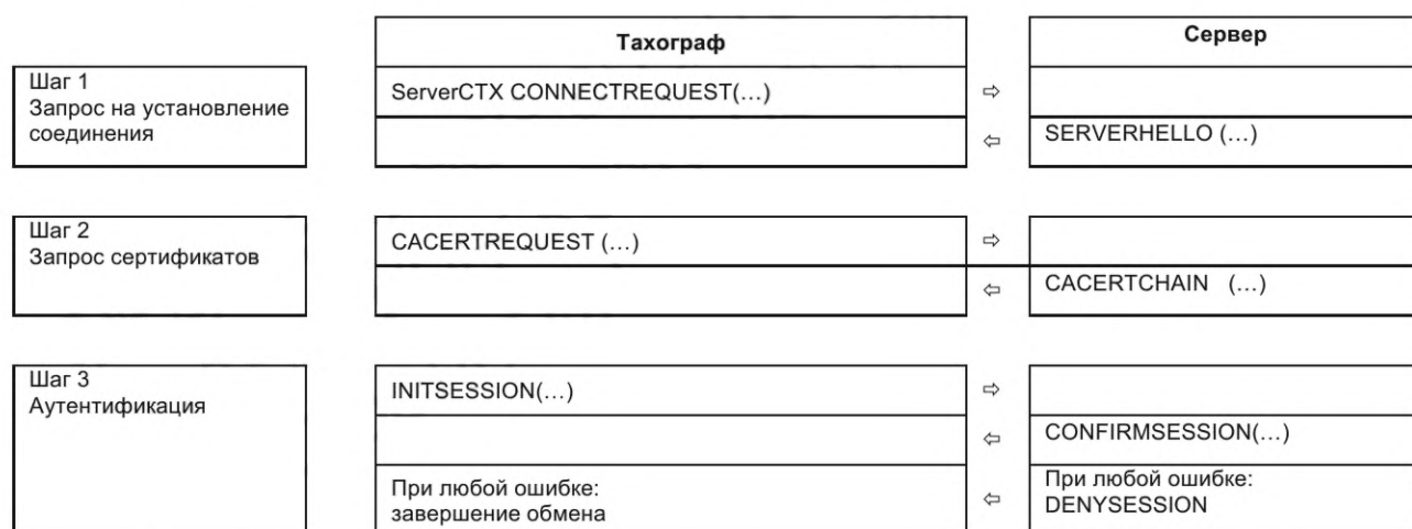
Рисунок 1 — Открытие сессии передачи тахографом подготовленных данных
