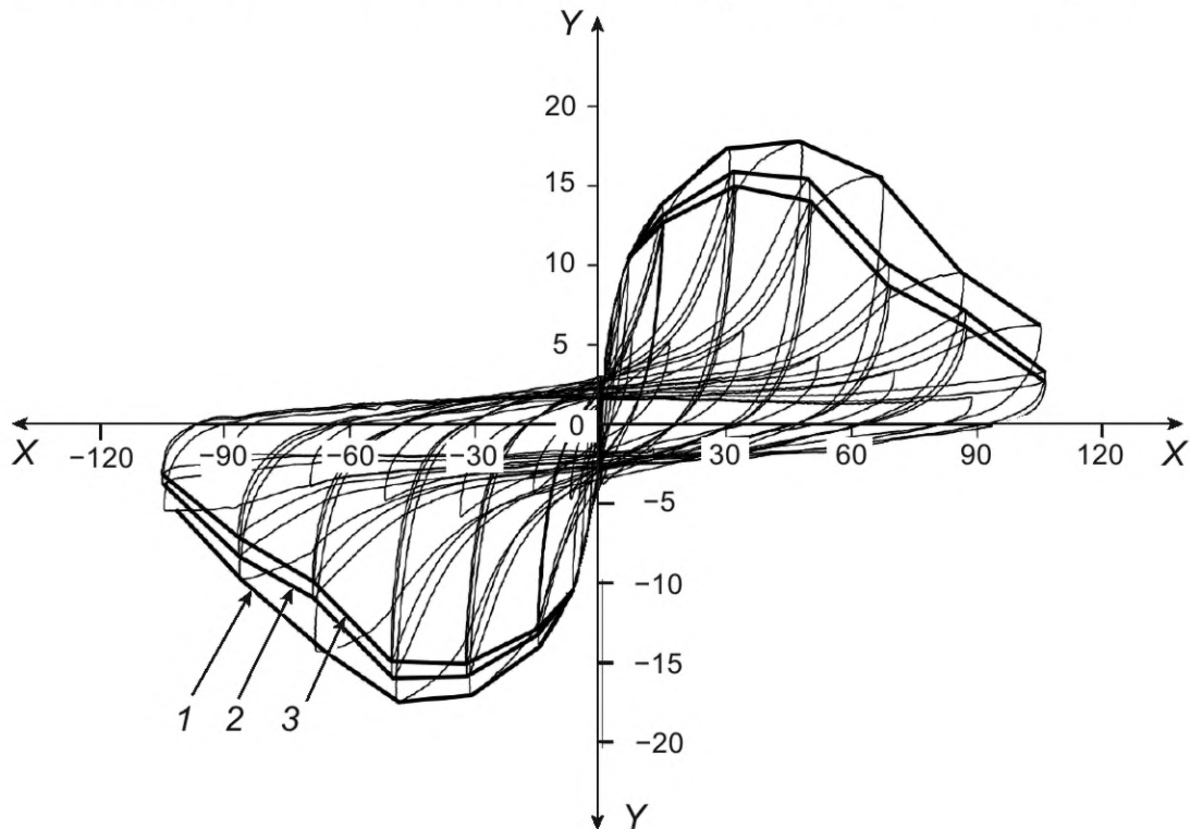
1 — первая огибающая кривая; 2 — вторая огибающая кривая; 3 — третья огибающая кривая; X — нагрузка F, кН/м; Y — смещение l, мм
