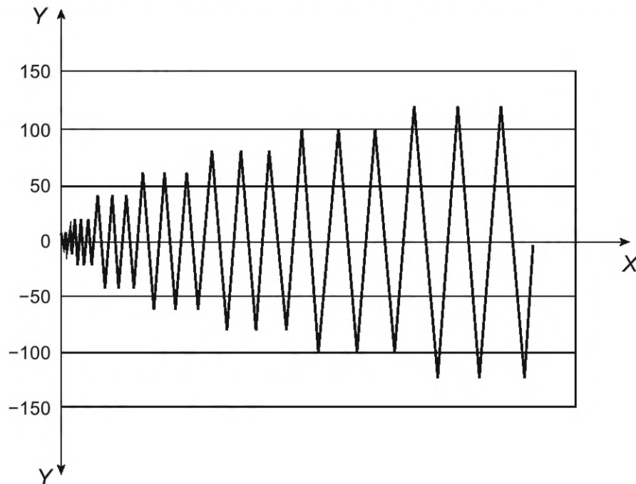
Рисунок 5 — График деформирования образца при циклических нагрузках
