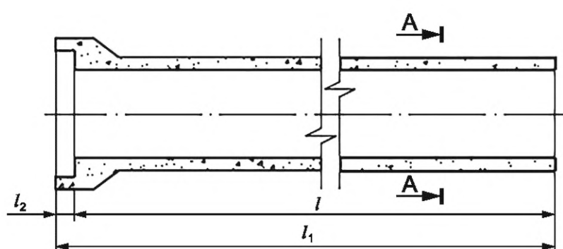
Рисунок А.2 — Общий вид труб типа БДТ
