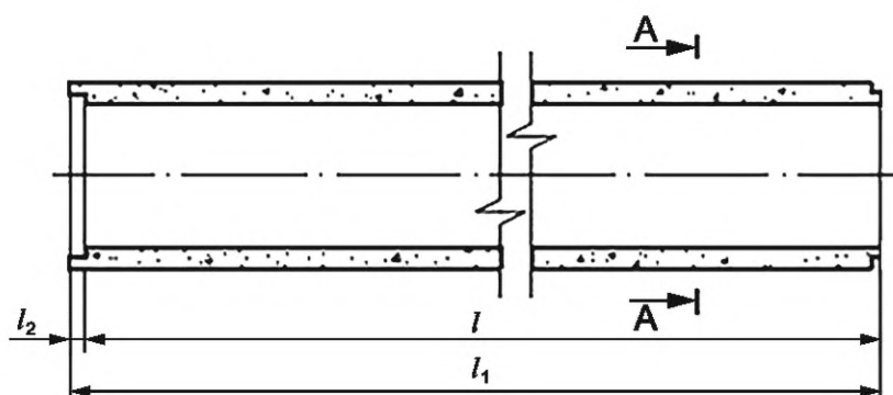
Рисунок А.1 — Общий вид труб типа БДТФ
