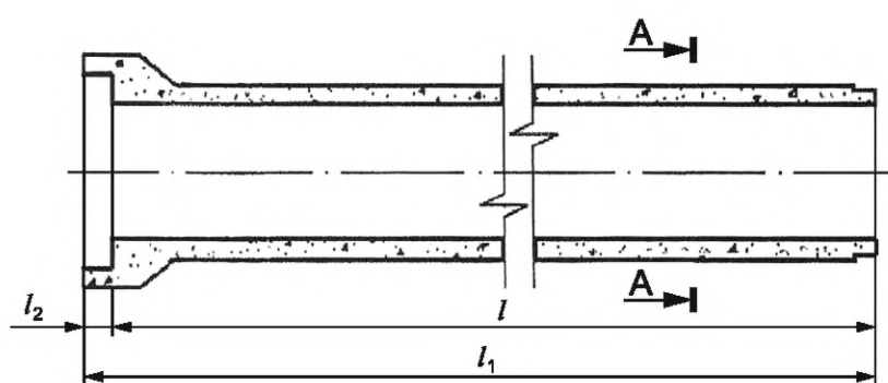
Рисунок А.3 — Общий вид труб типа БДТС
