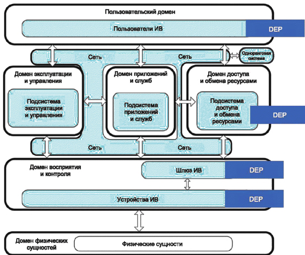
Рисунок 4 — Функции DEP в типовых моделях ИВ
