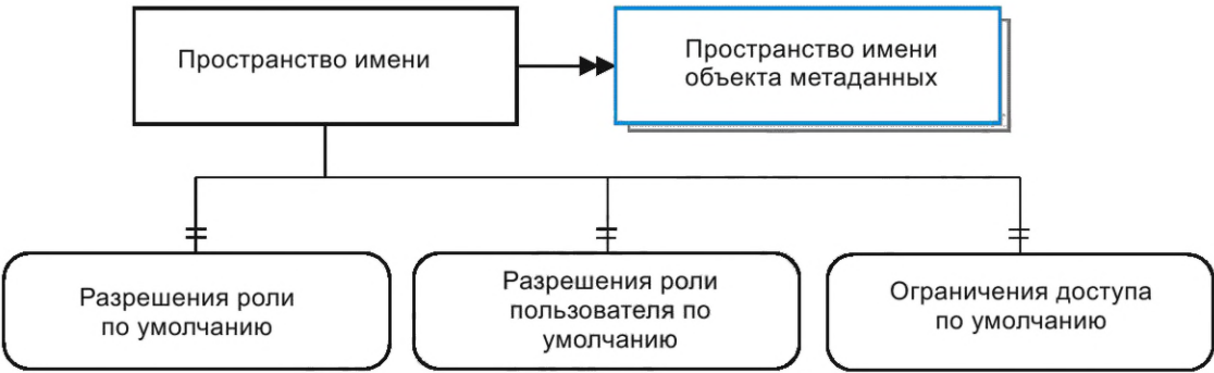
Рисунок 6 — Разрешения в адресном пространстве
