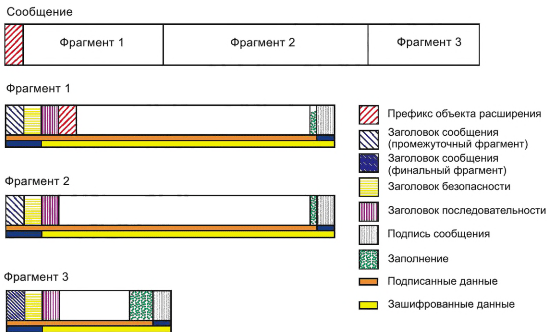
Рисунок 12 — Структура сообщения протокола соединения OPC UA
