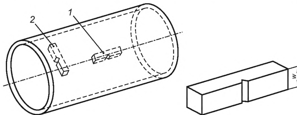
1 — продольный образец; 2 — поперечный образец; w — ширина образца
