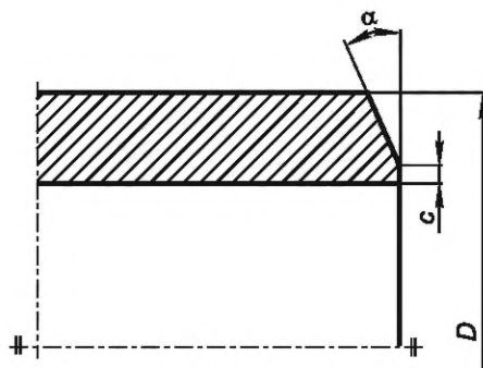
Рисунок 1 — Отделка концов труб
