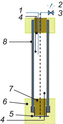
1 — подача жидкого азота; 2 — расходомер; 3 — выпуск газообразного азота; 4 — температура среды T_c ; 5 — концевое соединение; 6 — наружная изоляция; 7 — изоляция; 8 — температура внешней поверхности шланга T_{вн}
