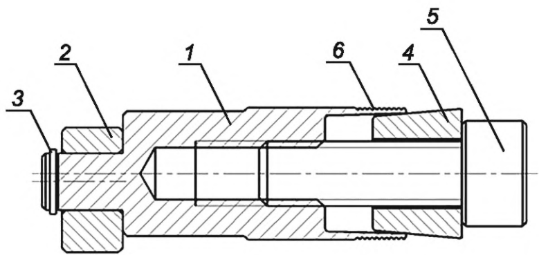
а) ПЗВ исполнения 1 для глушения теплообменной трубы
