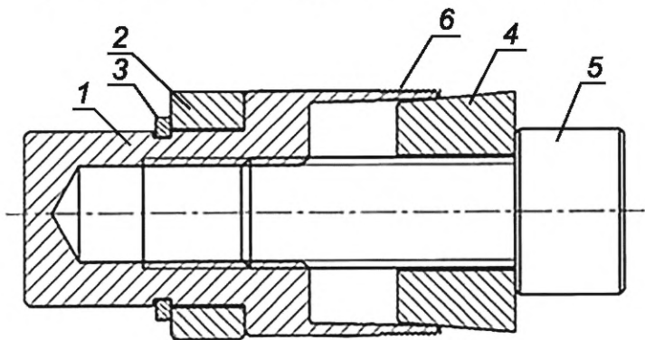
б) ПЗВ исполнения 2 для глушения отверстия трубной решетки
