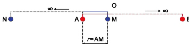
Рисунок 4 — Схема потенциал-установки
