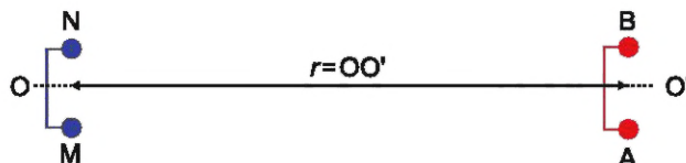
Рисунок 6 — Схема дипольной экваториальной установки зондирования
