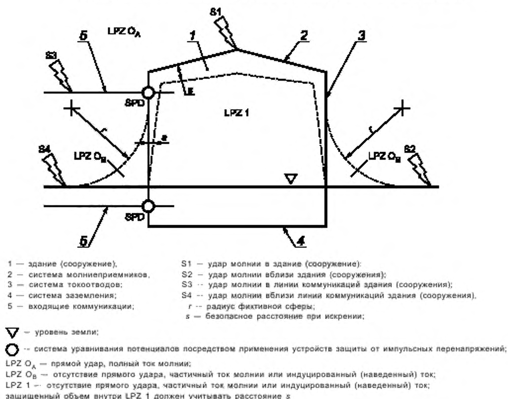
Рисунок 3 — Зона защиты от молнии, определенная в соответствии с LPS (МЭК 62305-3)
