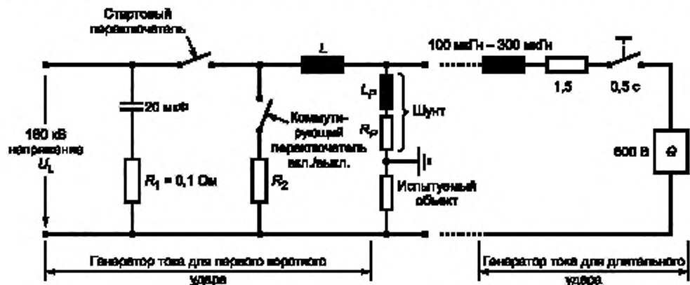
Рисунок С.1 — Пример генератора, используемого для моделирования удельной энергии тока первого положительного импульса и заряда длительного удара
