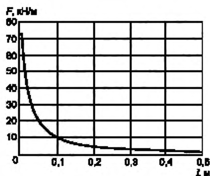
Рисунок D.4 — График зависимости силы на единицу длины F для горизонтального проводника, изображенного на рисунке D.2
