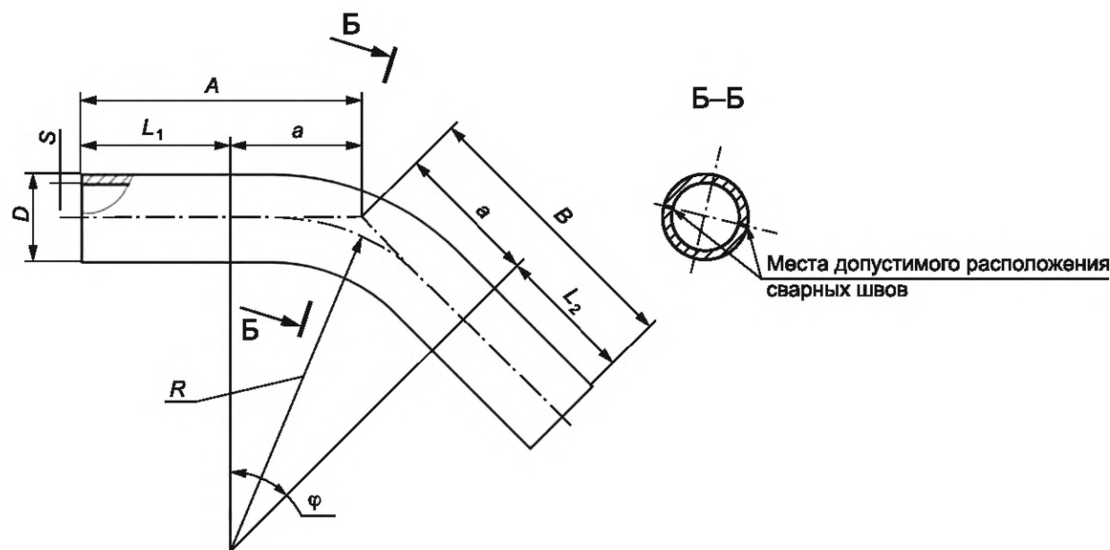
Рисунок 4 — Отвод горячегогнутый
