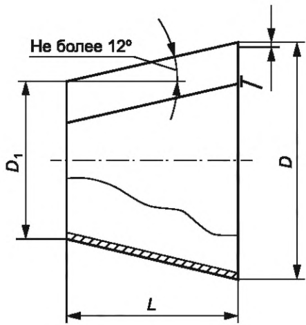
б) Переходы сварные концентрические
