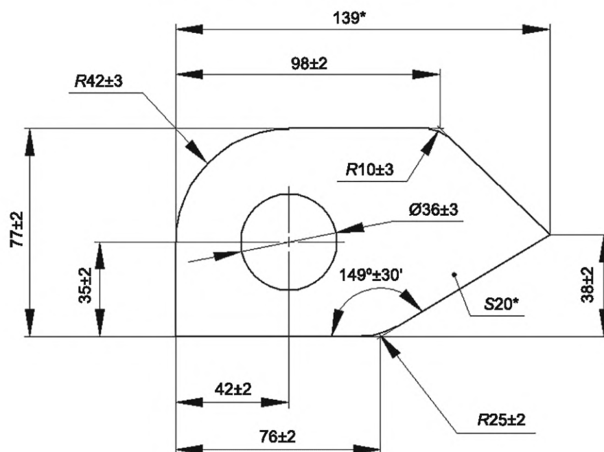
Рисунок 14 — Увязочные кольца типов I и II
