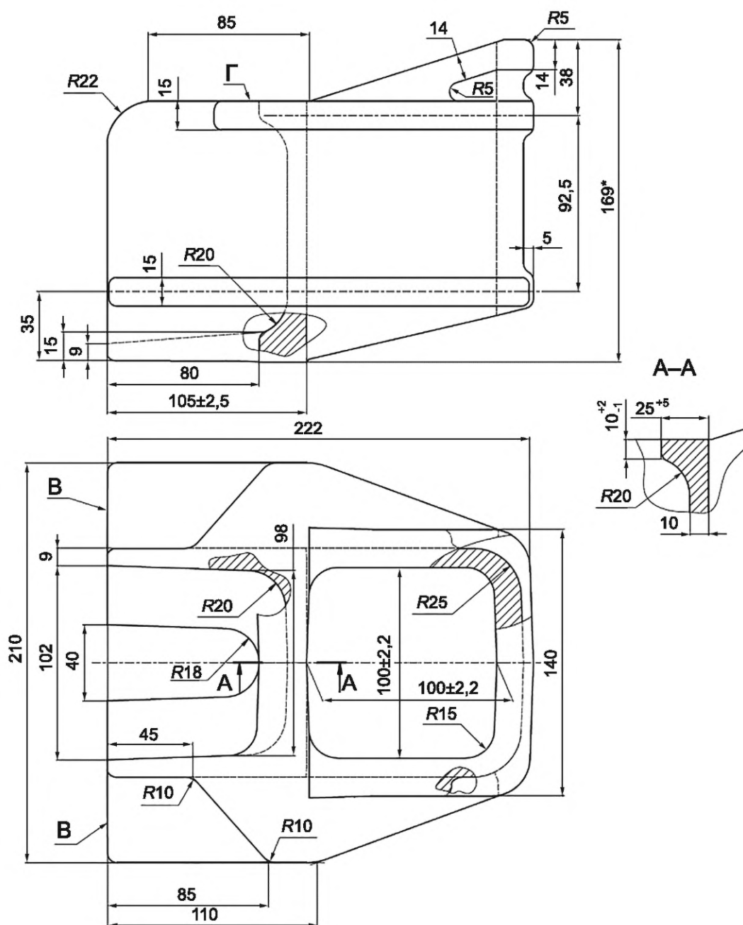
Рисунок 4 — Стоечная скоба типа III исполнения -03
