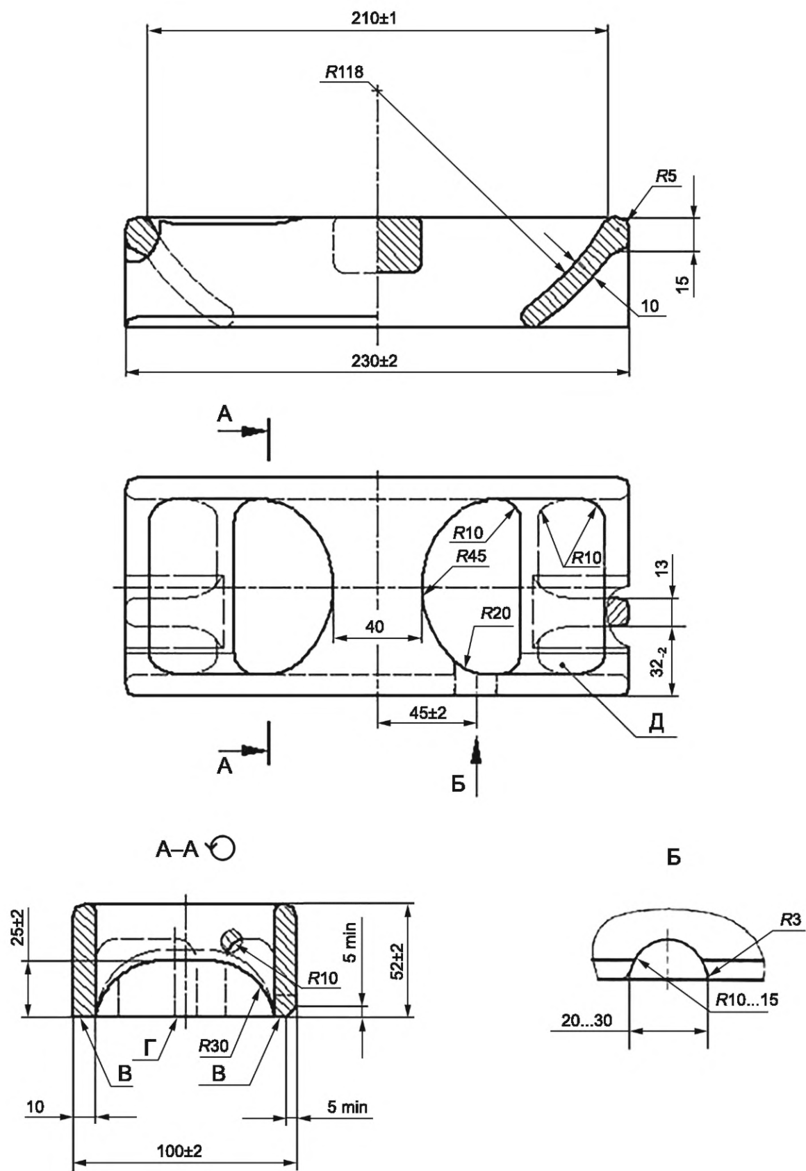
Рисунок 11 — Увзачная скоба типа III исполнения -02
