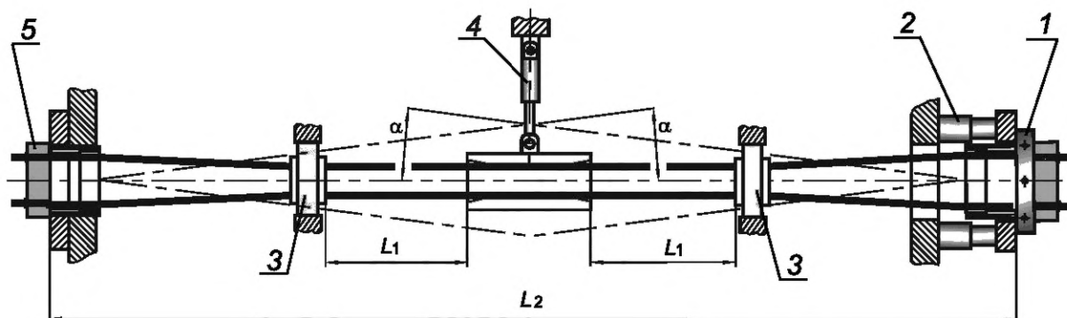
1 — регулируемый вантовый анкер; 2 — привод осевого перемещения; 3 — фиксированный девиатор; 4 — привод поперечного перемещения; 5 — нерегулируемый вантовый анкер; \alpha — см. пункт Б.5; L_1 \geq 0,5 м; L_2 \geq 3,5 м
