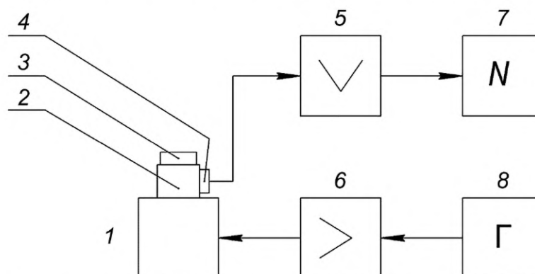
1 — вибрационный стенд; 2 — приспособление для испытаний; 3 — испытуемое изделие; 4 — пьезоэлектрический преобразователь; 5 — селективный микровольтметр; 6 — усилитель мощности; 7 — осциллограф; 8 — задающий генератор
