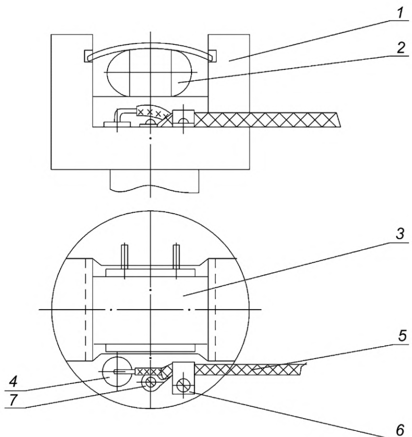
Рисунок А.1 — Конструкция приспособления и крепления изделия
