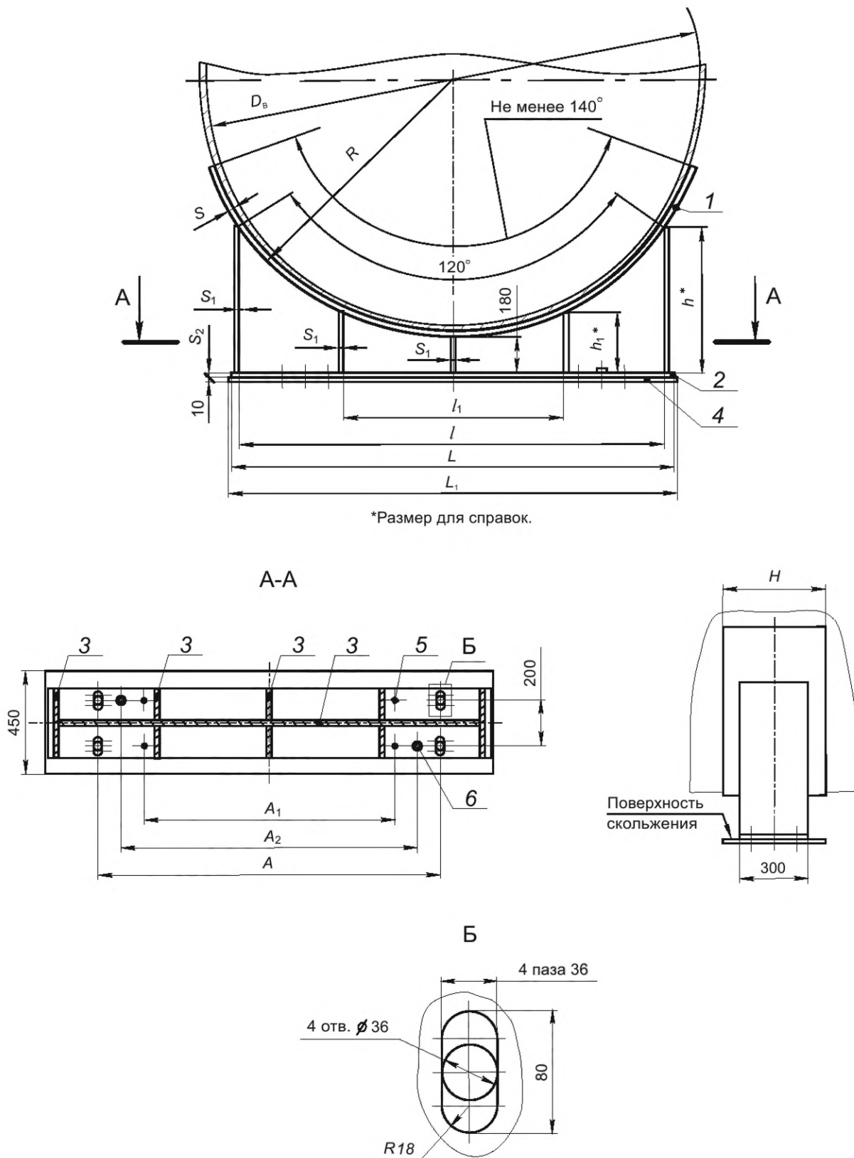
Рисунок 5 — Конструкция подвижной опоры типа 3
