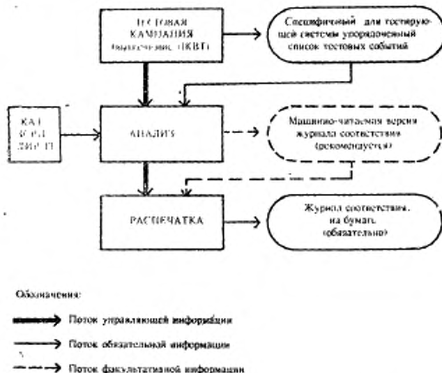
Рисунок А.2 — Создание журнала соответствия
