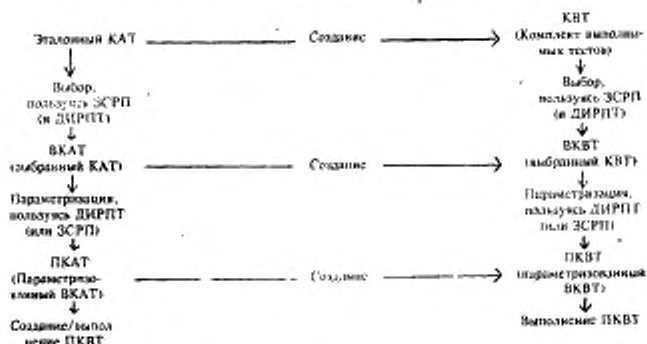
Рисунок А.1 Процесс создания/выполнения ПКВТ
