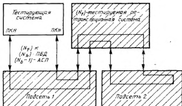
Рисунок 13 — Метод шлейфового тестирования (МШТ)
