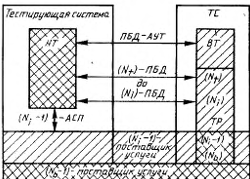
Рисунок 11 — Пример метода COBT: тестирование (N_i) -протокола в (N_b) до (N_i) -протоколе ТР
