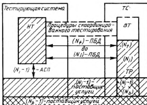
Рисунок 12 — Пример метода УОВТ: тестирование (N_1) -протокола в (N_2) до (N_c) -протоколе TP
