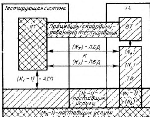
Рисунок 10 — Пример метода ROBT: тестирование (N_i) -протокола в (N_b) до (N_i) -протоколе ТР
