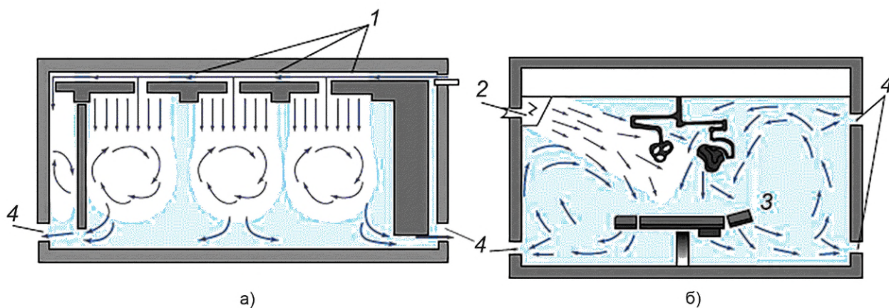
1 — потолочный воздухоораспределитель; 2 — настенный воздухоораспределитель, совмещенный с высокоэффективным фильтром очистки класса Н; 3 — технологическое оборудование (операционный стол); 4 — вытяжные сепараторы пуха
