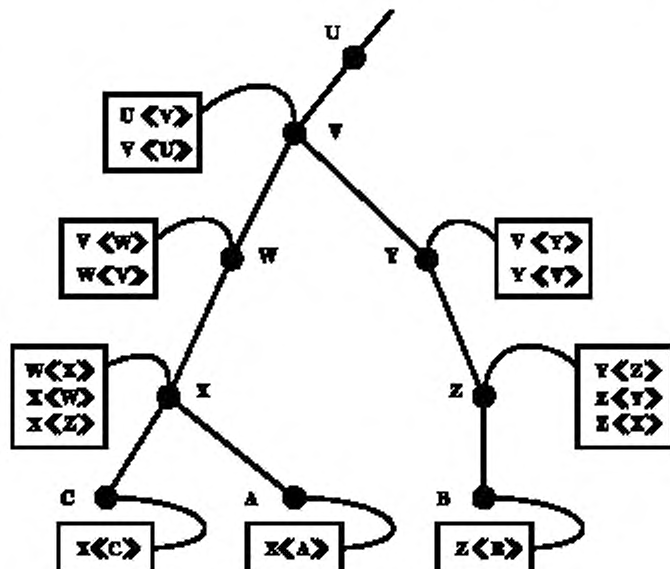
Рисунок 4 — Иерархия. Гипотетический пример
