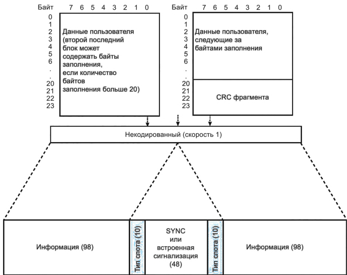
Рисунок 120 — Формат блока данных без подтверждения в режиме «без кодирования» («скорость кодирования 1»)
