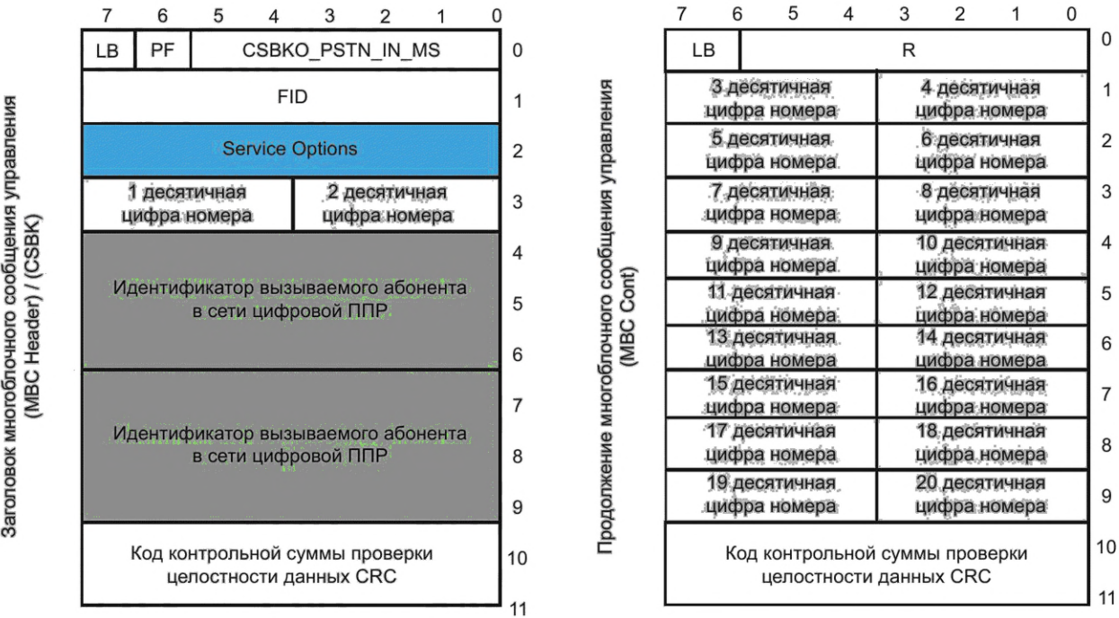
Рисунок А.3 — Пакет входящего вызова от шлюза ССОП на АС
