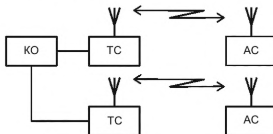
Рисунок 10 — Структурная схема организации сети ППР настоящего комплекса стандартов с использованием режима транкинга
