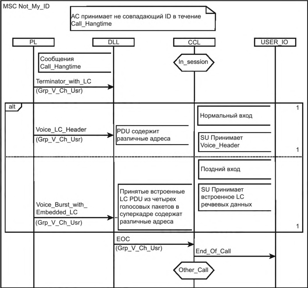
Рисунок 101 — MSC для Not_My_ID
