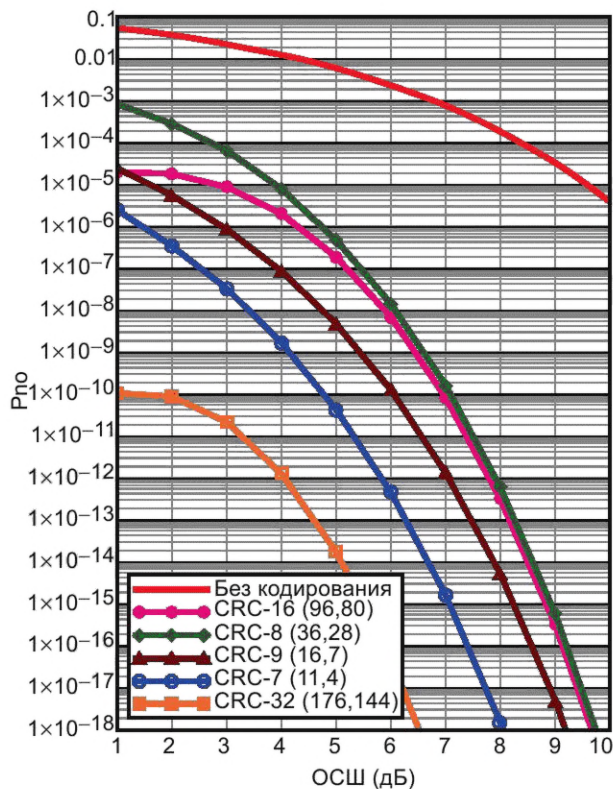
в) Графики вероятности необнаружения искажения в пакете для CRC-кодов (постоянная скорость передачи информации)
