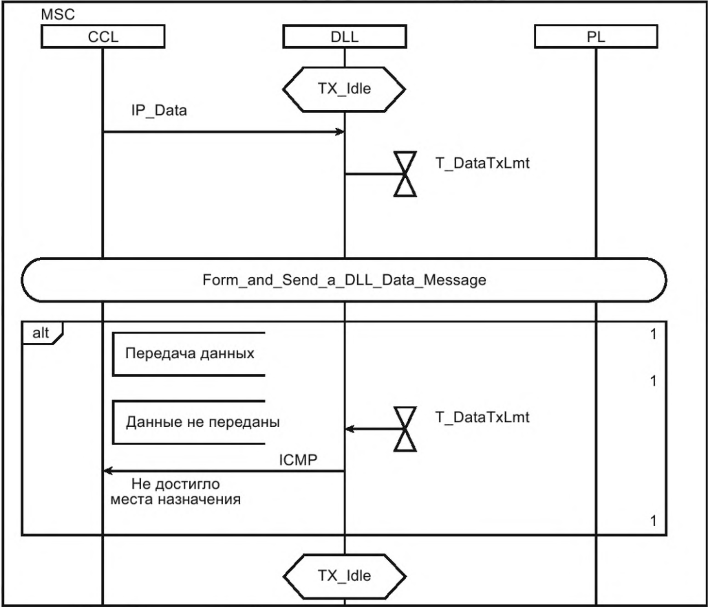
Рисунок 43 — MSC передачи неподтверждаемых IP-данных
