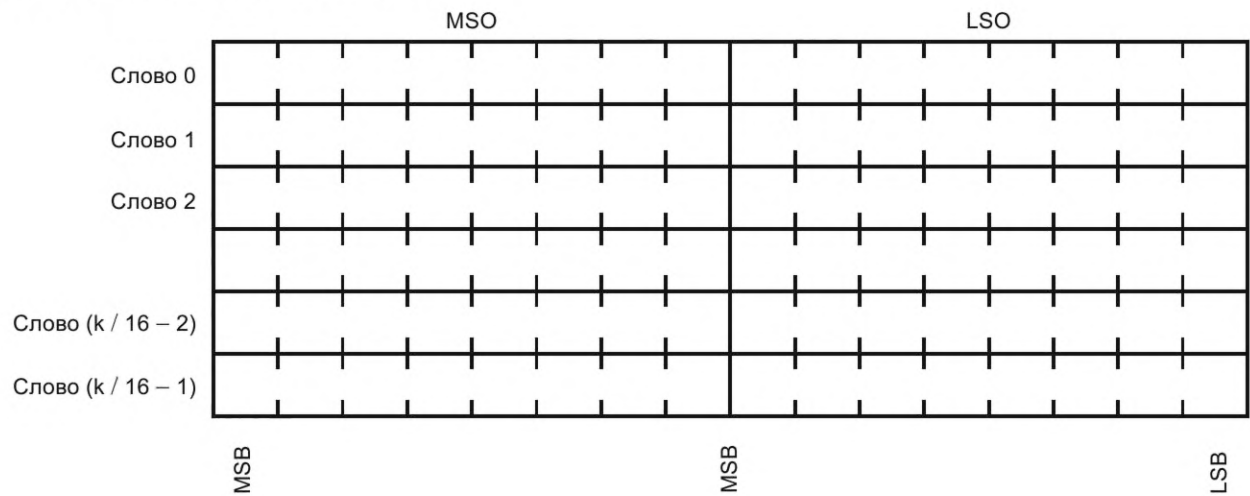
Рисунок Б.9 — Пользовательские данные и байты заполнения в виде слов по 16 бит
