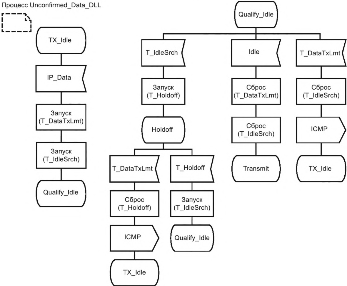
Рисунок 42 — SDL-диаграмма доступа к каналу при передаче неподтверждаемых IP-данных
