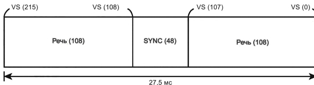
Рисунок 56 — Речевой пакет с синхронизацией
