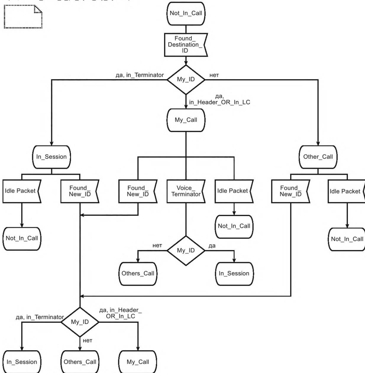
Рисунок Е.3 — SDL-диаграмма АС уровня 2
