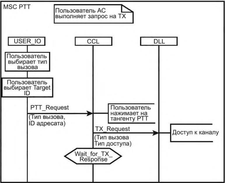
Рисунок 93 — MSC для PTT
