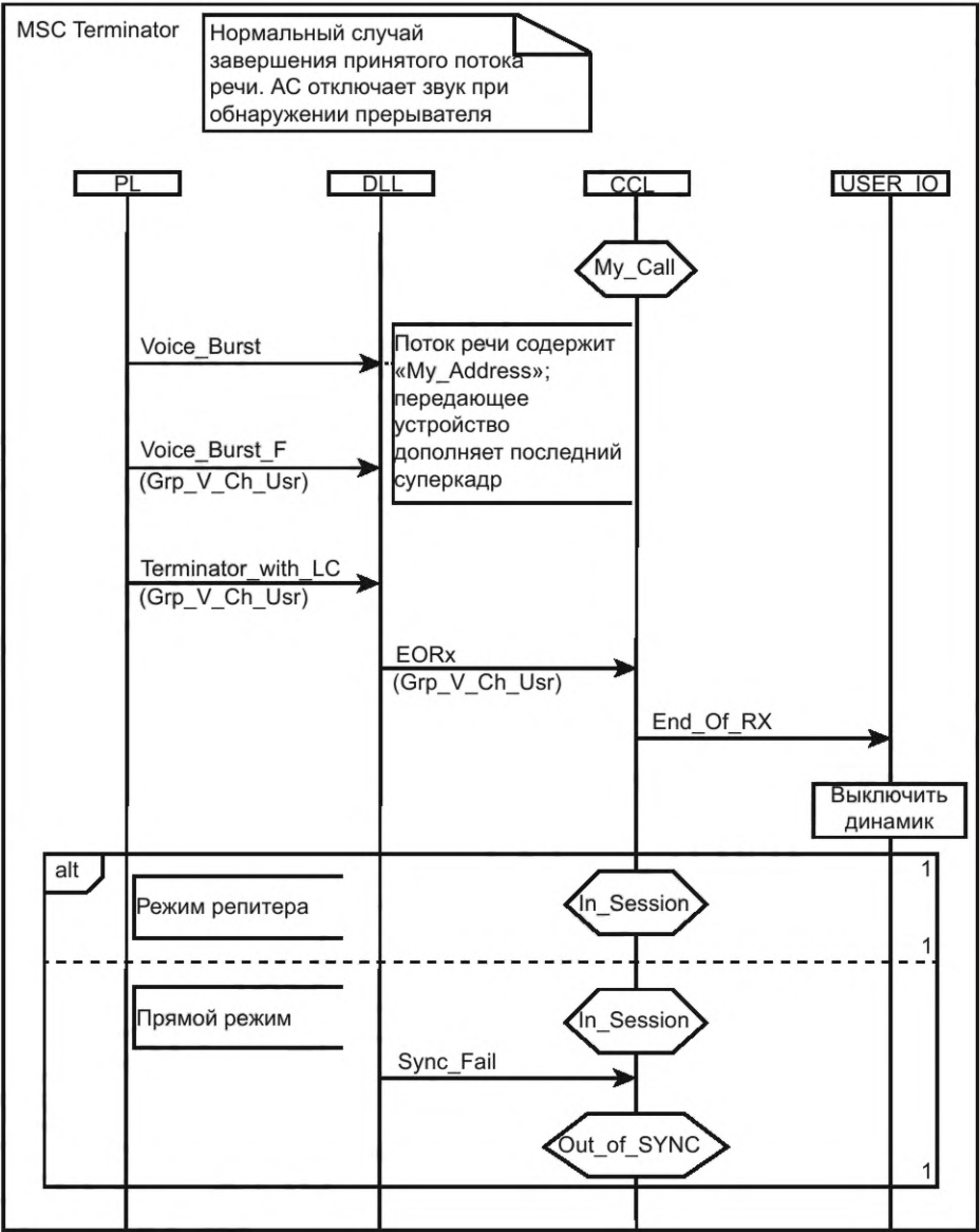
Рисунок 99 — MSC для прерывателя
