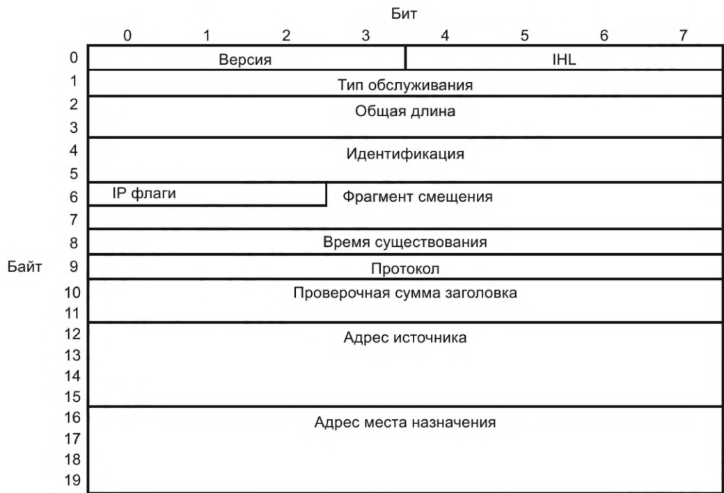
Рисунок 51 — Заголовок IPv4
