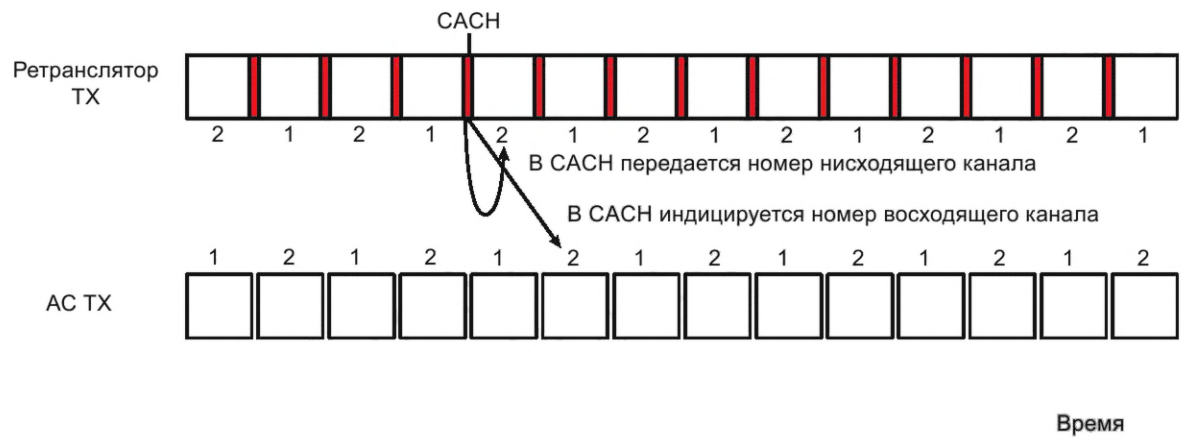
Рисунок 9 — Передача указателя о номере таймслота доступного канала
