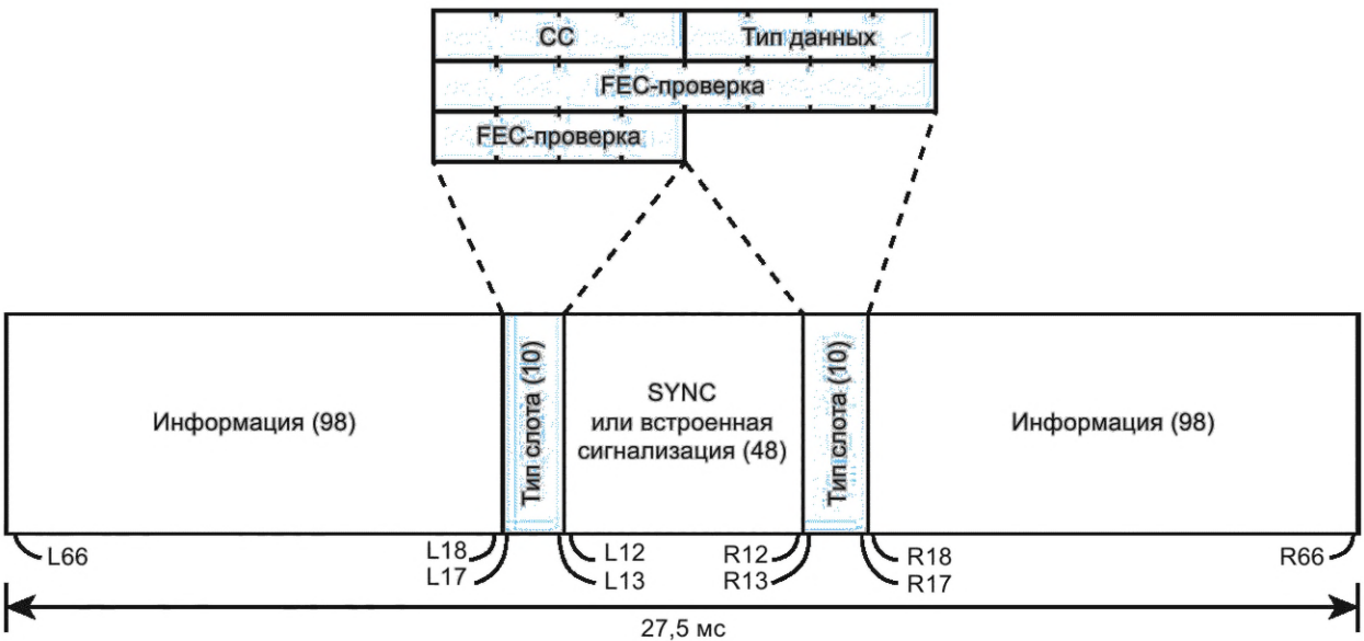
Рисунок 58 — Структура пакета данных (управления)
