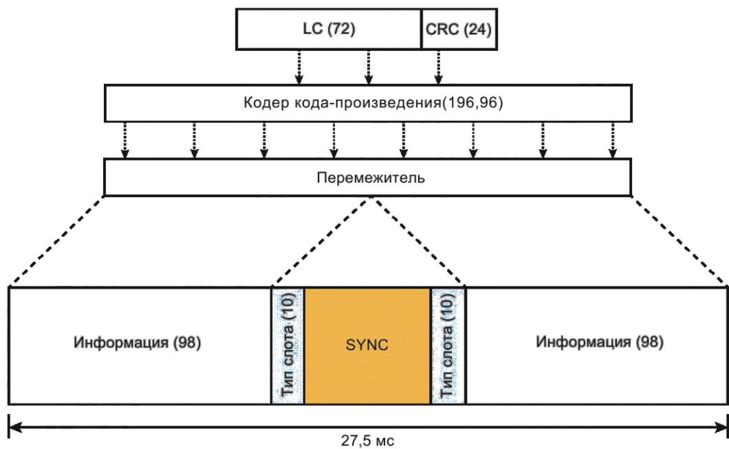
Рисунок 64 — Формирование прерывателя с LC
