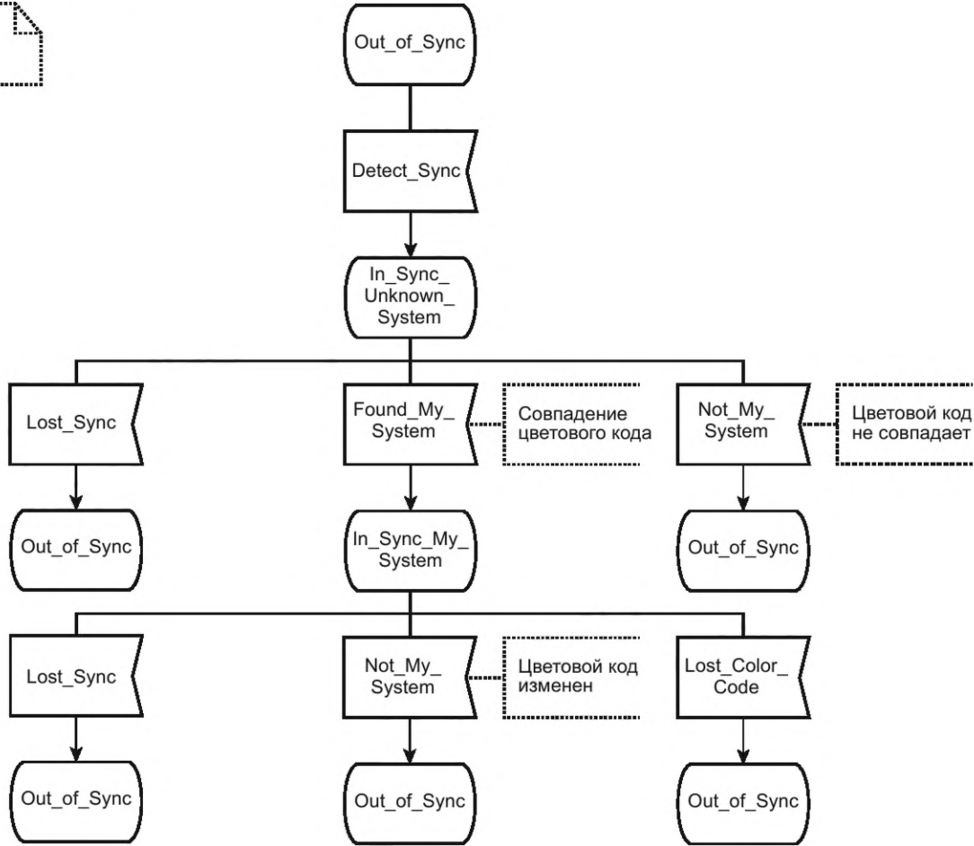
Рисунок Е.1 — SDL-диаграмма АС уровня 1, прямой режим
