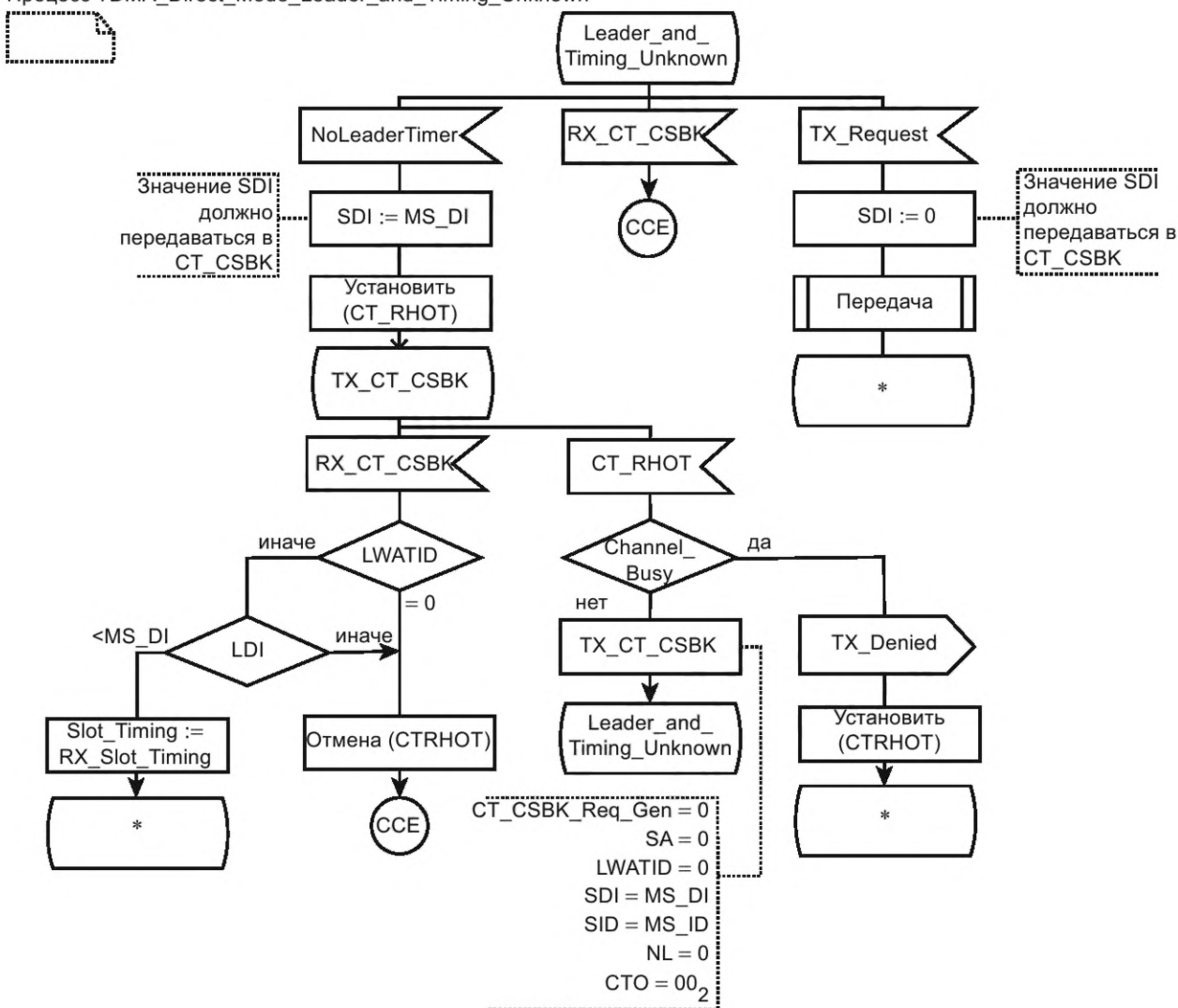
Рисунок 79 — SDL для состояния Leader_and_Timing_Unknown
