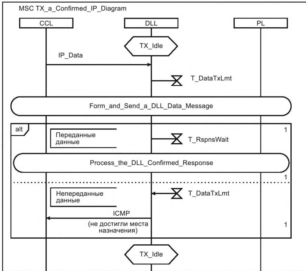
Рисунок 47 — MSC передачи подтверждаемых IP-данных
