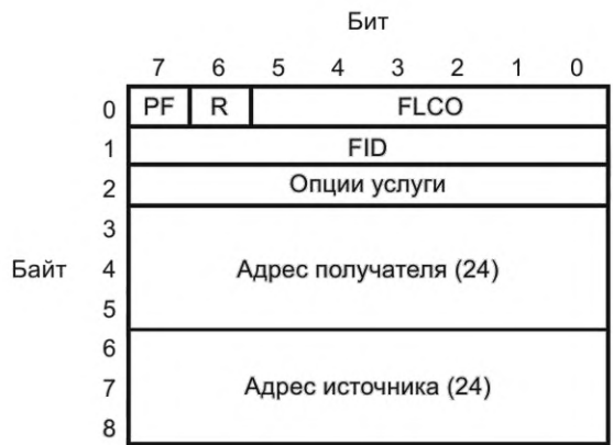
Рисунок 60 — Структура заголовка Full LC для индивидуального вызова
