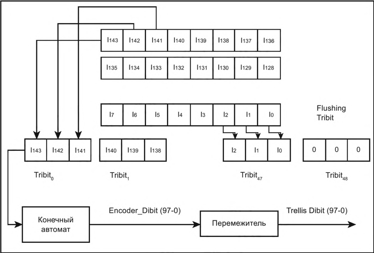
Рисунок Б.8 — Процедура кодирования треллис-кодом 3/4
