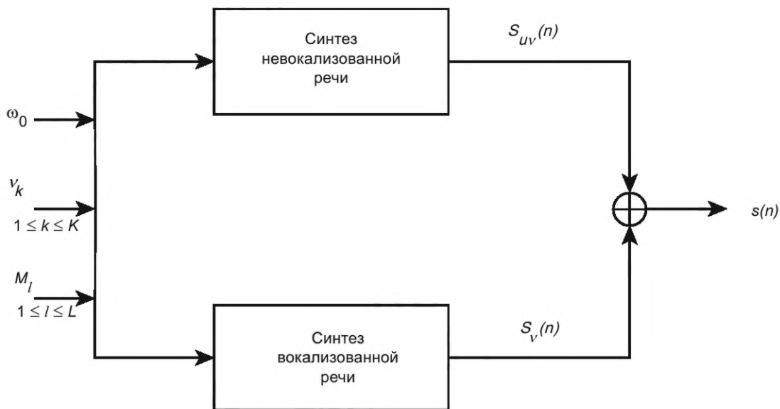
Рисунок К.9 — Синтез речи
