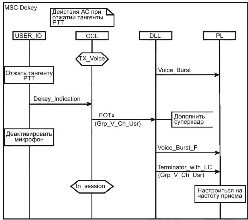
Рисунок 98 — MSC для состояния, когда тангента РТТ отжата
