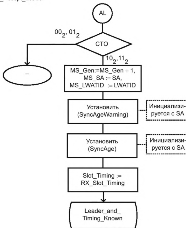
Рисунок 86 — SDL для процедуры AL
