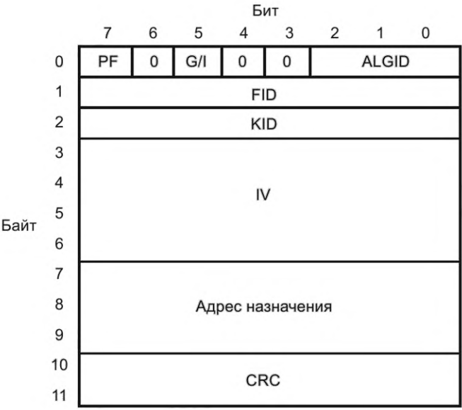
Рисунок 61 — Структура заголовка PI PDU
