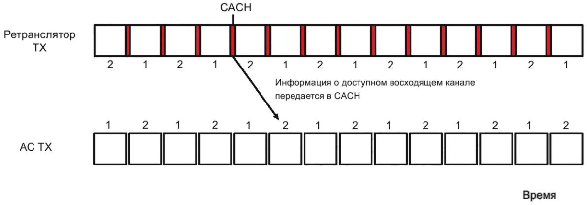
Рисунок 8 — Передача указателя о доступном восходящем канале
