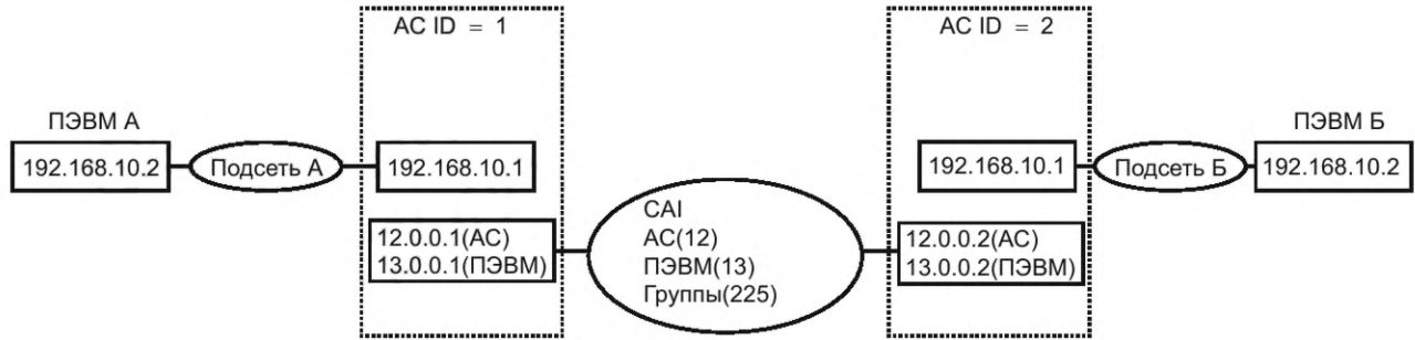
Рисунок А.8 — Пример IP-радиосети с NAT-преобразованиями локальных адресов периферийных устройств
