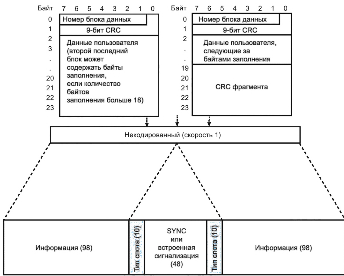
Рисунок 123 — Формат блока данных с подтверждением для схемы без кодирования
