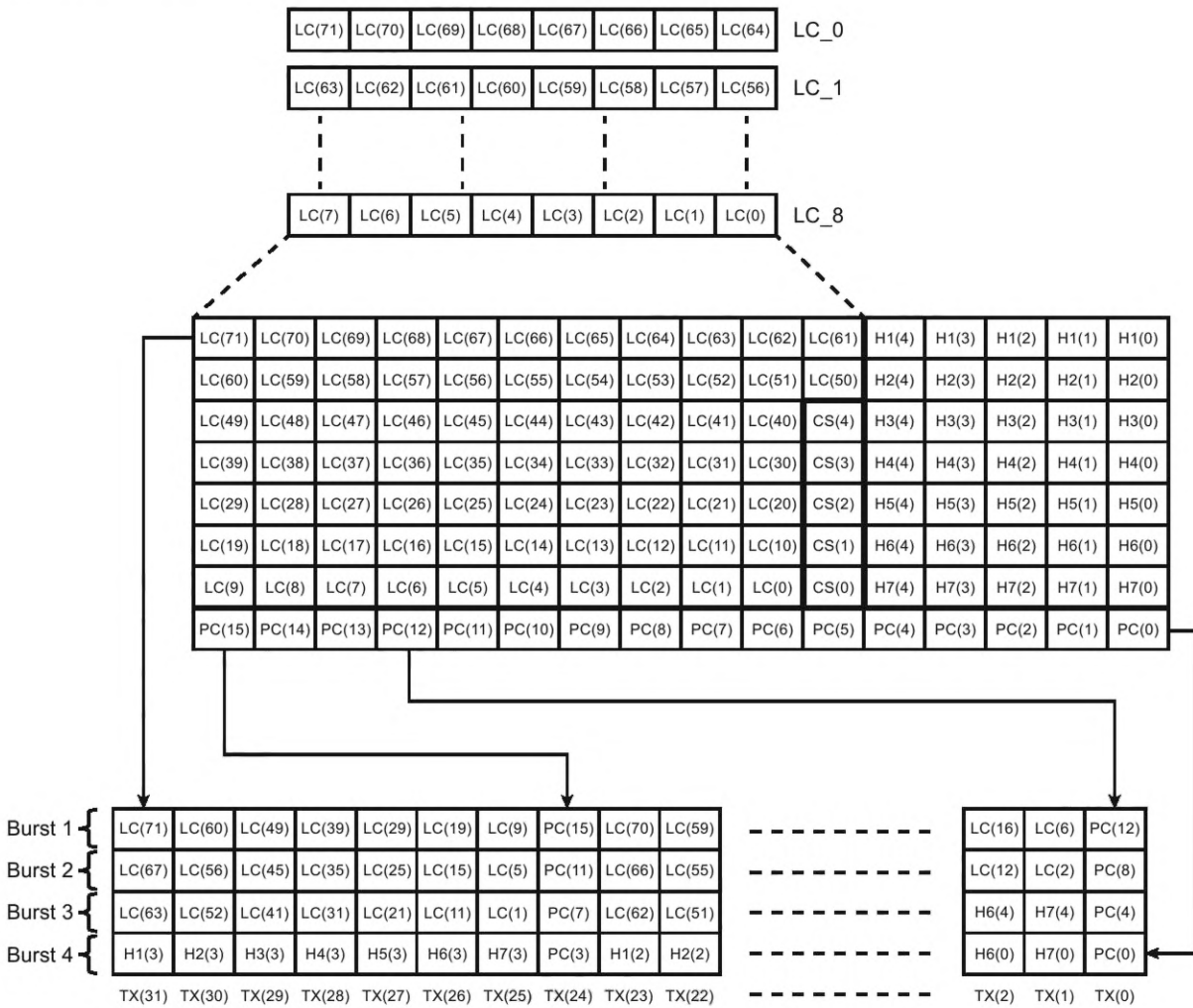
Рисунок Б.3 — Структура пакетов встроенной сигнализации
