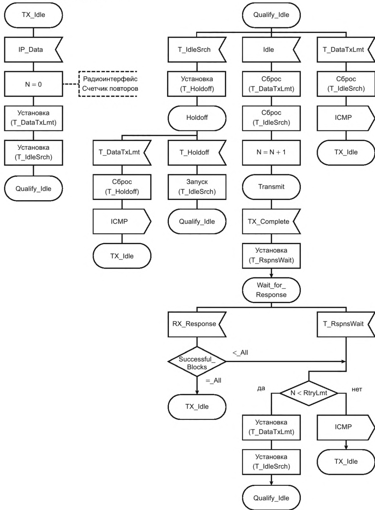
Рисунок 45 — SDL-диаграмма передачи подтверждаемых данных источником
