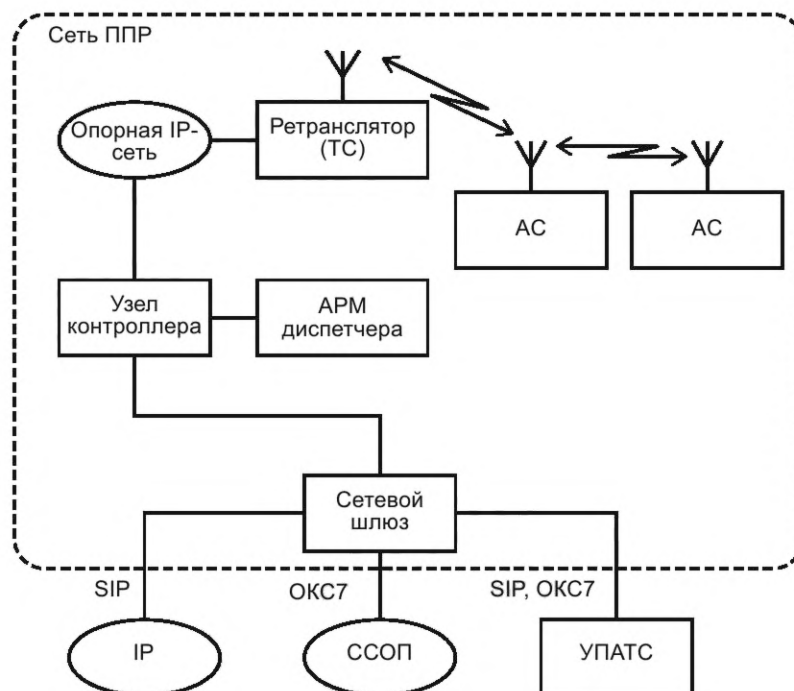
Рисунок 12 — Пример схемы организации сети ППР и ее присоединения к ССОП, УПАТС и IP-сетям
