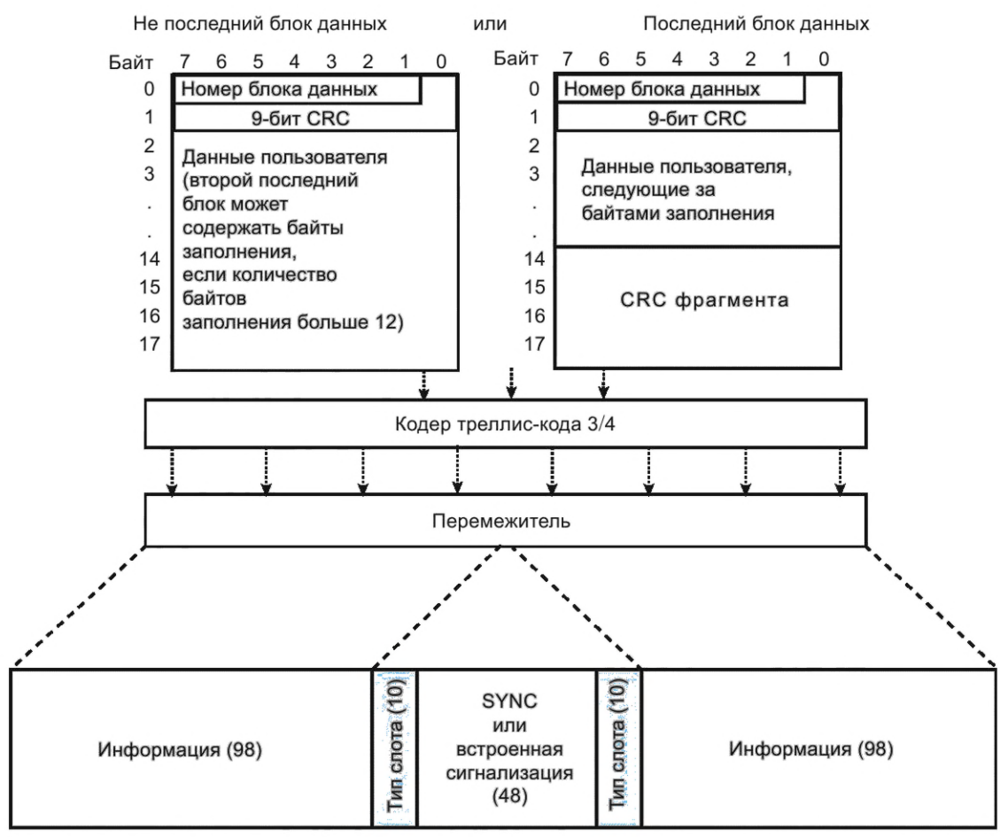
Рисунок 121 — Формат блока данных с подтверждением достоверности и треллис-кодом со скоростью кодирования 3/4
