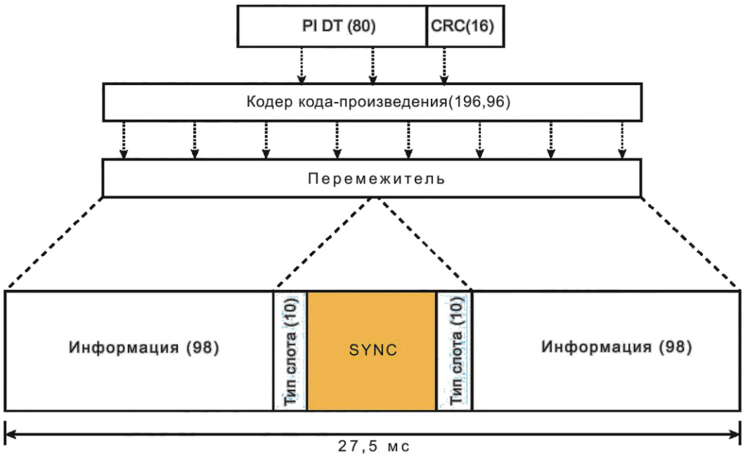
Рисунок 67 — Формирование заголовка передачи шифрованных данных
