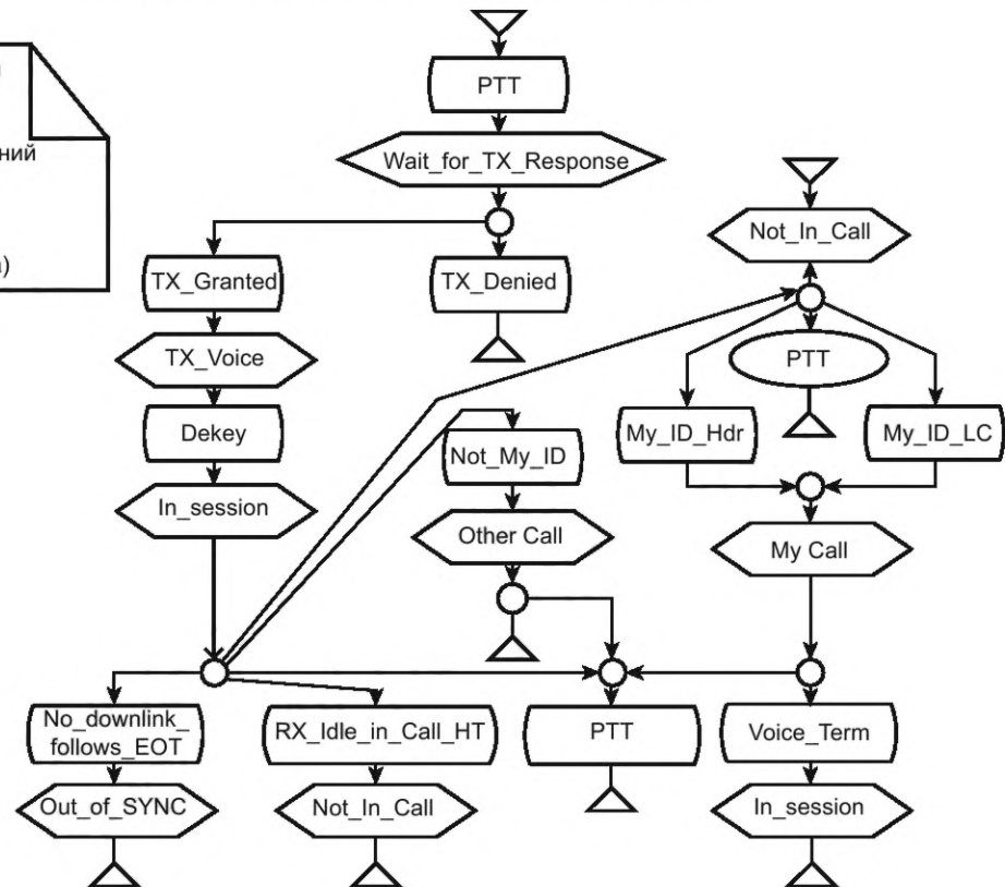
Рисунок 92 — HMSC для передачи группового вызова
