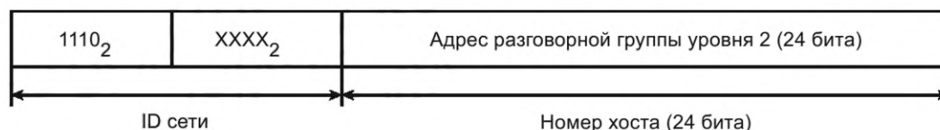
Рисунок 41 — Формат адреса класса D
