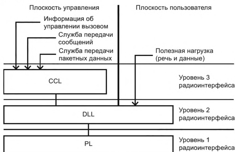
Рисунок 18 — Стек протоколов настоящего комплекса стандартов
