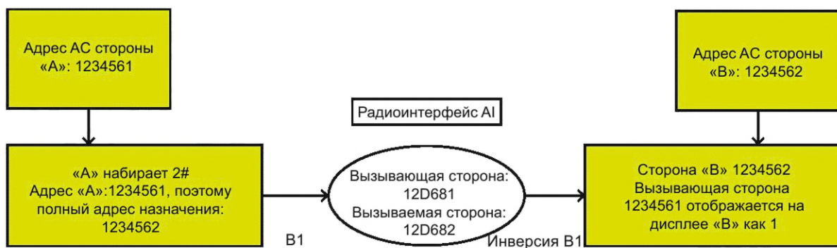
Рисунок А.15 — Пример сокращенного набора
