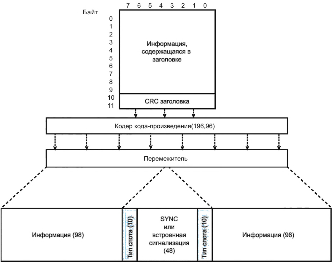
Рисунок 109 — Структура общего первого блока заголовка
