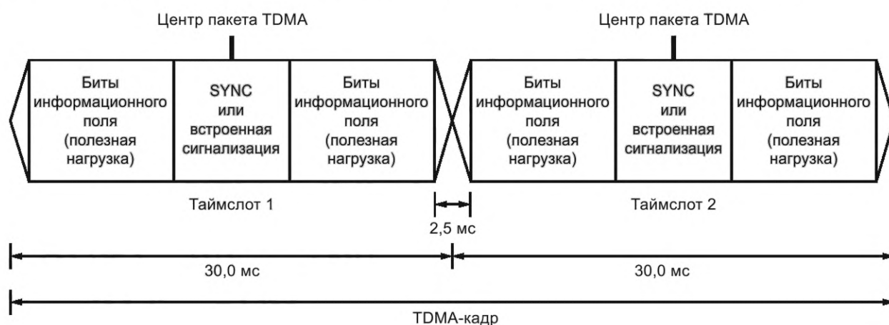
Рисунок 21 — Временная диаграмма расположения TDMA-пакетов
