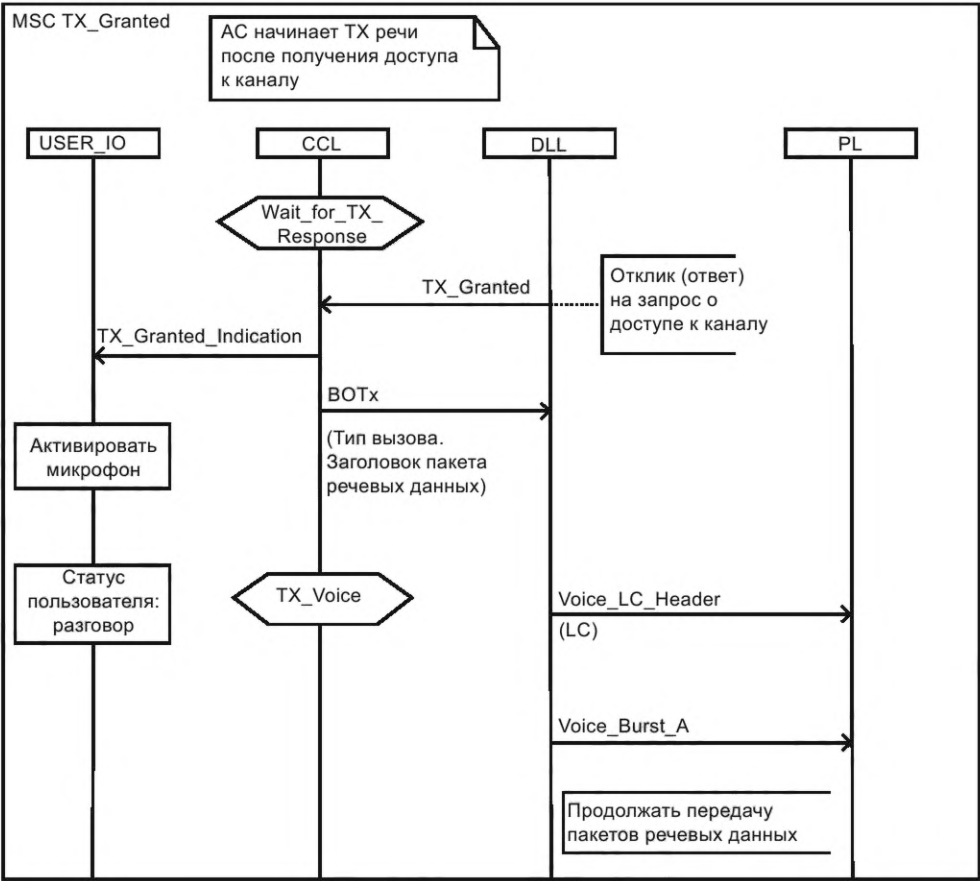
Рисунок 95 — MSC для TX_Granted
