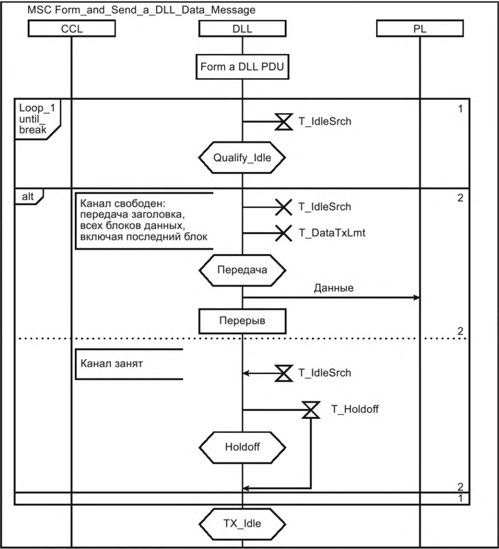
Рисунок 44 — MSC формирования и отправления DLL-сообщений данных
