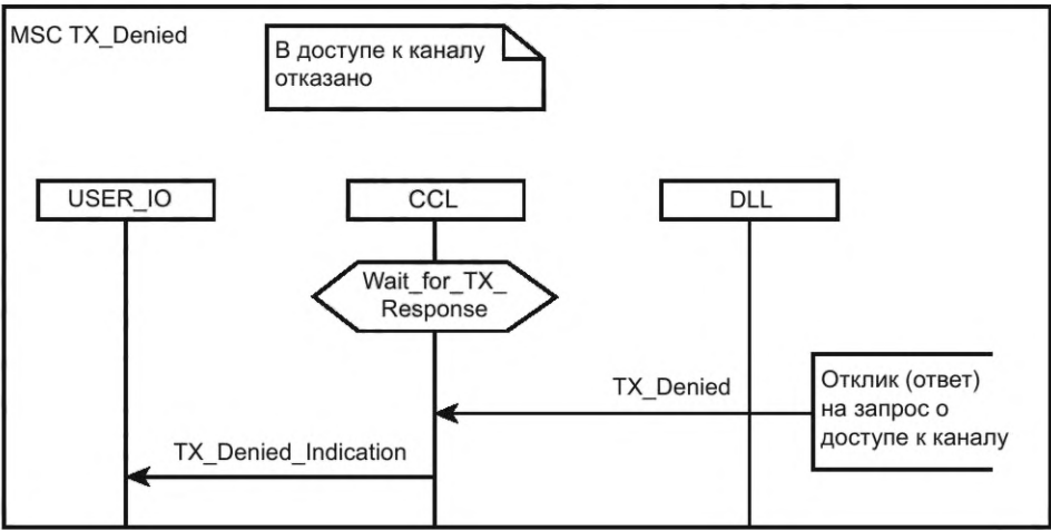
Рисунок 94 — MSC для TX_Denied
