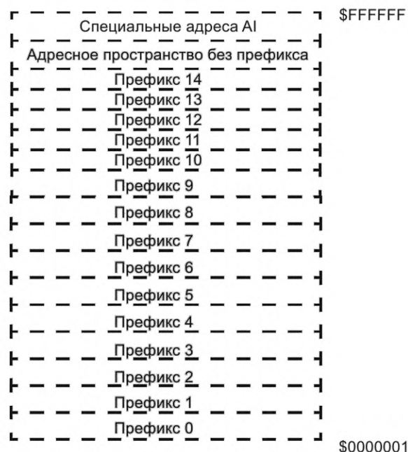
Рисунок А.14 — Разделение адресного пространства при помощи префикса
