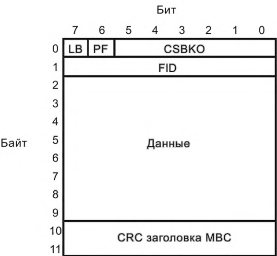
Рисунок 71 — Структура заголовка MBC
