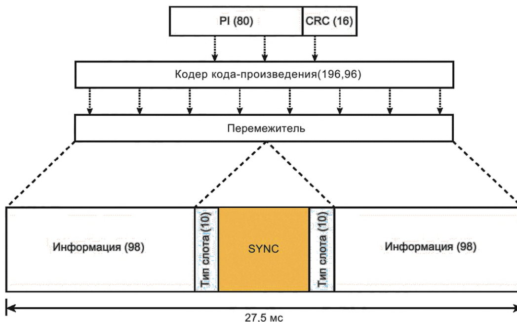
Рисунок 63 — Формирование PI-заголовка передачи шифрованной речи
