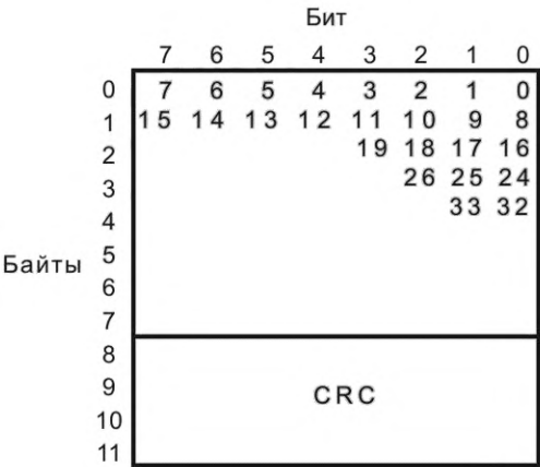
Рисунок 124 — Блок данных ответного пакета
