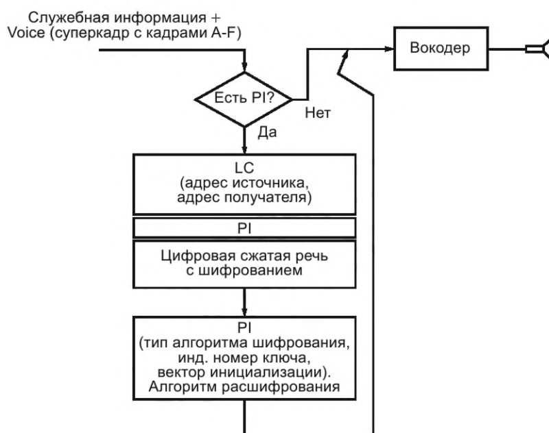
Рисунок 16 — Структурная схема расшифрования речевого сообщения в АС
