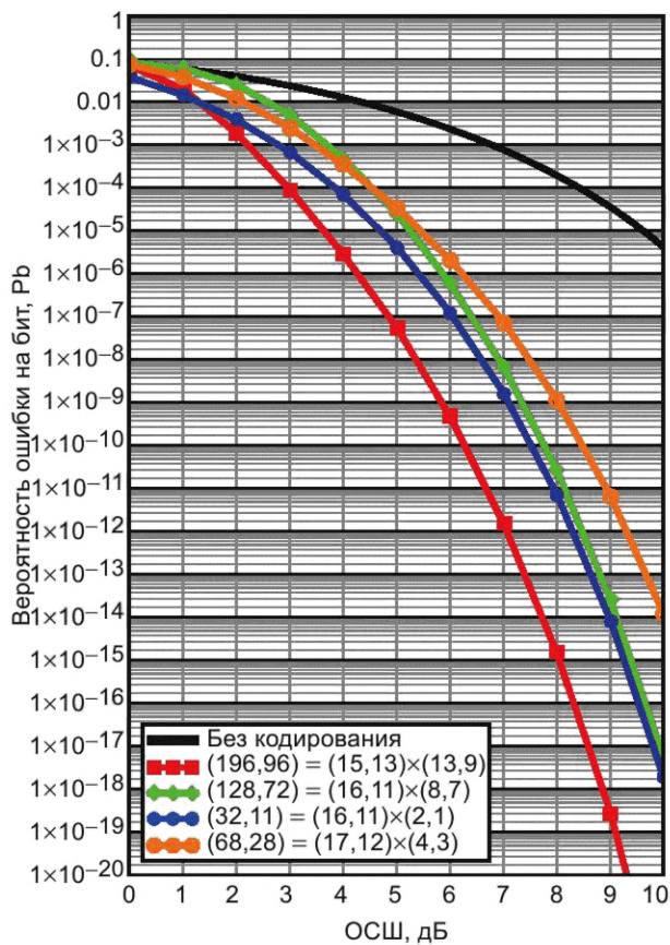
а) Графики вероятности ошибки кодов-произведений. Потенциальные границы ВРТС, постоянная скорость
