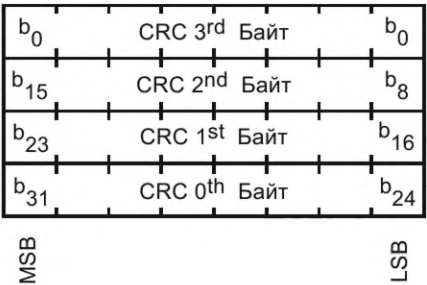
Рисунок Б.11 — Порядок размещения проверочных битов CRC-32 по байтам
