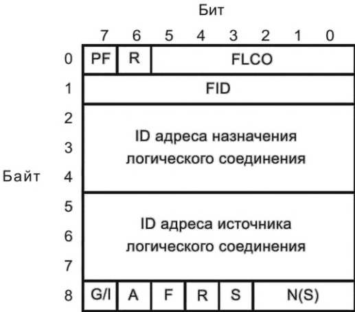
Рисунок 125 — Структура TD_LC PDU
