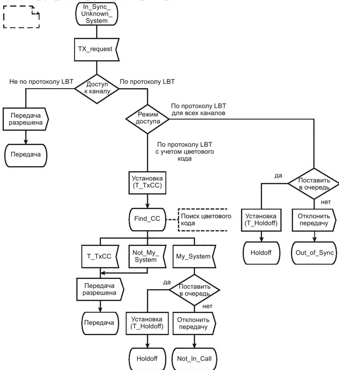
Рисунок 35 — SDL-диаграмма In_Sync_Unknown_System
