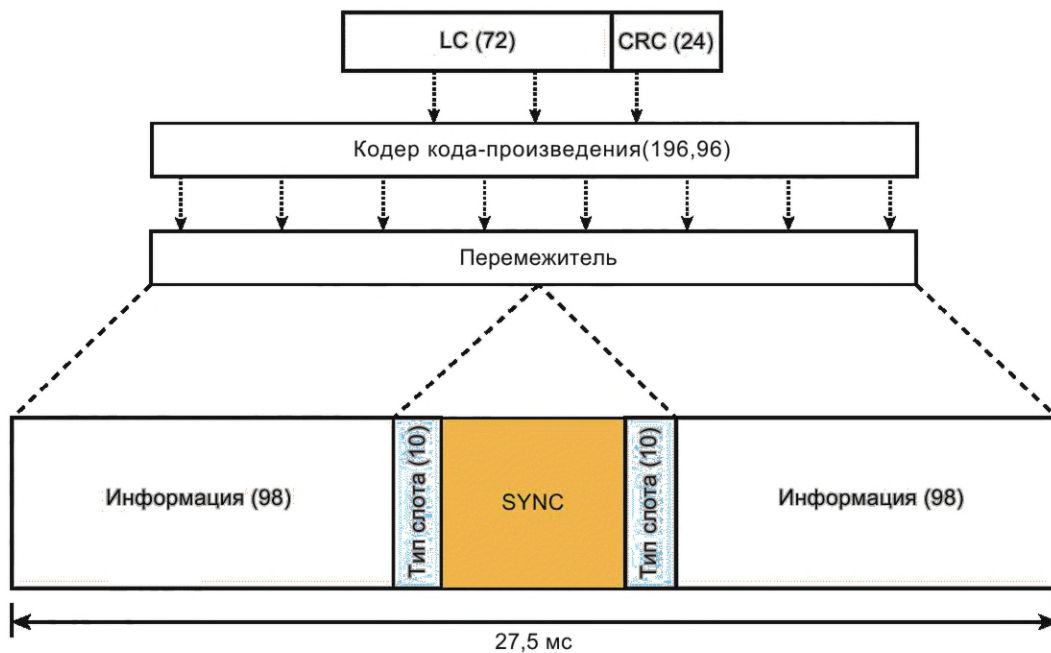
Рисунок 62 — Формирование речевого LC-заголовка
