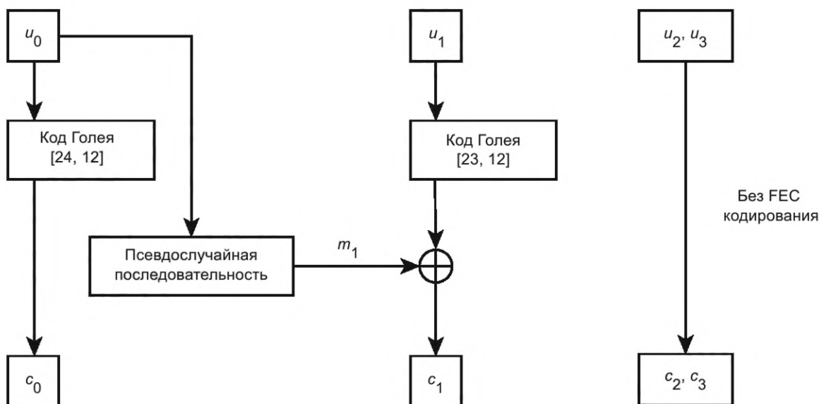
Рисунок К.10 — Построение кодовых слов
