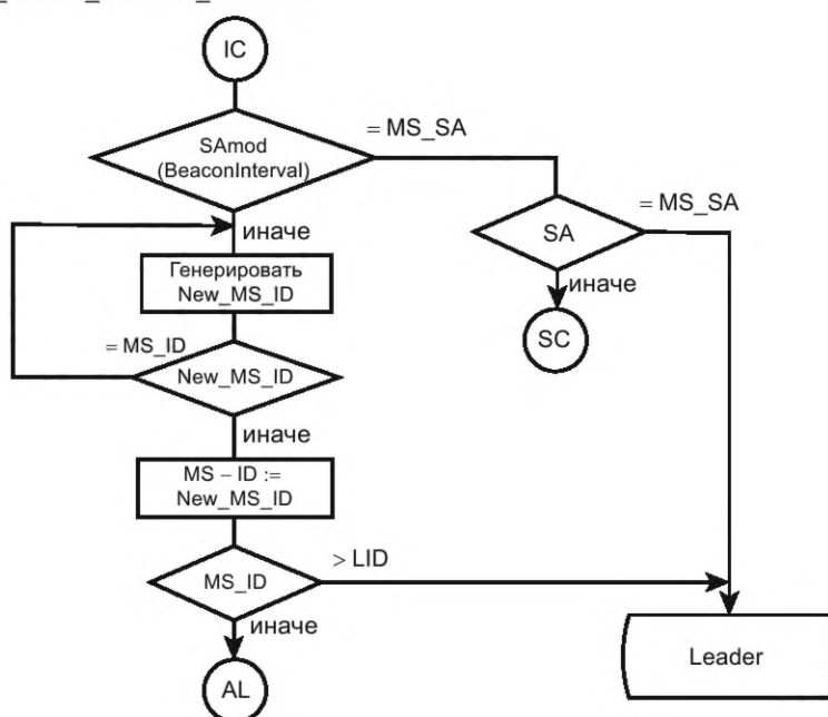
Рисунок 83 — SDL процедуры IC
