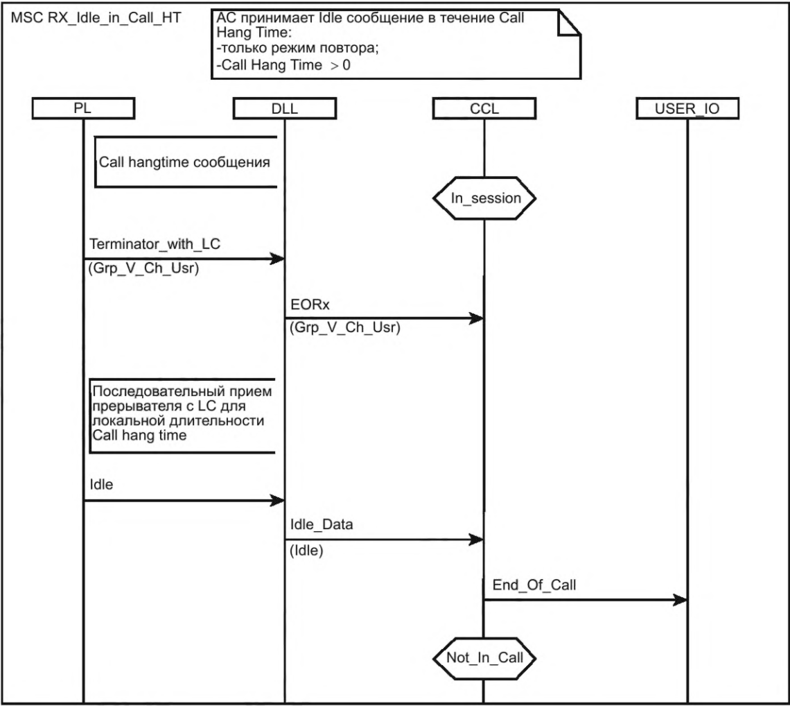
Рисунок 100 — MSC для RX_Idle_SYNC_in_Call_HT
