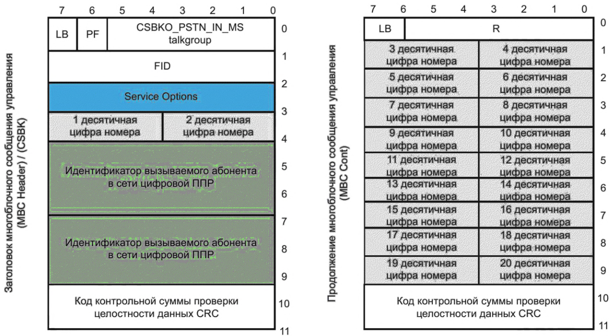
Рисунок А.5 — Пакет входящего вызова от шлюза ССОП на разговорную группу АС
