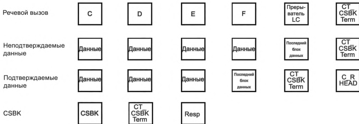
Рисунок 77 — Прерывание с использованием CT_CSBK_Term
