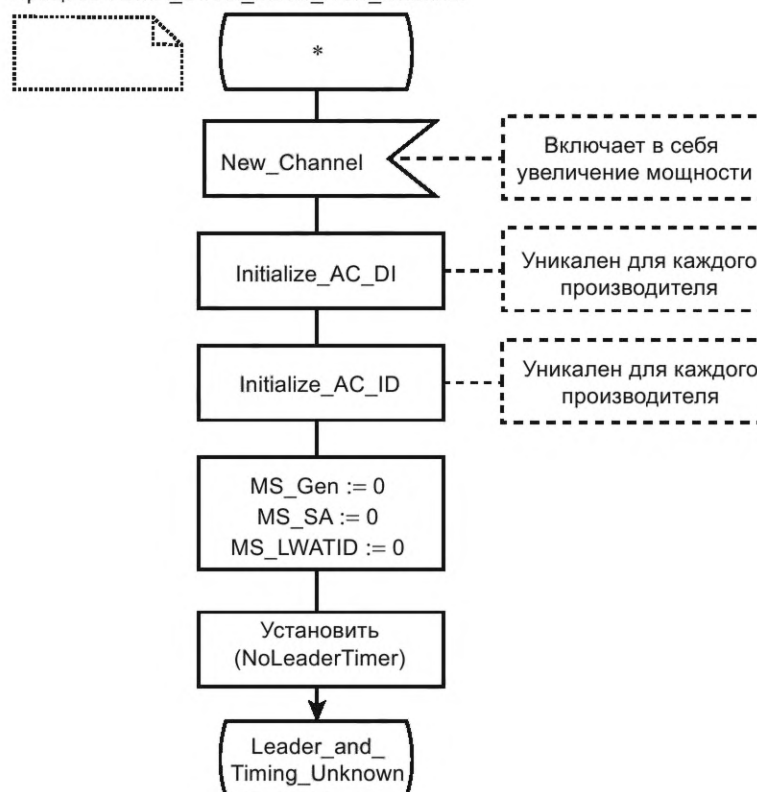
Рисунок 78 — SDL повышения мощности и смены канала
