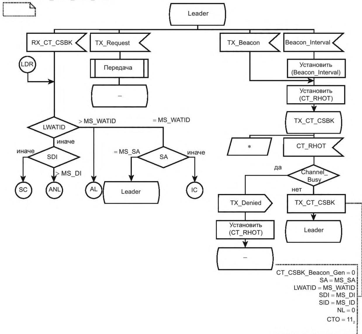
Рисунок 82 — SDL для состояния Leader
