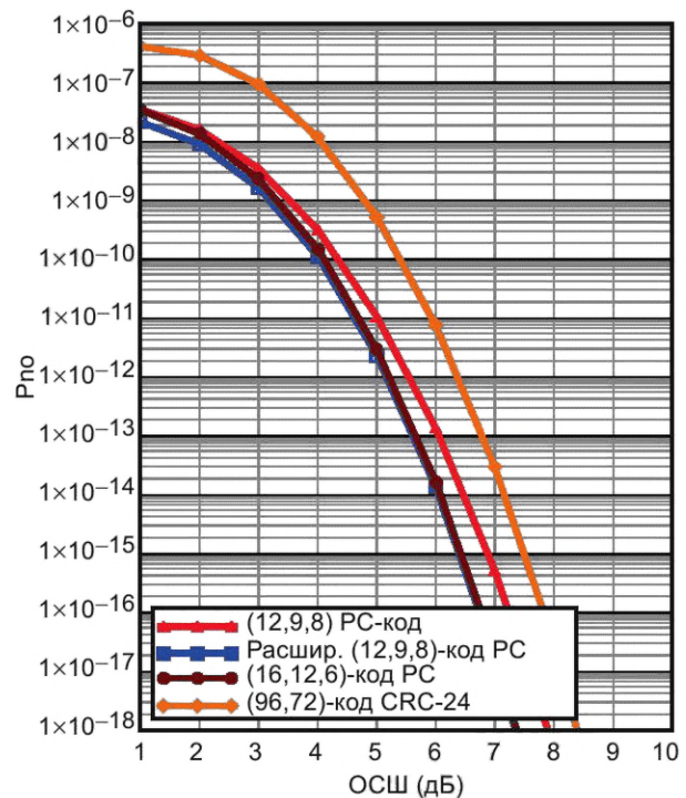
г) Графики вероятности необнаружения искажения в пакете для кодов Рида-Соломона (12,9,8) (постоянная скорость передачи информации)
