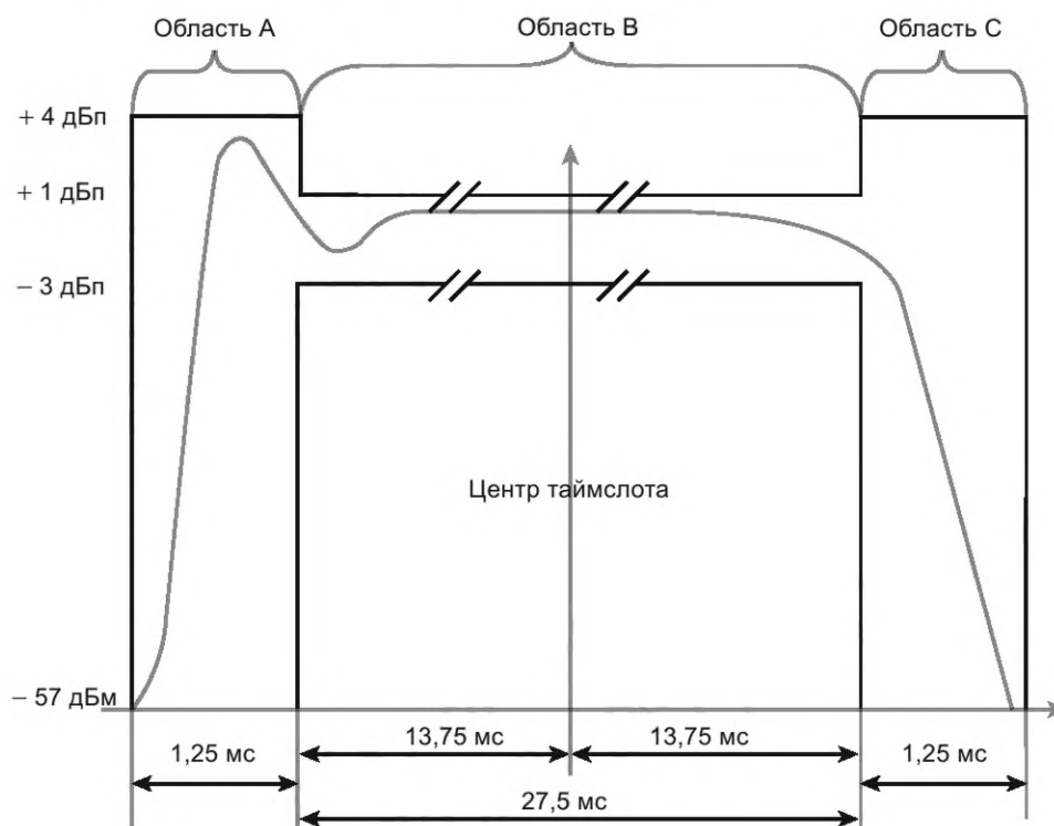
Рисунок 132 — «Маска» мощности огибающей волны передатчика для общего пакета физического уровня
