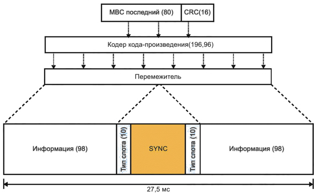
Рисунок 76 — Структура последнего блока MBC
