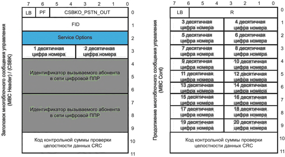
Рисунок А.1 — Пакет инициирования исходящего вызова от АС на шлюз ССОП
