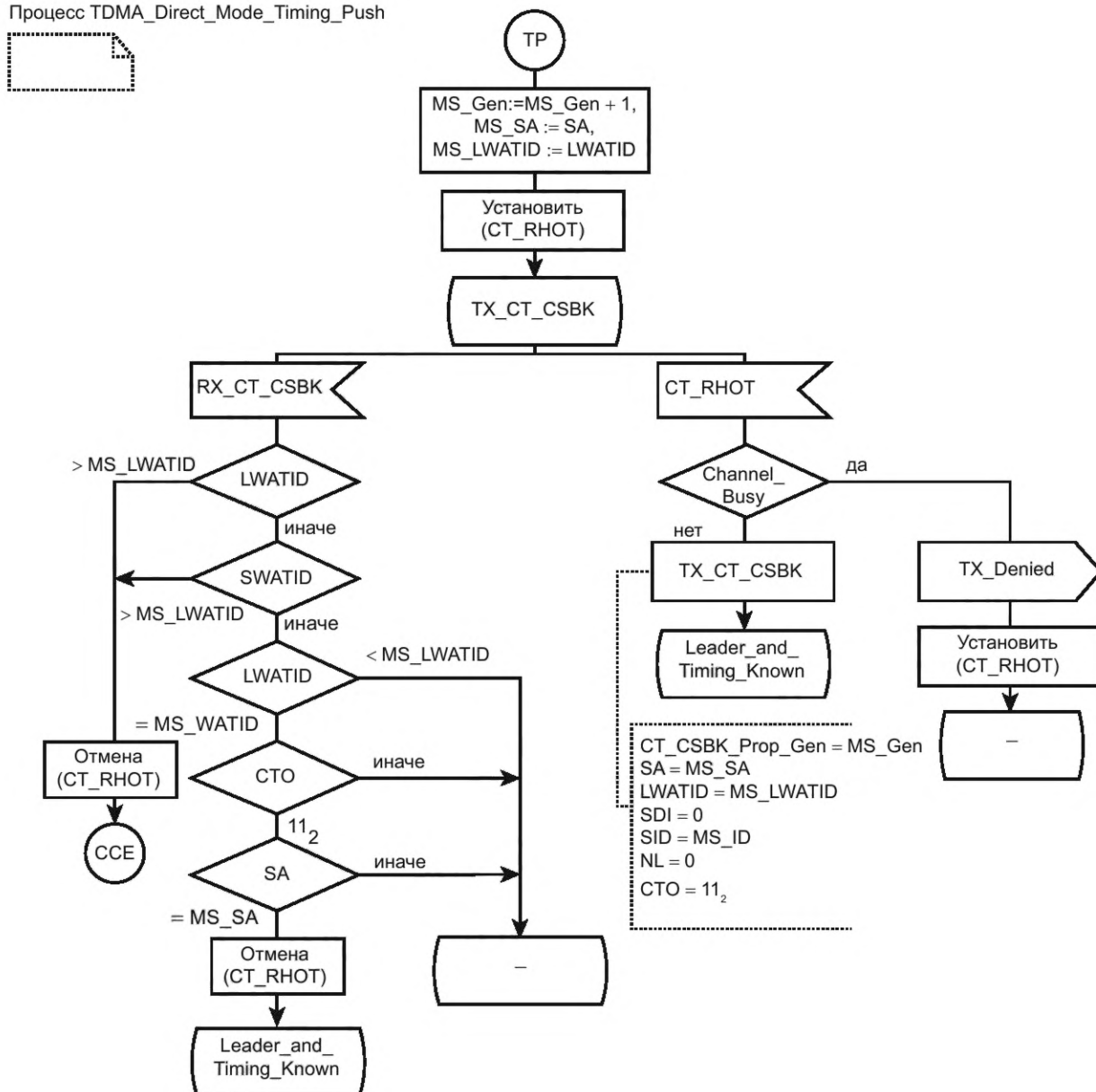
Рисунок 88 — SDL для процедуры TP
