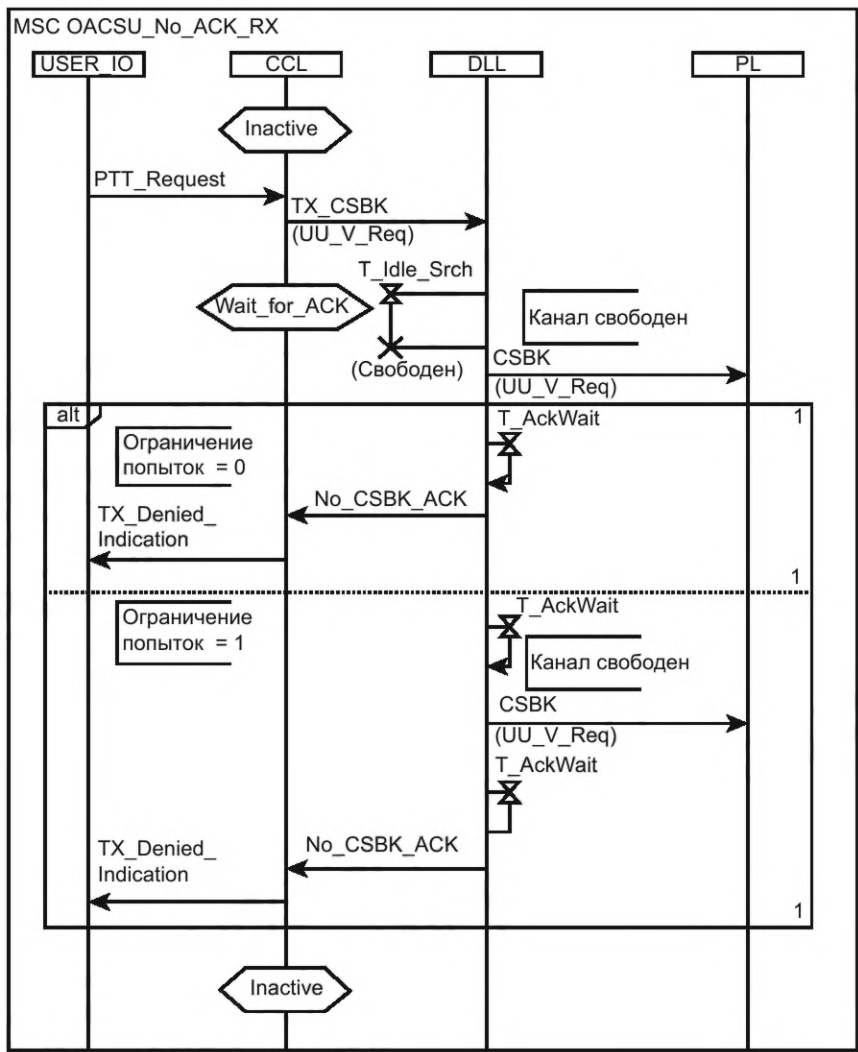
Рисунок 106 — OACSU для индивидуального вызова, когда не получено ACK
