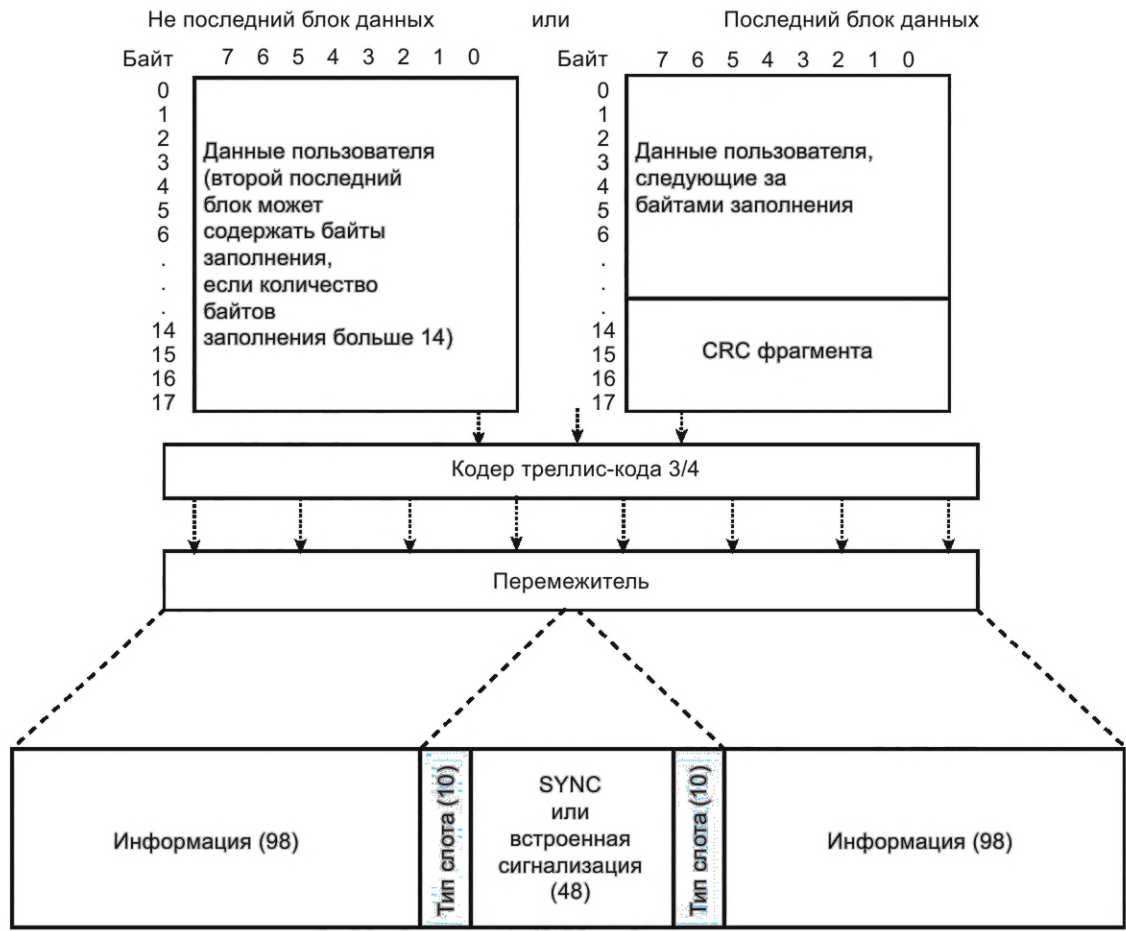
Рисунок 119 — Формат блока данных без подтверждения с FEC со скоростью кодирования ¾
