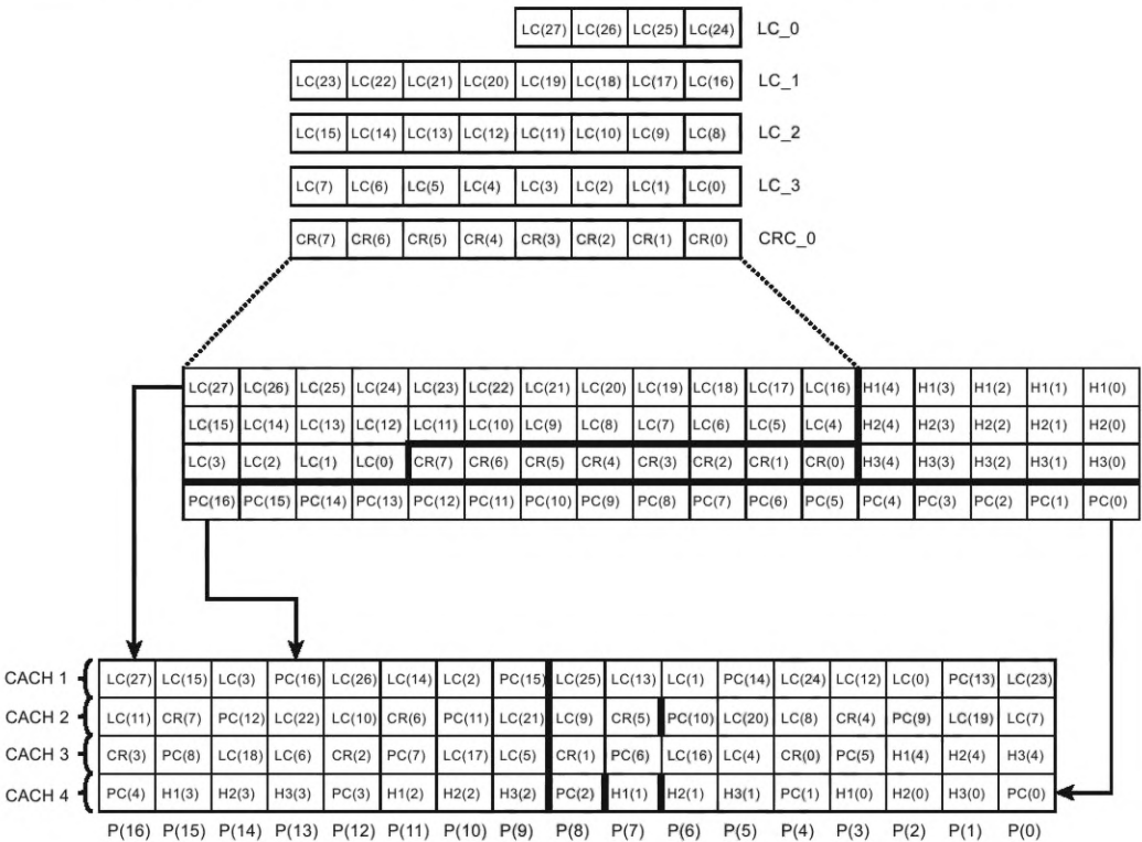
Рисунок Б.7 — Структура пакетов с CACH
