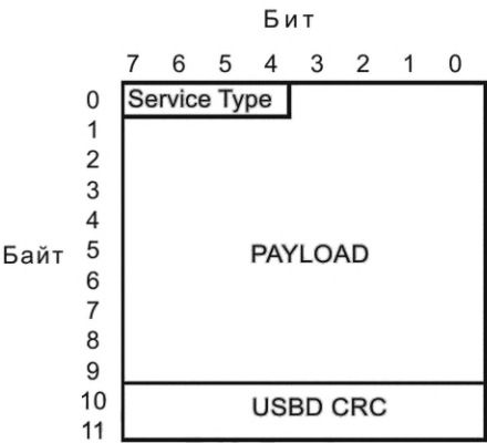
Рисунок 128 — Структура USBД
