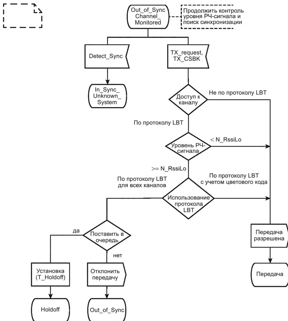
Рисунок 34 — SDL-диаграмма Out_of_Sync_Channel_Monitored
