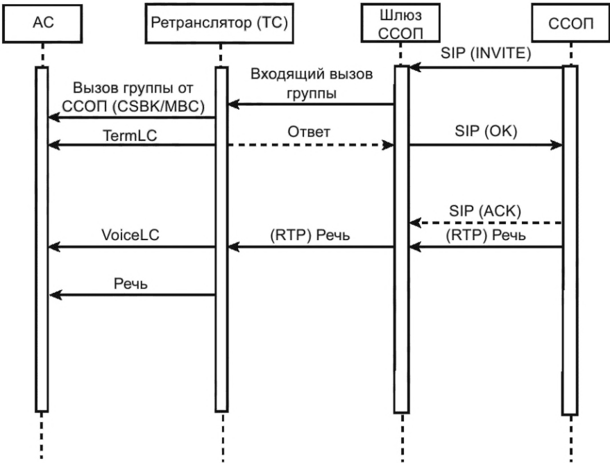
Рисунок А.6 — Последовательность установки соединения с телефонным шлюзом ССОП при групповом вызове
