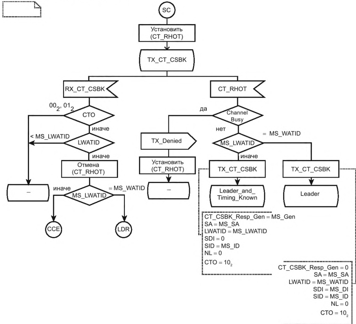
Рисунок 85 — SDL для процедуры SC
