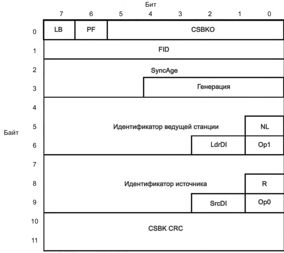
Рисунок 129 — Структура CT_CSBBK PDU
