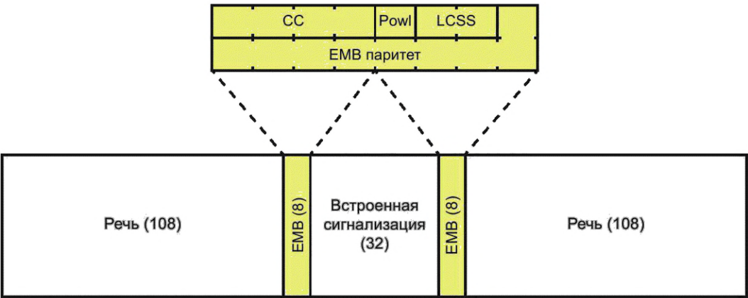
Рисунок 57 — Речевой пакет со встроенной сигнализацией
