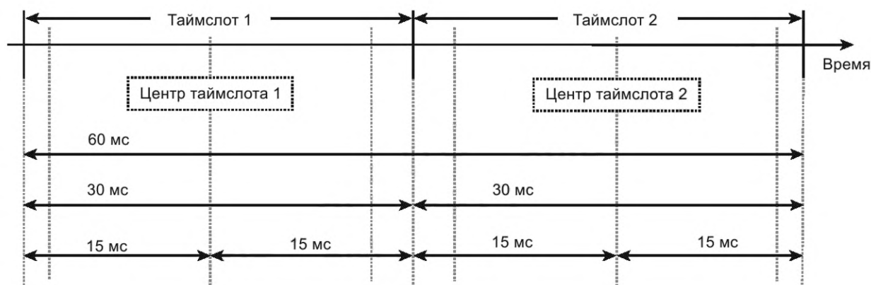
Рисунок 131 — TDMA-кадр
