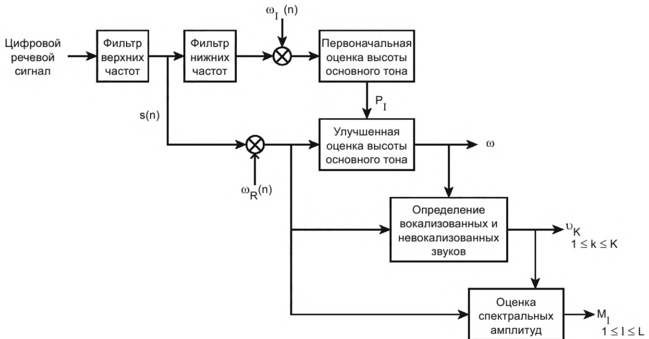
Рисунок К.1 — Структурная схема алгоритма анализа речи
