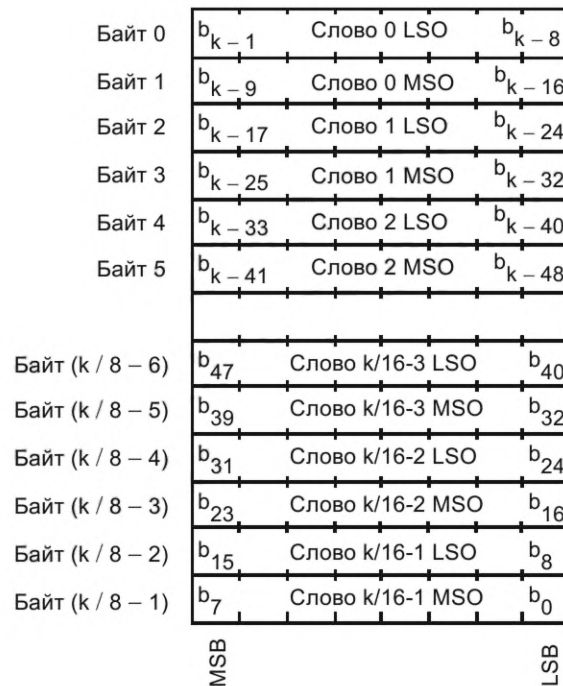
Рисунок Б.10 — Пользовательские данные и байты заполнения, расположенные как восьмиразрядные слова в «линейном» формате
