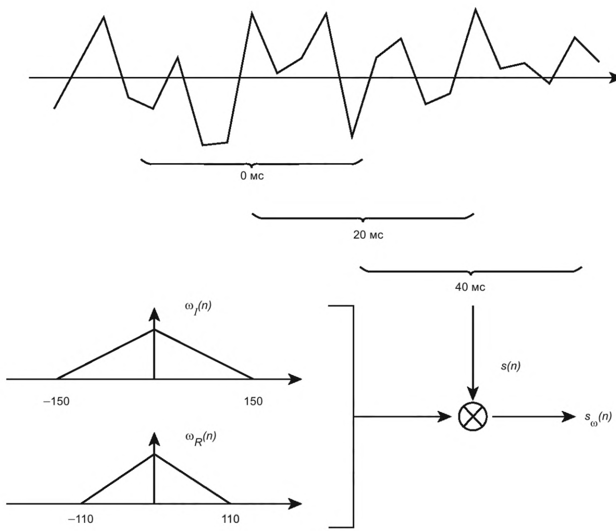
Рисунок К.3 — Алгоритм выравнивания окон
