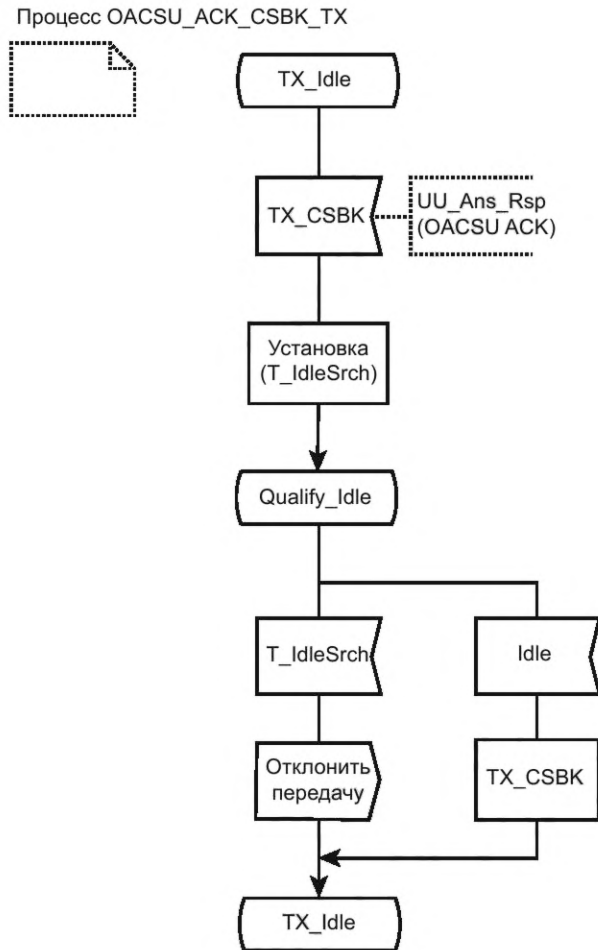
Рисунок 104 — SDL для доступа к каналу UU_Ans_Rsp
