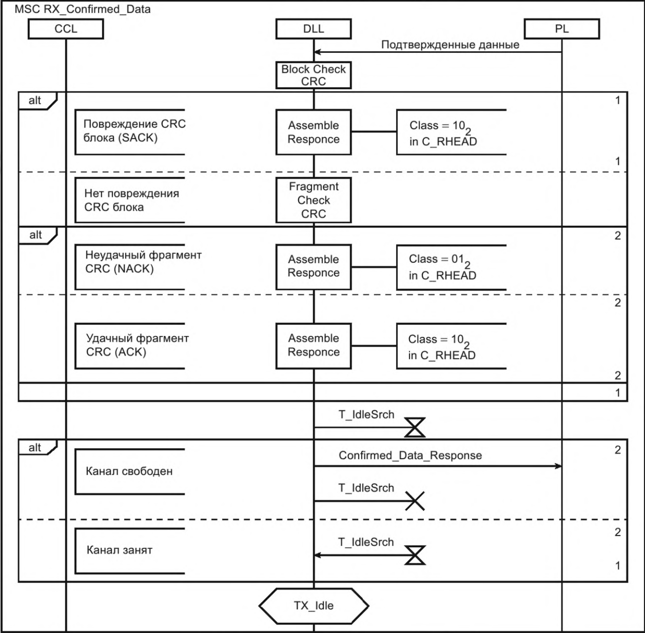
Рисунок 49 — MSC приема подтверждаемых данных
