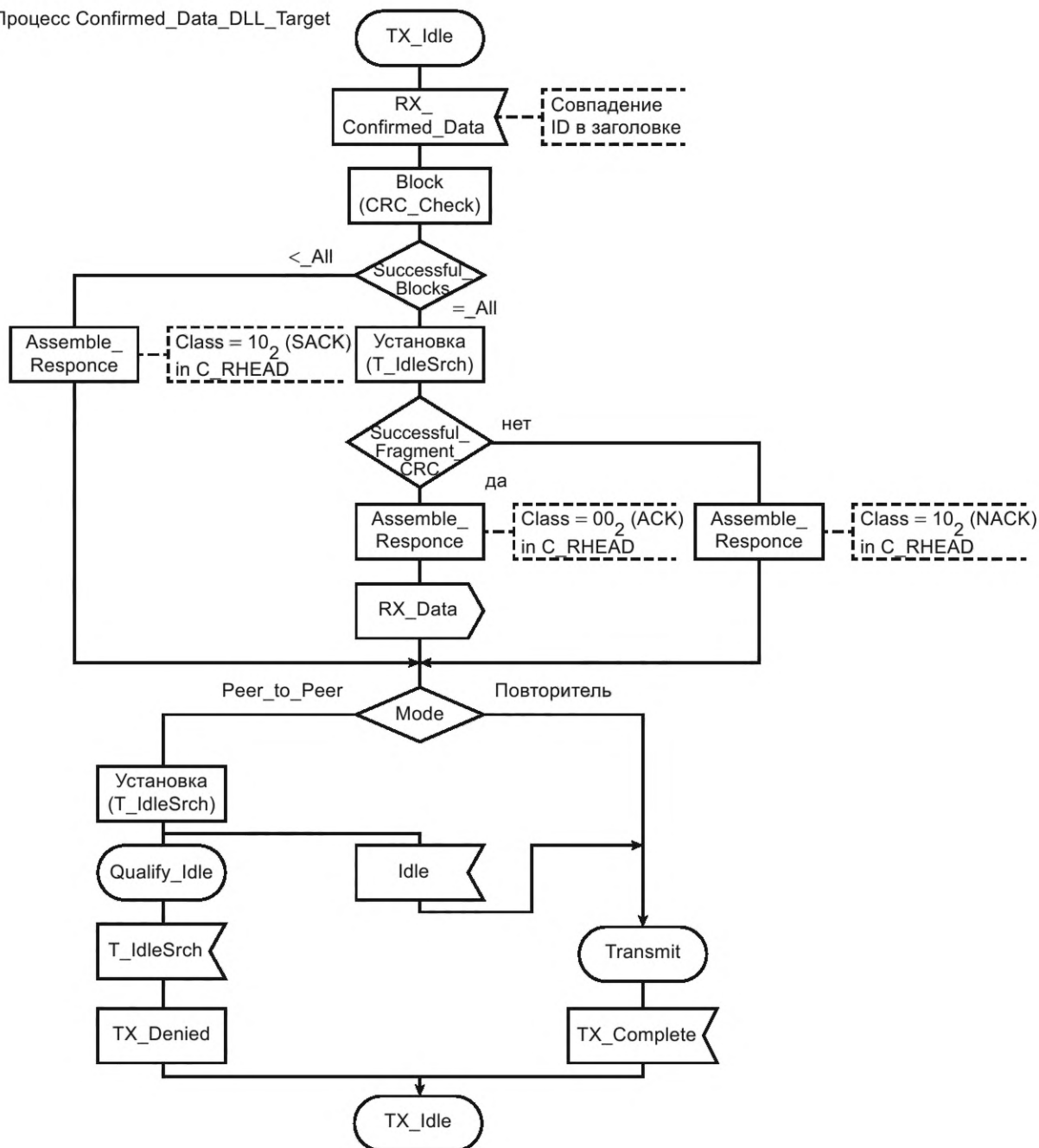
Рисунок 46 — SDL-диаграмма передачи подтверждаемых данных принимающей стороной (Target confirmed data transmission SDL)
