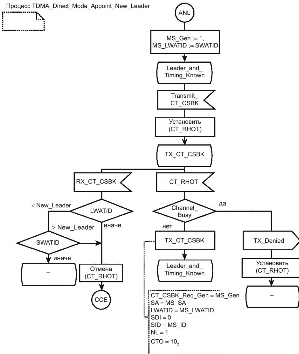
Рисунок 87 — SDL для процедуры ANL
