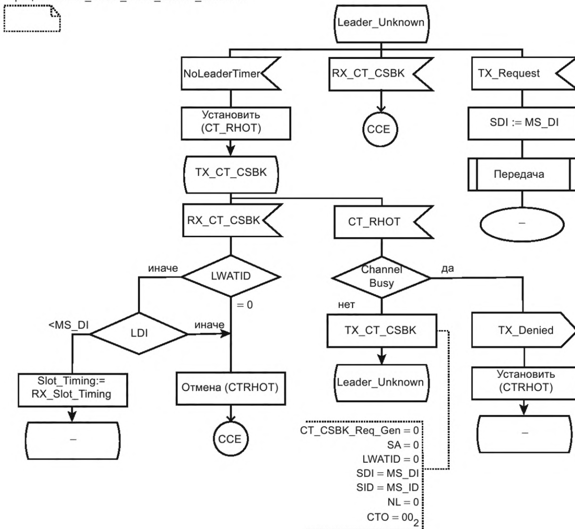
Рисунок 80 — SDL для состояния Leader_Unknown
