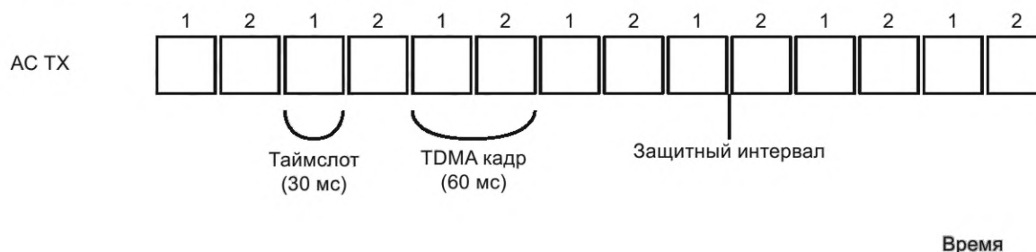
Рисунок 19 — Обобщенная временная диаграмма TDMA
