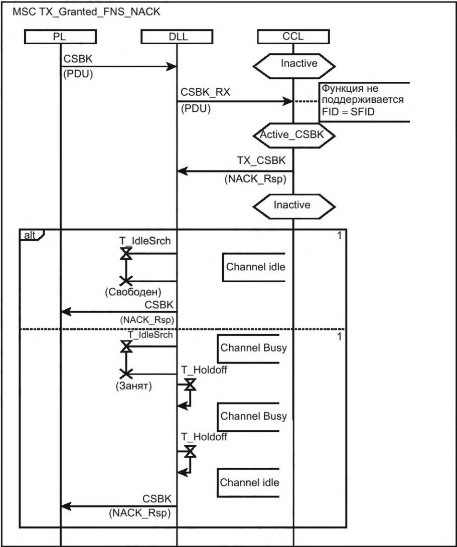
Рисунок 90 — MSC для NACK_Rsp с доступом к каналу по протоколу LBT
