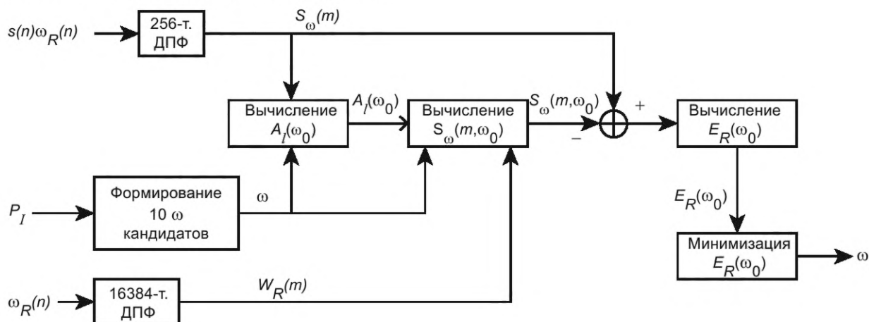
Рисунок К.5 — Улучшения высоты тона
