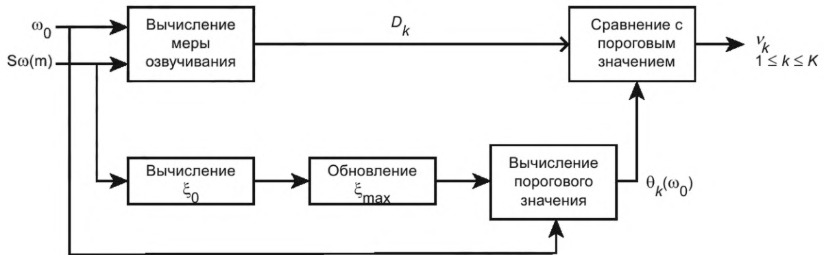
Рисунок K.6 — Определения вокализованной/невокализованной полосы частот
