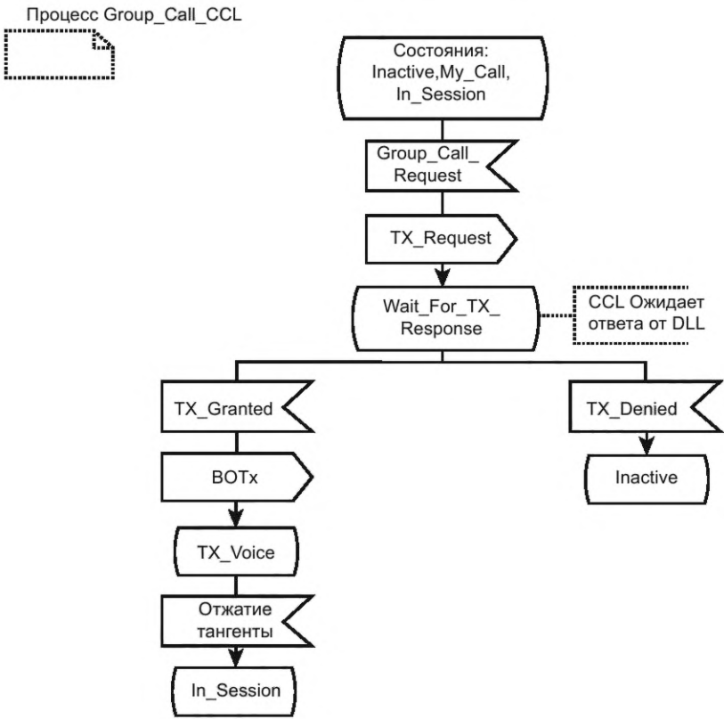
Рисунок 91 — SDL для процесса CCL передачи группового вызова
