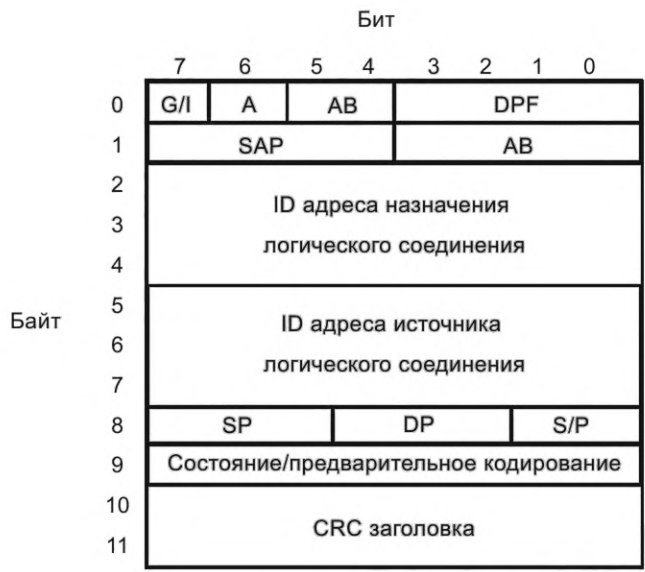
Рисунок 114 — Специальный первый блок заголовка коротких данных состояния/предварительного кодирования
