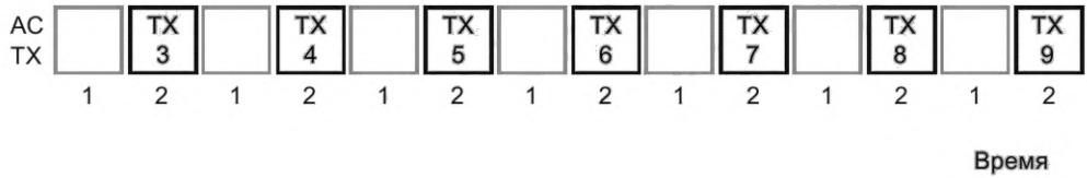
Рисунок 32 — Временная диаграмма прямого режима TDMA
