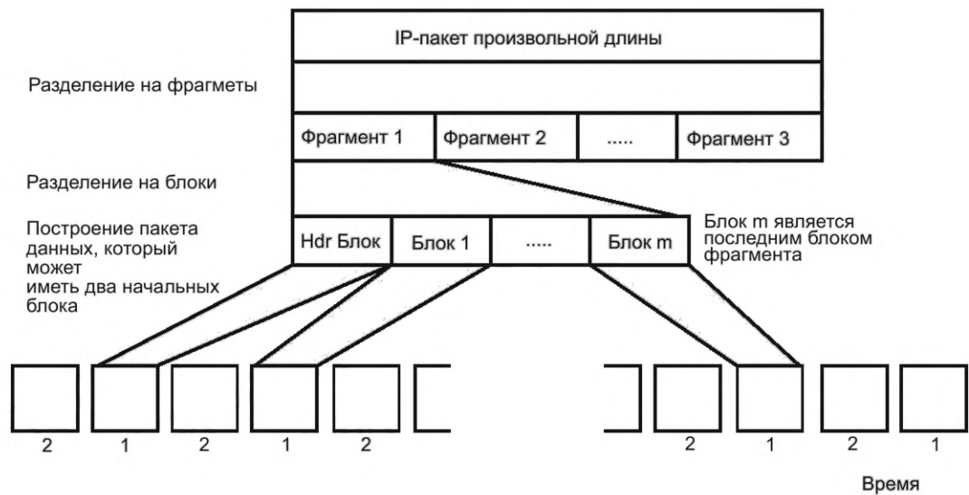
Рисунок 108 — Фрагментация IP-пакета
