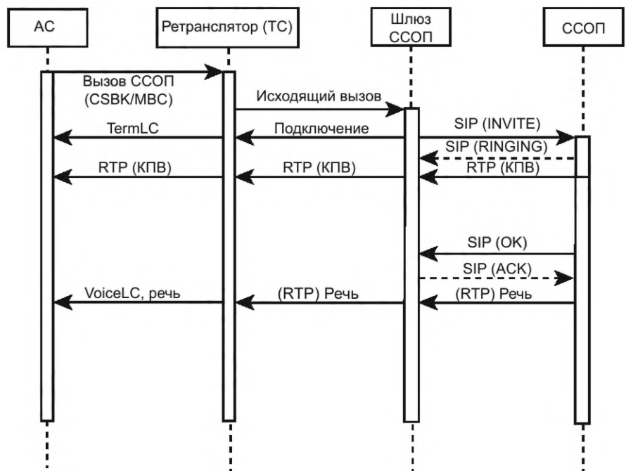
Рисунок А.2 — Последовательность установки соединения со шлюзом ССОП
