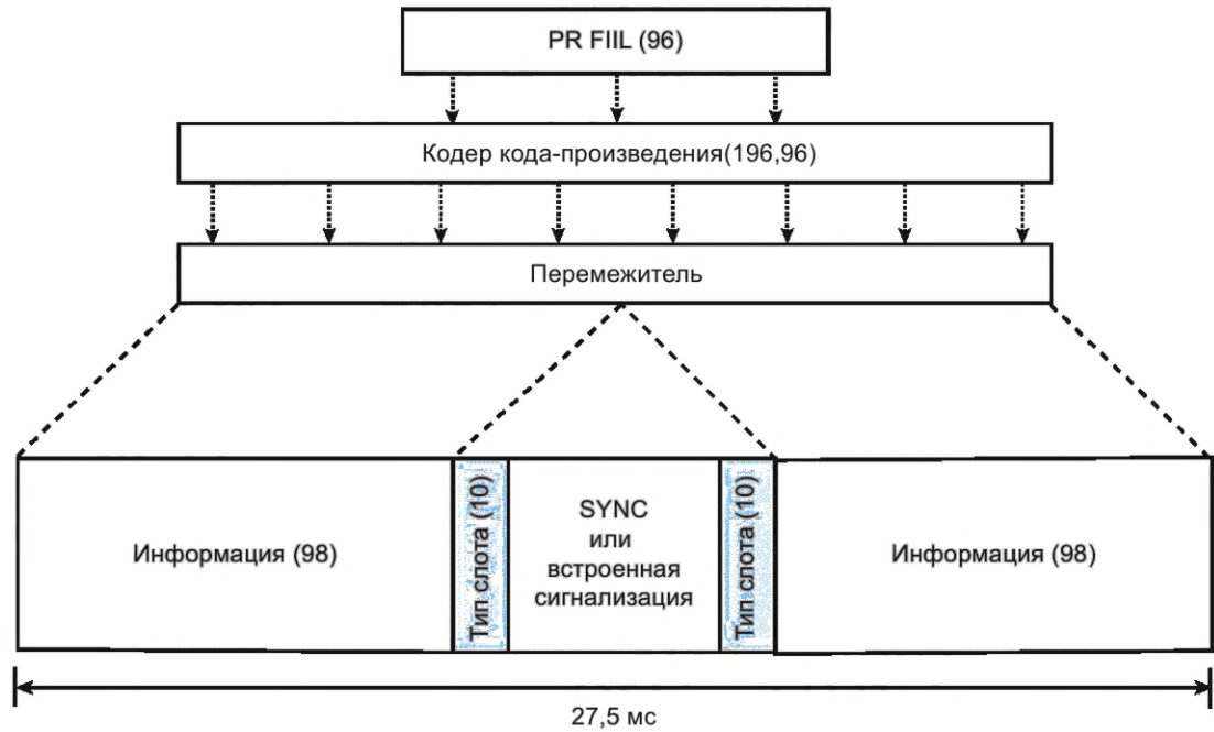
Рисунок 70 — Формирование сообщения Idle
