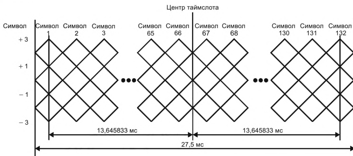
Рисунок 133 — Расположение во времени символов общего пакета в таймслоте
