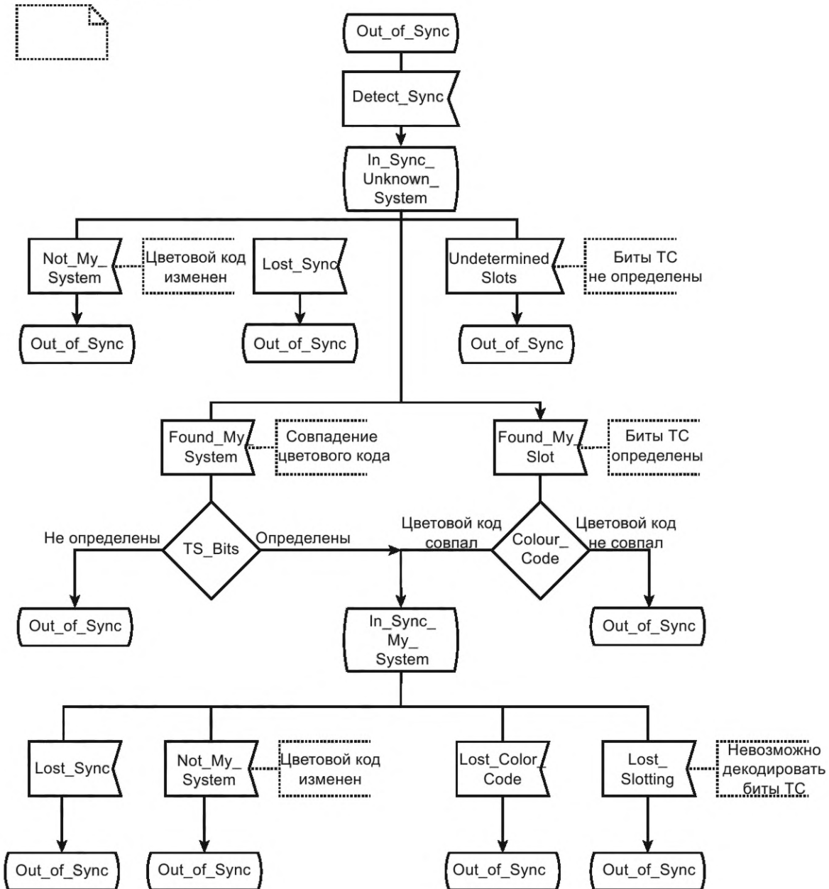
Рисунок Е.2 — SDL-диаграмма AC уровня 1, режим ретранслятора
