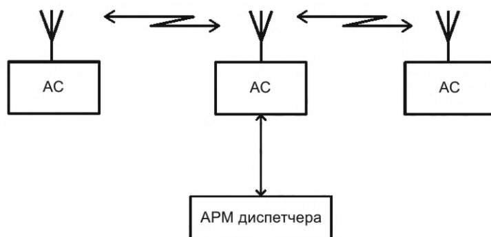
Рисунок 2 — Структурная схема организации подвижной радиосвязи в прямом режиме с АРМ диспетчера
