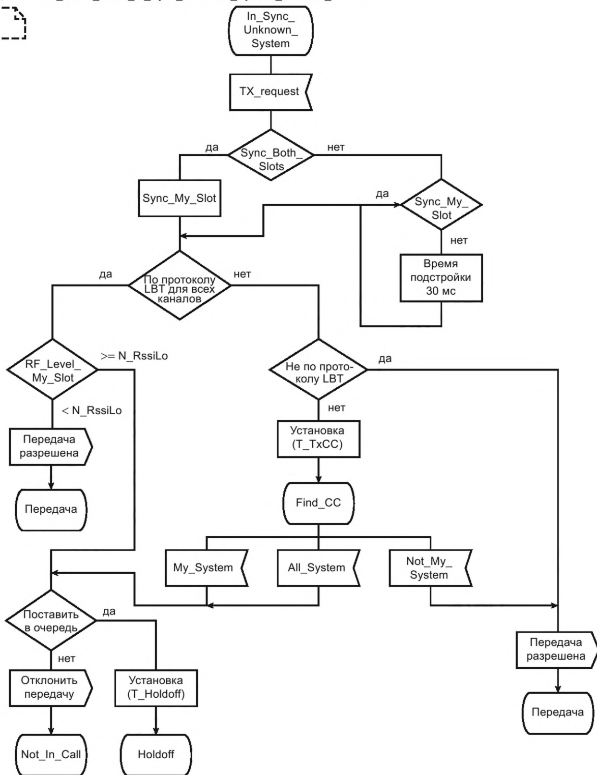
Рисунок 39 — SDL-диаграмма In_Sync_Unknown_System
