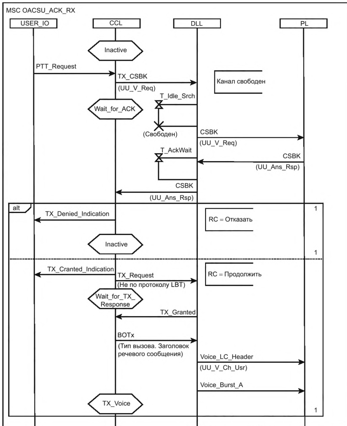
Рисунок 107 — Индивидуальный вызов по методу OACSU, когда получено ACK
