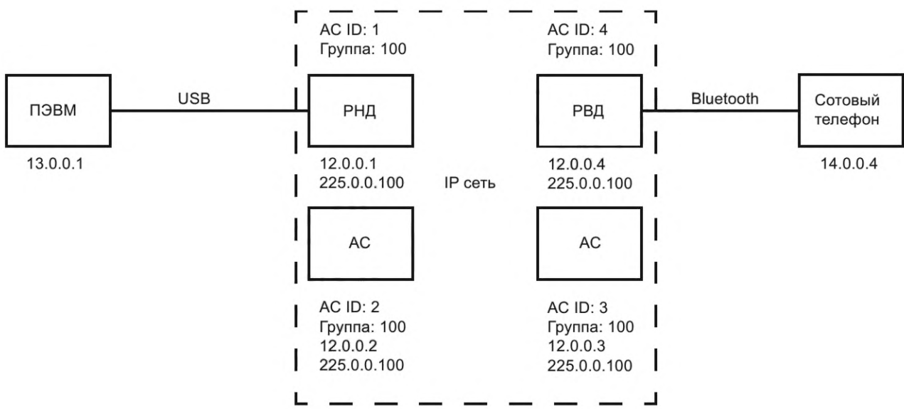
Рисунок А.7 — Пример IPv4-радиосети
