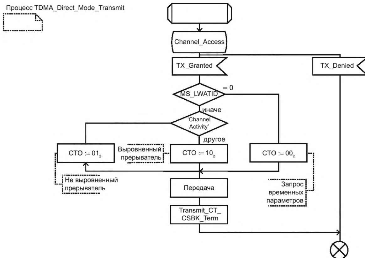
Рисунок 89 — SDL для процедуры передачи
