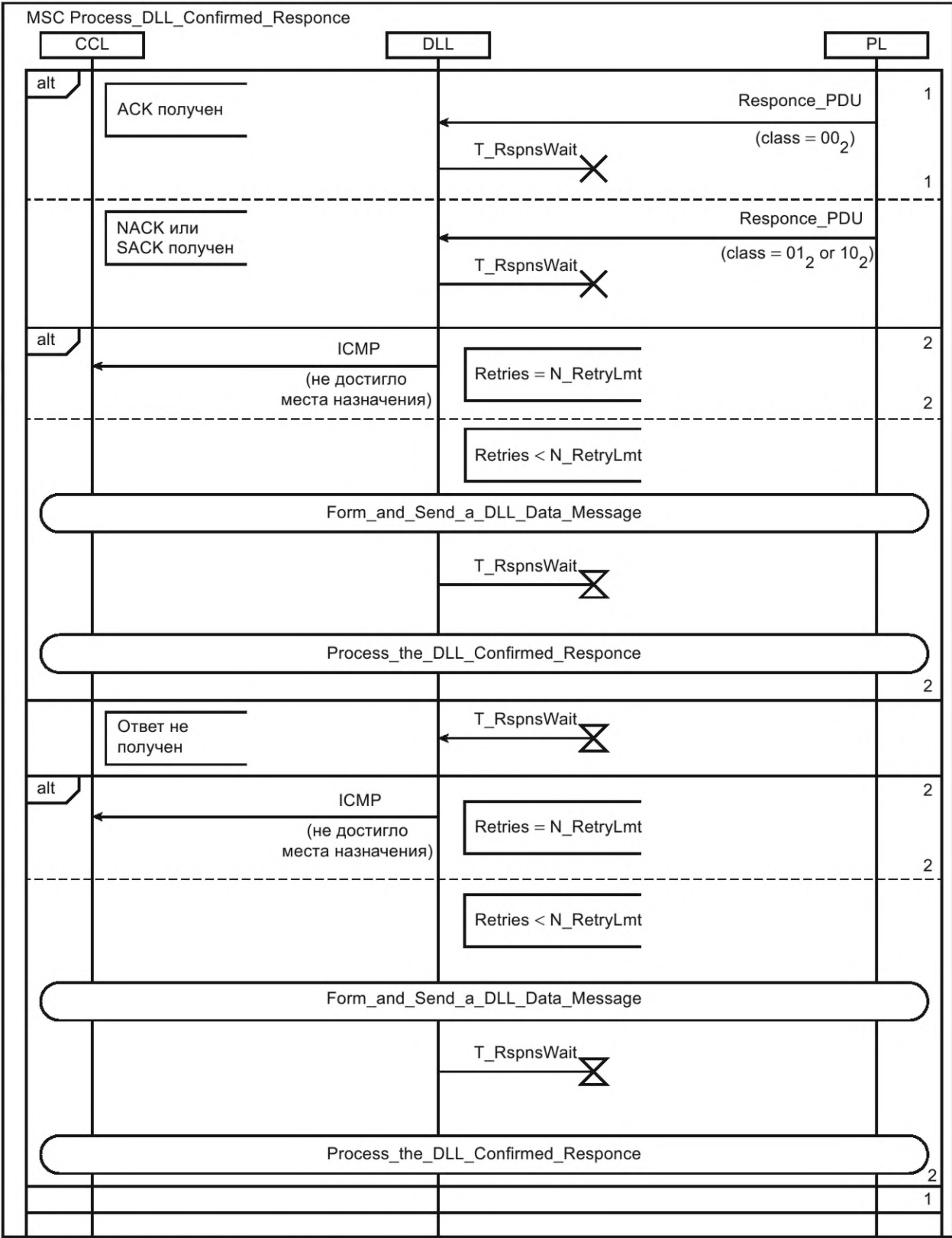
Рисунок 48 — MSC формирования DLL ответа на получение подтверждаемых данных
