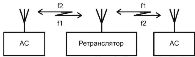
Рисунок 7 — Режим двухчастотной ретрансляции
