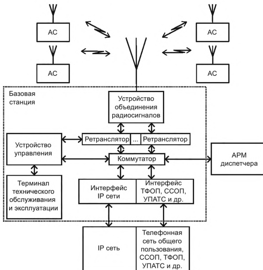
Рисунок 11 — Базовая станция
