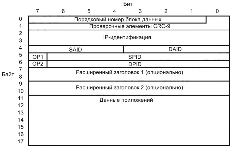
Рисунок 52 — Структура первого блока неподтверждаемых данных с FEC, со скоростью кодирования \frac{1}{2} и со сжатием заголовка UDP/IPv4
