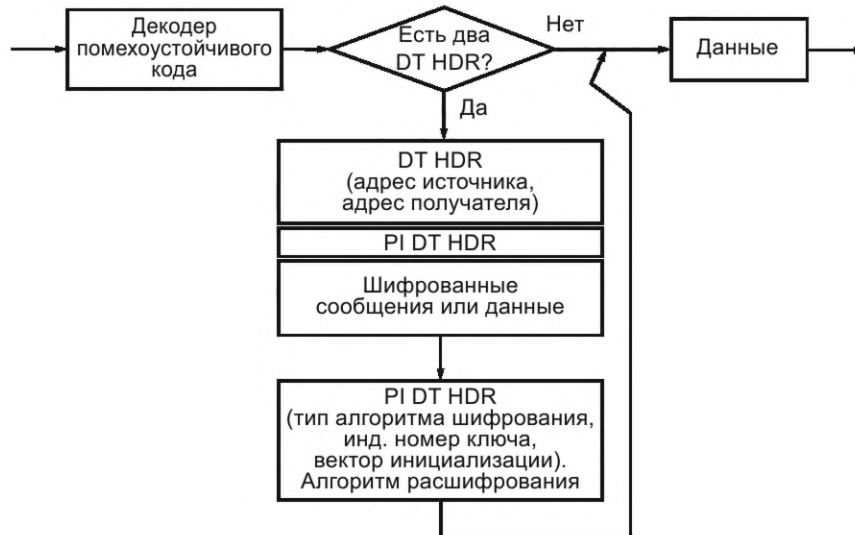
Рисунок 17 — Структурная схема расшифрования сообщений и данных в АС
