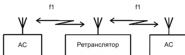
Рисунок 6 — Режим одночастотной ретрансляции
