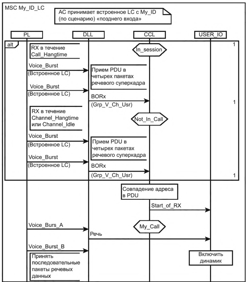
Рисунок 97 — MSC для My_ID_LC
