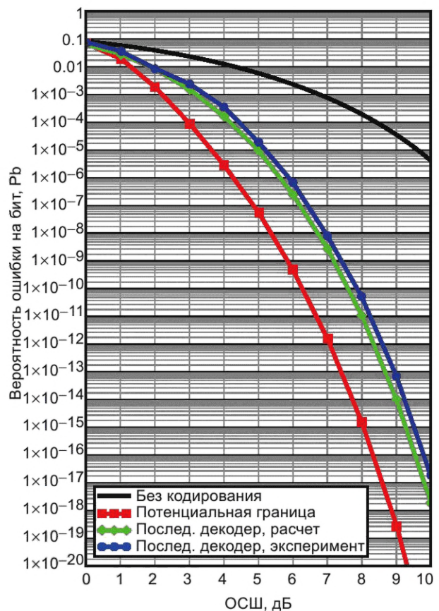
б) Графики вероятности ошибки кода-произведения (196, 96) (потенциальная граница и последовательный декодер). ВРТС (196,96), постоянная скорость
