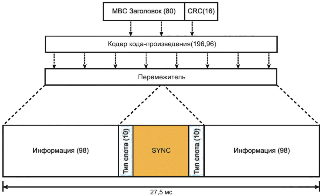
Рисунок 74 — Структура заголовка МВС
