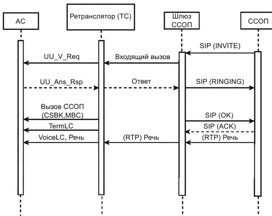
Рисунок А.4 — Последовательность установки соединения от шлюза ССОП к АС
