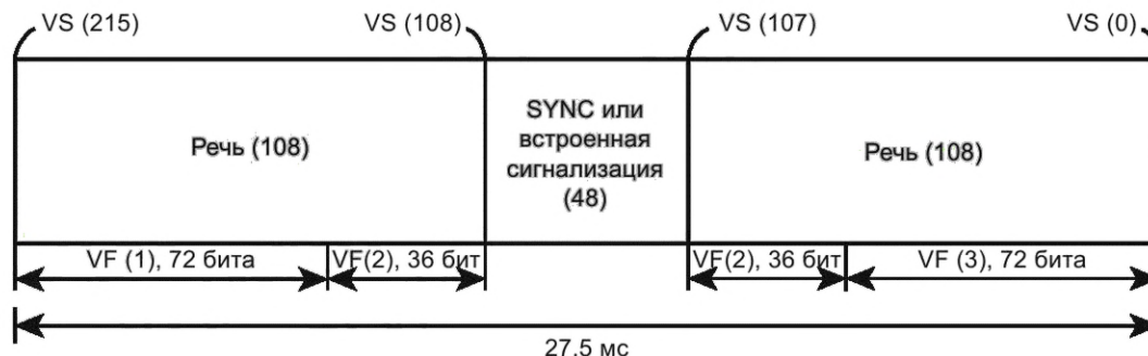
Рисунок 55 — Структура речевого пакета
