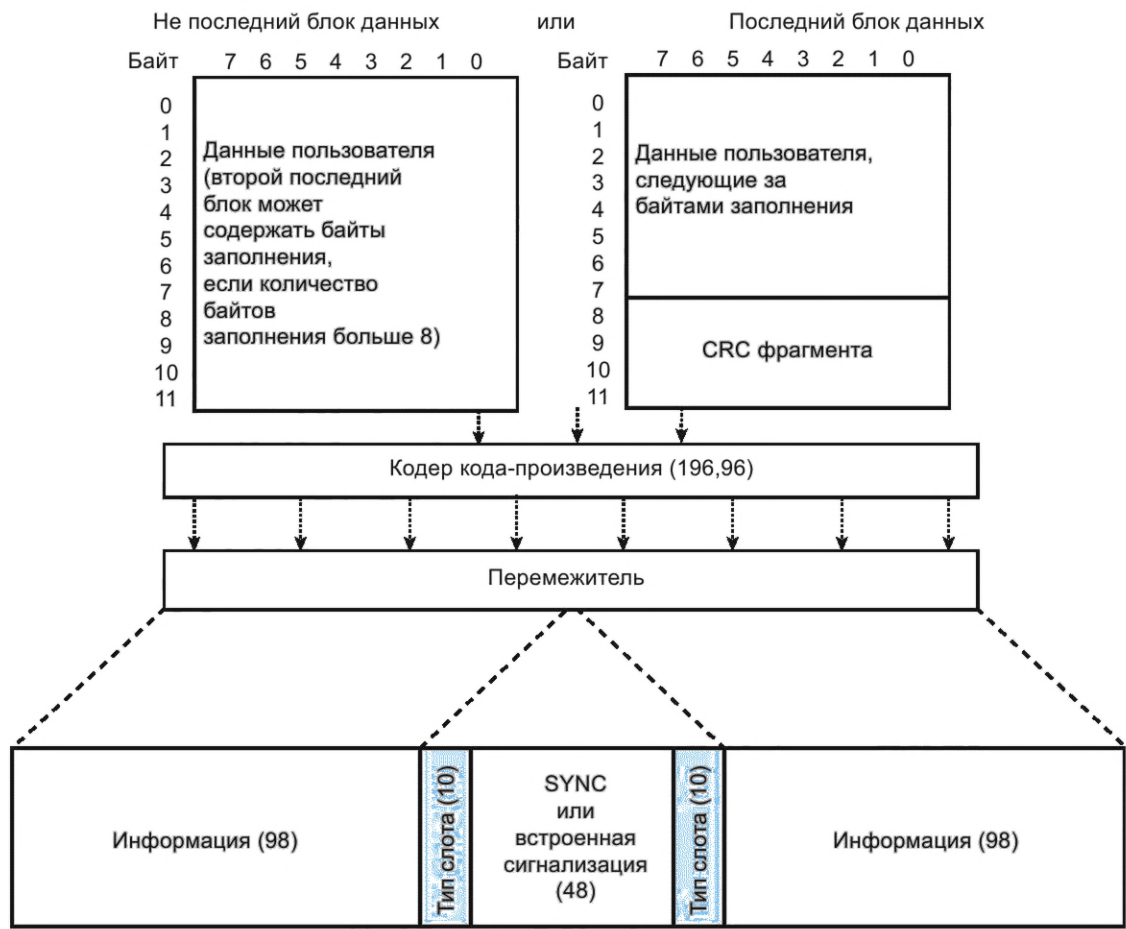
Рисунок 118 — Формат блока данных без подтверждения с FEC со скоростью кодирования \frac{1}{2}
