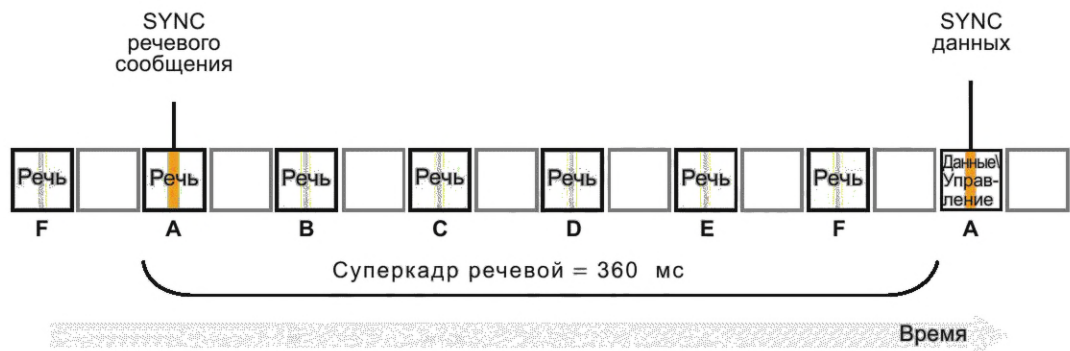
Рисунок 28 — Окончание передачи речи
