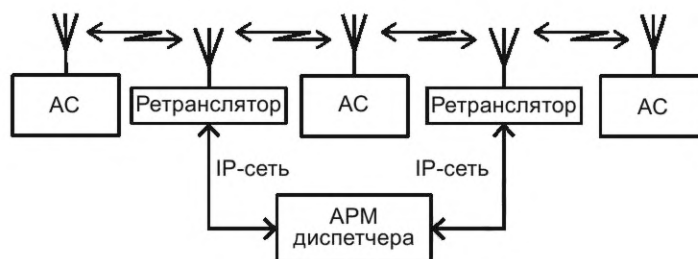
Рисунок 5 — Структурная схема организации ППР с использованием ретрансляторов и АРМ диспетчера
