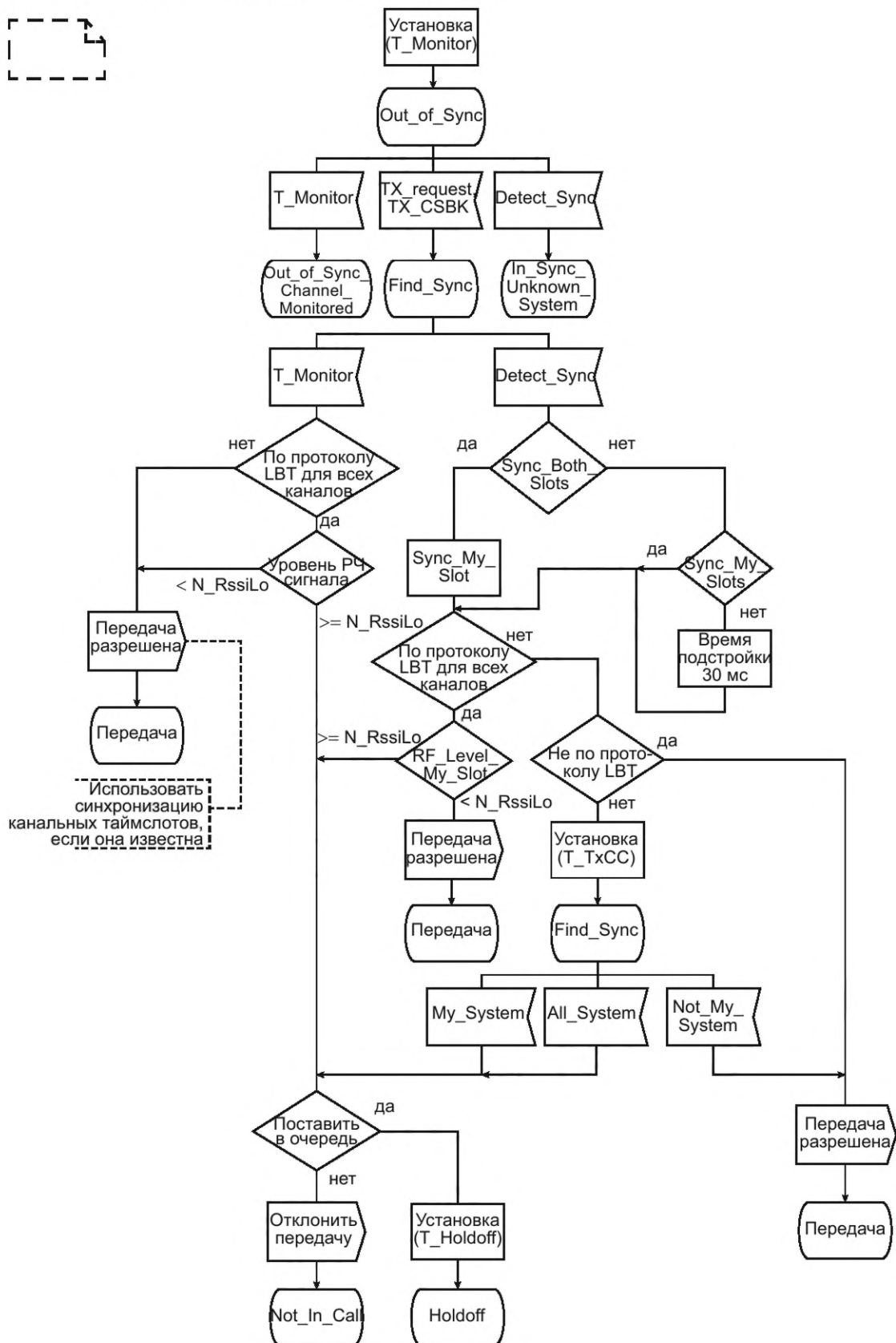
Рисунок 37 — SDL-диаграмма Out_of_Sync
