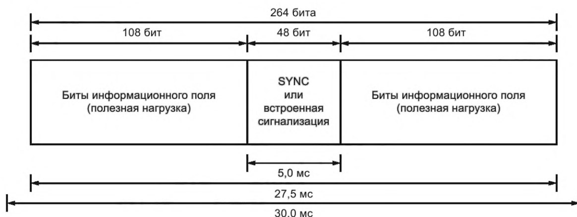
Рисунок 20 — Структура речевого пакета
