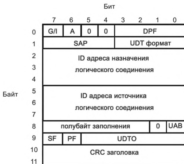
Рисунок 117 — Специальный первый блок заголовка для пакета UDT
