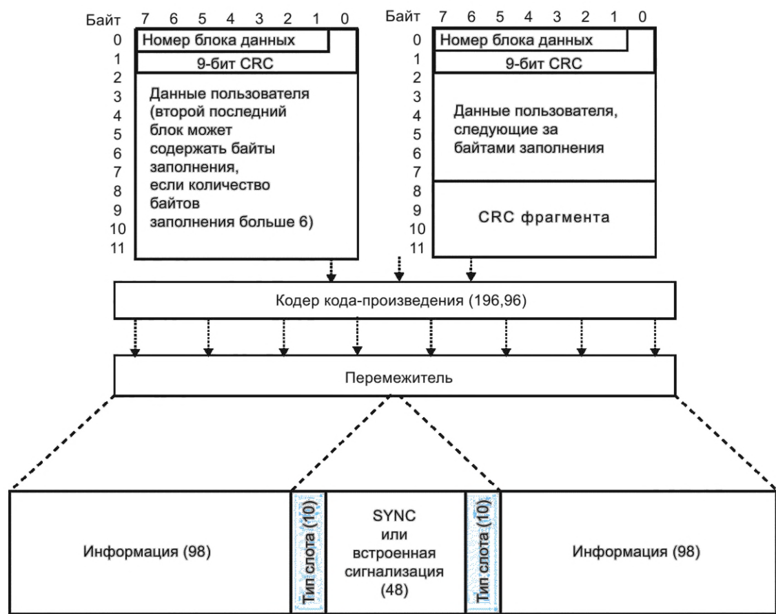
Рисунок 122 — Формат блока данных с подтверждением и FEC со скоростью кодирования 1/2
