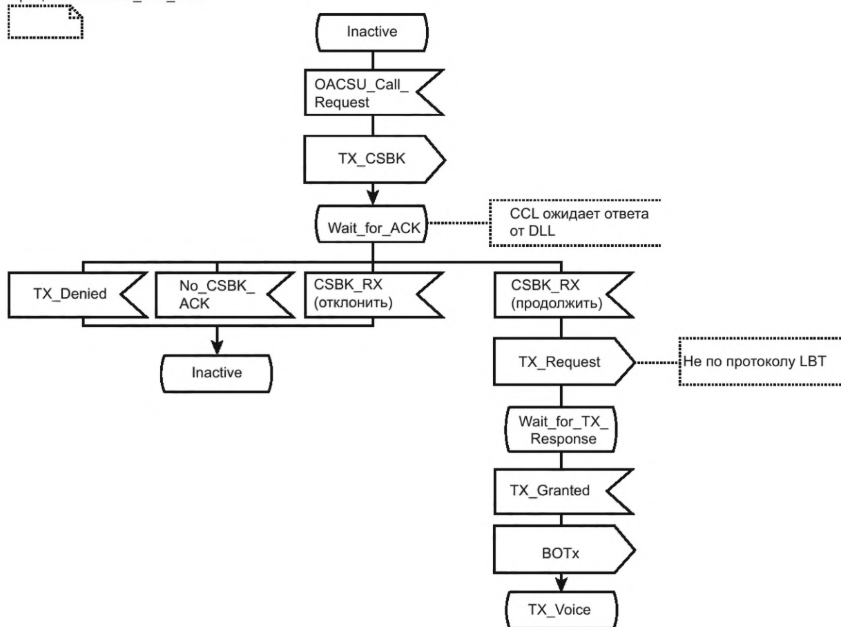
Рисунок 105 — SDL индивидуального вызова с CCL источника по методу OACSU
