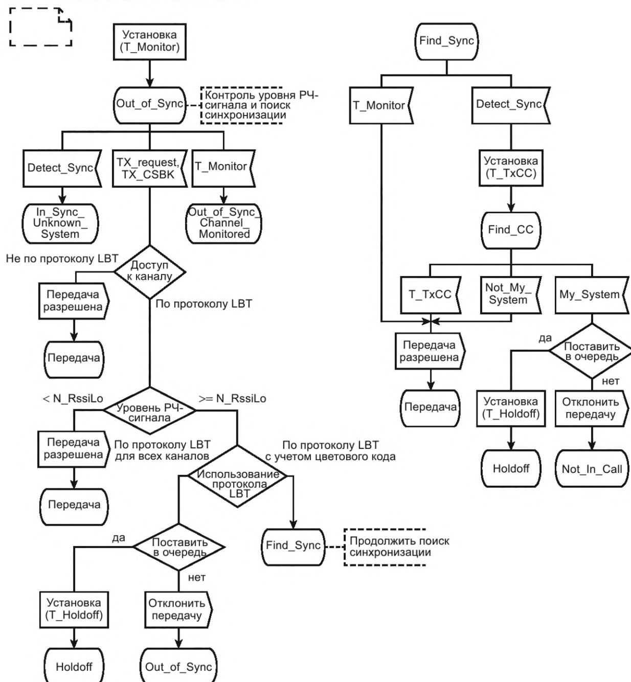
Рисунок 33 — SDL-диаграмма Out\_of\_Sync
