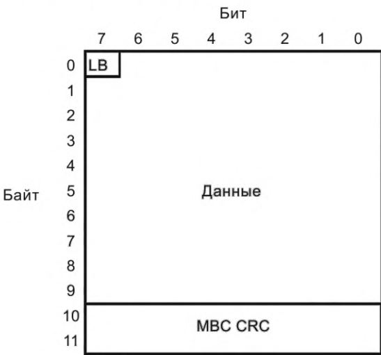
Рисунок 73 — Структура последнего блока MBC
