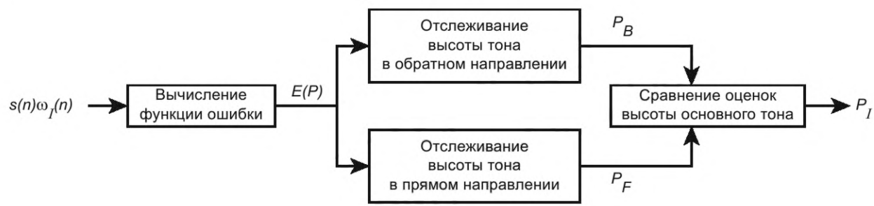
Рисунок К.4 — Первоначальная оценка высоты тона
