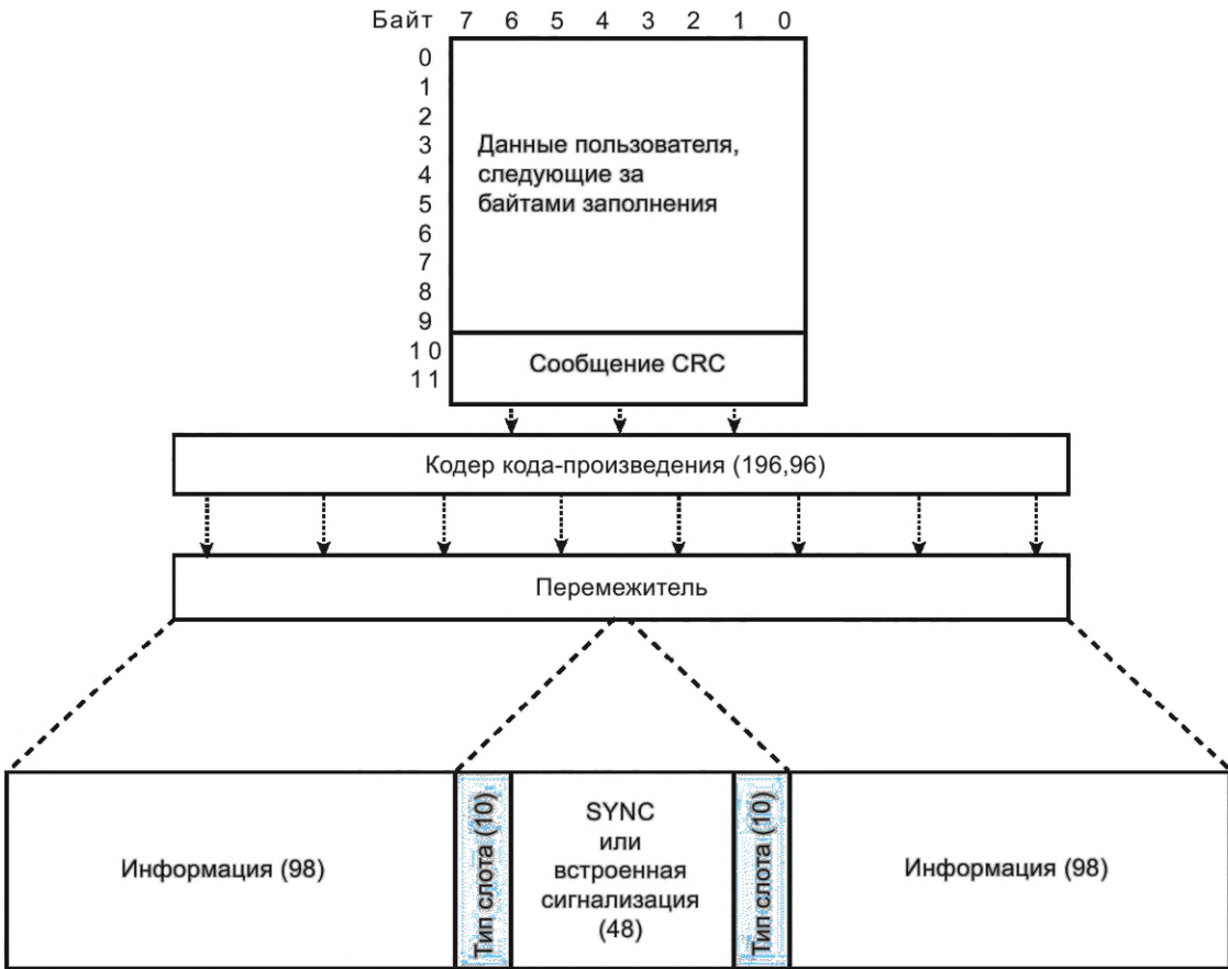
Рисунок 126 — Формат последнего блока данных UDT
