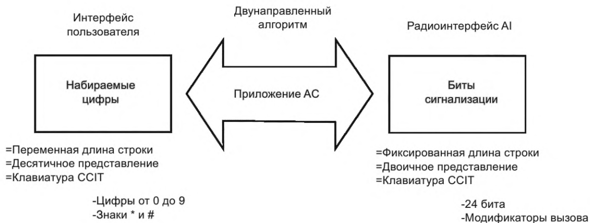
Рисунок А.11 — Преобразование набираемого номера
