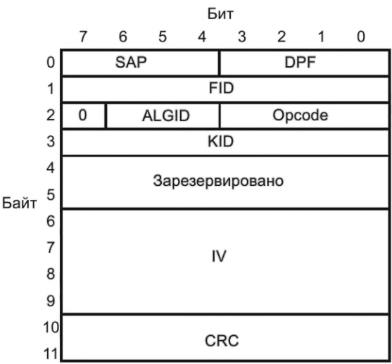
Рисунок 66 — Структура сообщения PI DT PDU
