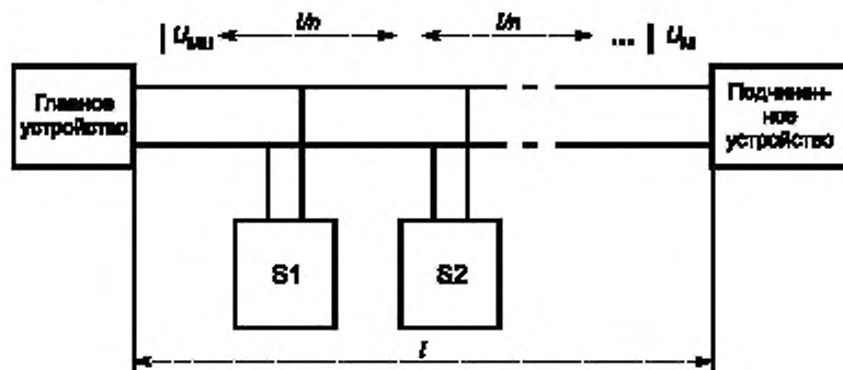
Рисунок В.3 — Тестовое оборудование для M-Bus ( l )
