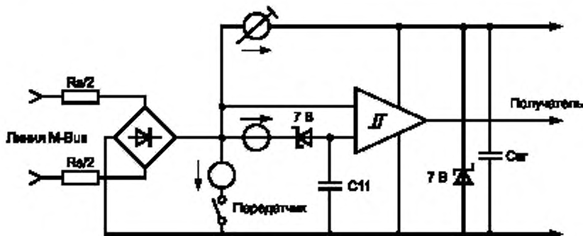
Рисунок 2 — Схема для интерфейса M-Bus
