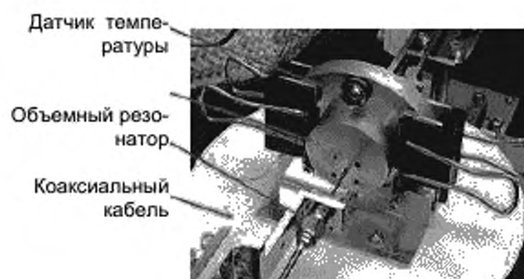
Рисунок 6 — Фото резонатора для измерений в области 10 ГГц
