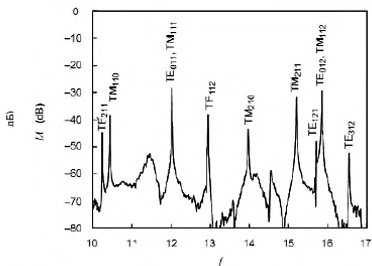
Рисунок 8 – Спектр резонансных частот резонатора
