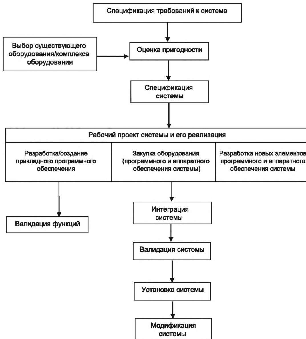
Рисунок 1 — Жизненный цикл системы (по МЭК 61513, для справки)
