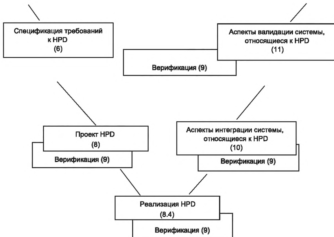
Рисунок 2 — Жизненный цикл разработки HPD
