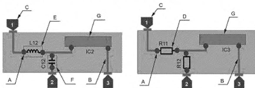
А — подключение к встроенному компоненту; В — проводящий рисунок; С — контрольная точка зонда; D — резистор; E — дроссель; F — конденсатор; G — микросхема (IC), большая микросхема (LSI)
