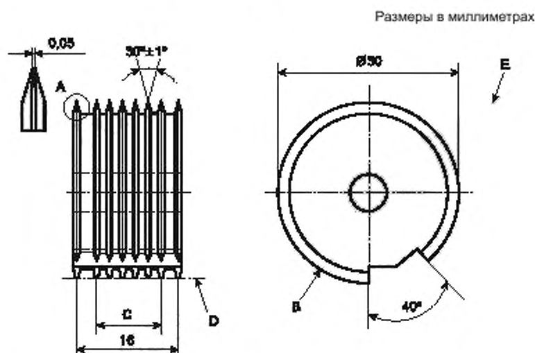
Рисунок 9 — Нож для нарезки
