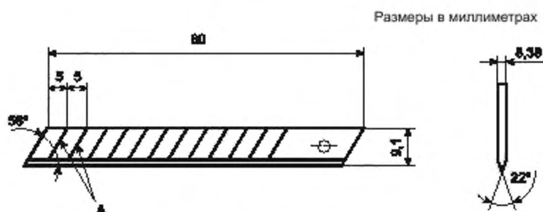
Рисунок 8 — Единичный инструмент
