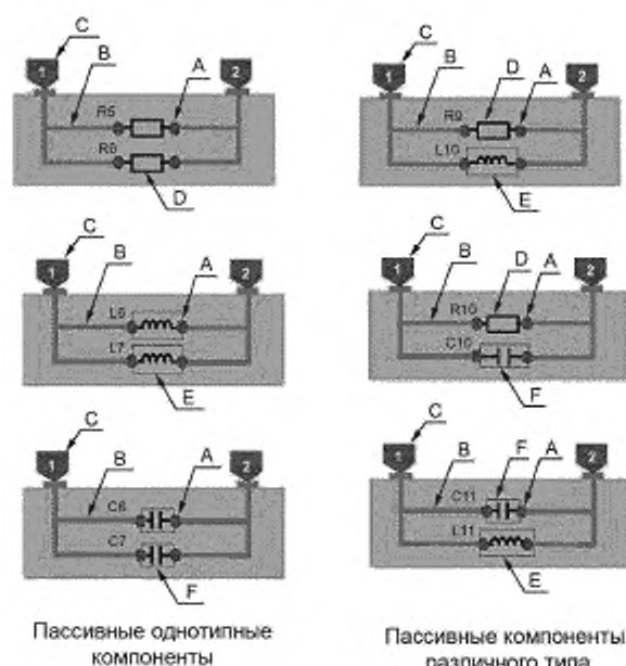
Рисунок 21 — Конструкция схемы для параллельного соединения пассивных компонентов
