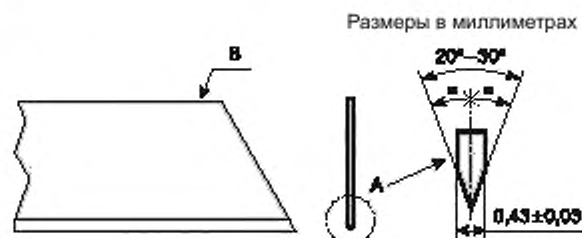
Рисунок 8 — Единичный инструмент
