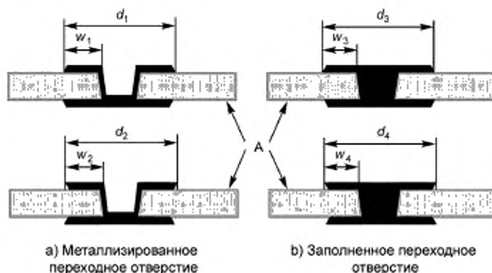
А — изоляционный слой; d_1 — d_5 — максимальный размер контактной площадки w_1 — w_4 — пояс контактной площадки во внешнем слое
