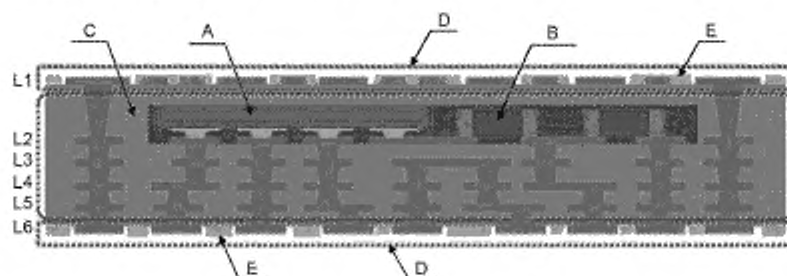
А — встроенный активный компонент; В — встроенный пассивный компонент; С — внутренний слой; D — внешний слой; E — паяльная маска
