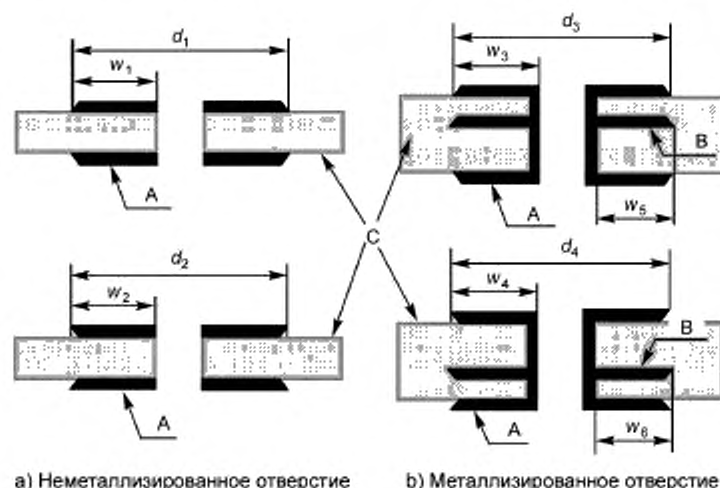
А — неметаллизированное отверстие; В — металлизированное отверстие, С — переходное отверстие в слое наращивания в соответствующей форме: d_1 — d_4 — максимальный размер контактной площадки, w_1 — w_4 — пояска контактной площадки во внешнем слое, w_5 , w_6 — пояска контактной площадки во внутреннем слое
