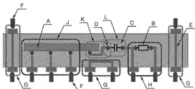
Рисунок 17 — Типовая схема построения платы со встроенными компонентами
