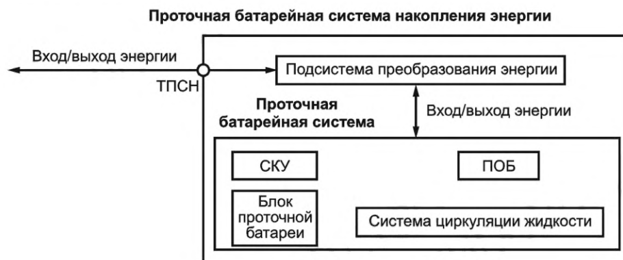
Рисунок 1 — Пример архитектуры СНЭБП
