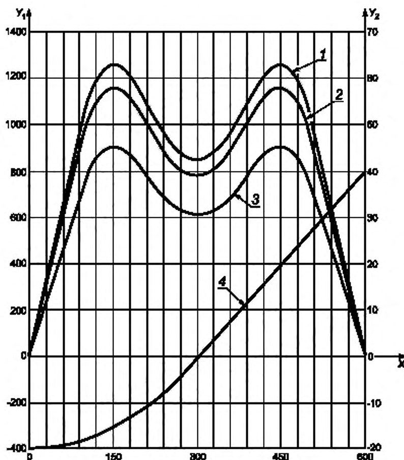
X — время, мс; Y_1 — сила, Н; Y_2 — угол, °; 1 — испытательная сила F для уровня испытательной нагрузки P5; 2 — испытательная сила F для уровня испытательной нагрузки P4; 3 — испытательная сила F для уровня испытательной нагрузки P3; 4 — угол наклона \gamma платформы стола (см. рисунок 5)
