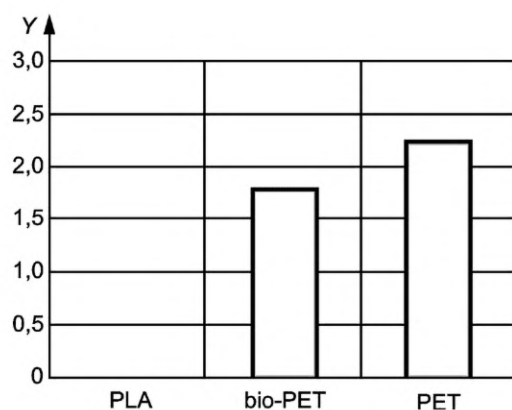
Рисунок 3 — Количество (масса) CO 2 , выделяемого в воздух, на 1 кг утилизированного полимера (B)
