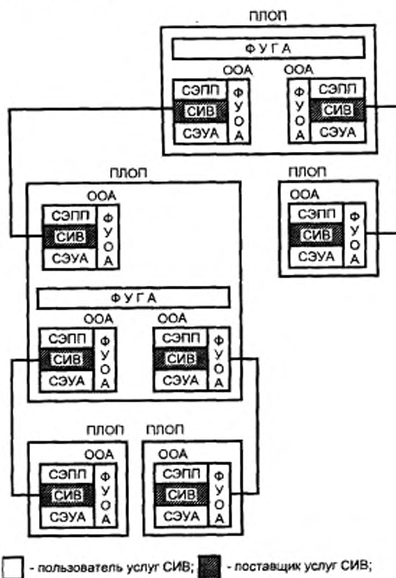
Рисунок В.1 — Архитектура дерева атомарного действия
