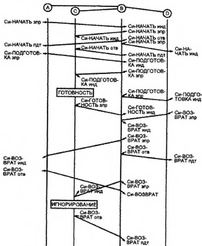
Рисунок С.5 — Последовательность примитивов — ВОЗВРАТ атомарного действия
