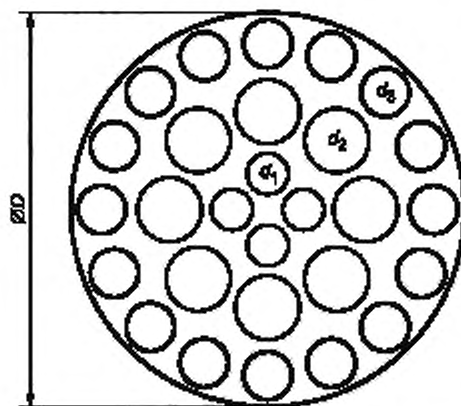
Рисунок В.2 — Выпрямитель потока
