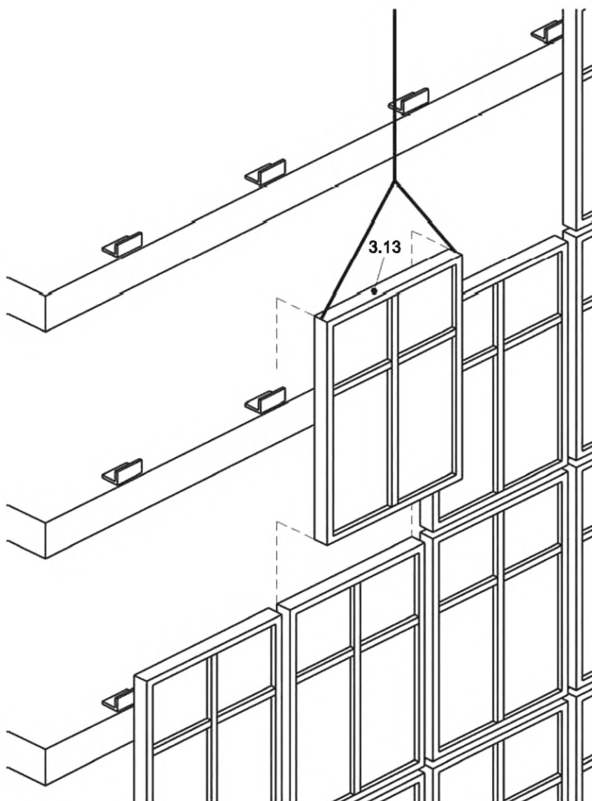
Рисунок А.6 — Пример модульной конструкции
