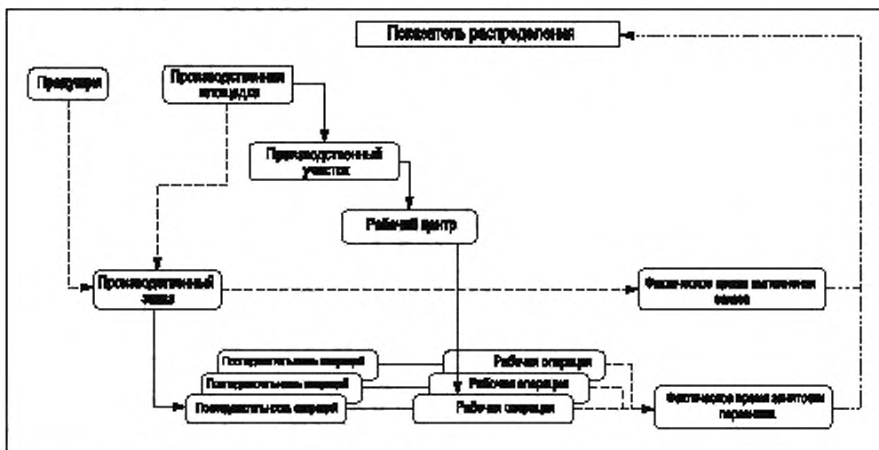
Рисунок A.2 — Диаграмма модели действия элементов KPI-показателя «Показатель распределения»
