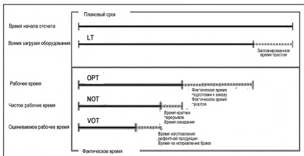
Рисунок В.1 — Временная модель для расчета общей эффективности использования оборудования (OEE)
