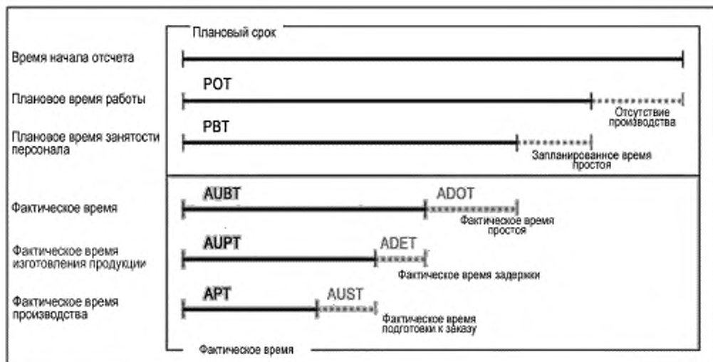
Рисунок 4 — Временные диаграммы рабочих операций
