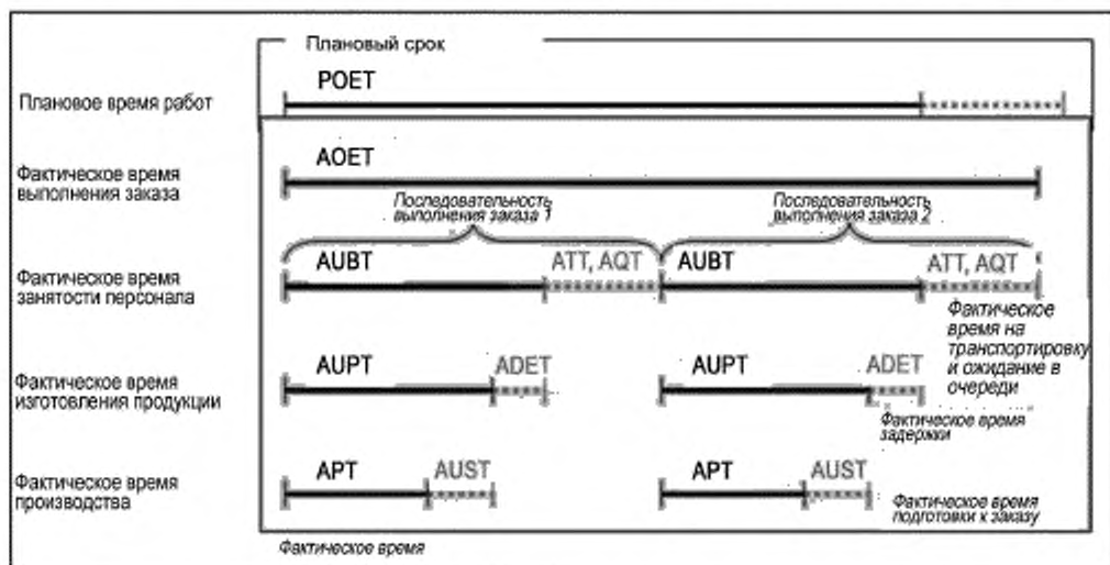
Рисунок 5 — Временные диаграммы работ по производственному заказу
