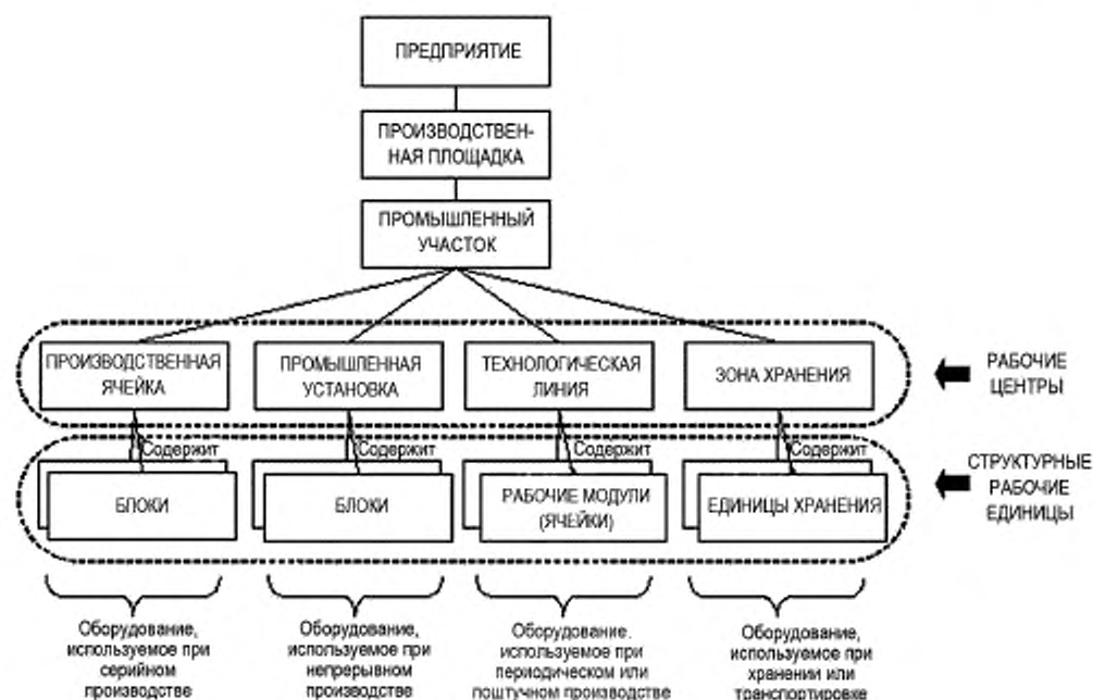
Рисунок 2 — Иерархия оборудования, основанная на ролевом принципе
