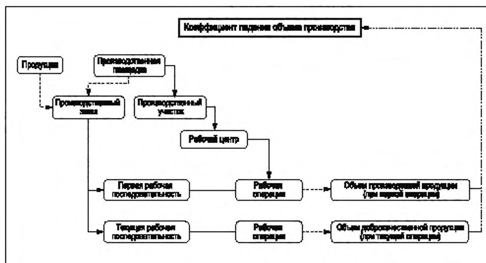
Рисунок А.18 — Диаграмма модели действия элементов KPI-показателя «Коэффициент падения объема производства»
