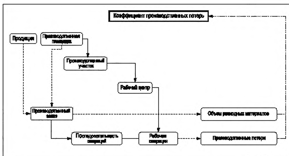
Рисунок А.25 — Диаграмма модели действия элементов KPI-показателя «Коэффициент производственных потерь»
