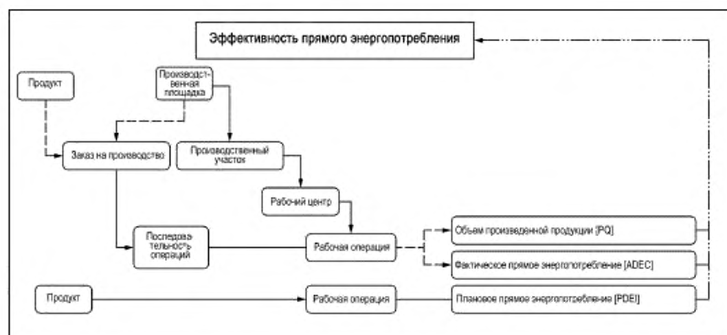
Рисунок А.33 — Эффективность прямого энергопотребления
