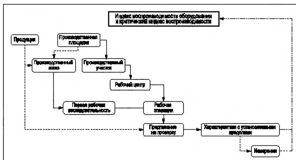
Рисунок А.19 — Диаграмма модели действия элементов KPI-показателя «Индекс воспроизводимости оборудования и критический индекс воспроизводимости оборудования»
