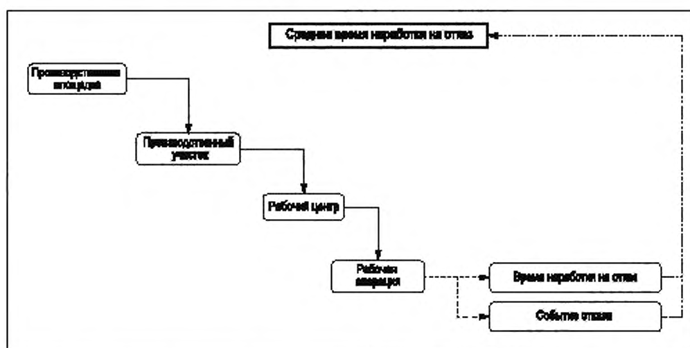
Рисунок А.30 — Диаграмма модели действия элементов KPI-показателя «Среднее время наработки на отказ»
