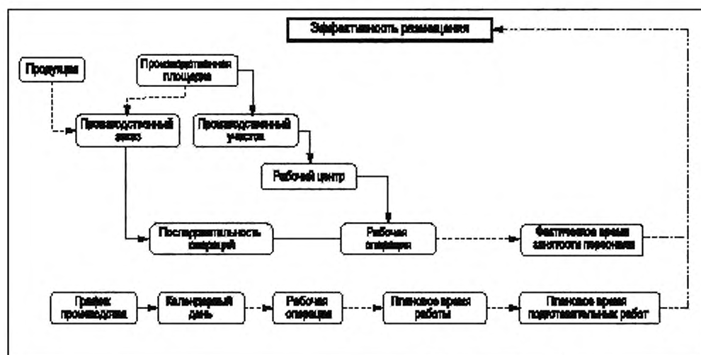
Рисунок А.4 — Диаграмма модели действия элементов KPI-показателя «Эффективность размещения»
