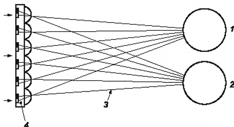
1 — правый глаз; 2 — левый глаз; 3 — матрица цилиндрических линз, формирующая зоны наблюдения, 4 — LCD-монитор со смешанными (наложенными) изображениями
