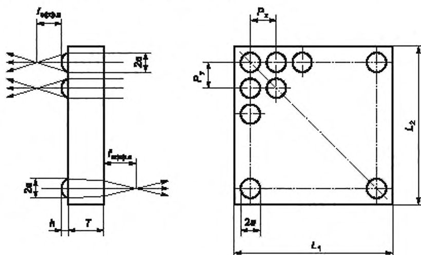
Рисунок 3 — Структура матриц микролинз
