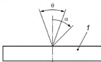
1 — планарный детектор, \Theta — угол расходимости лазерного пучка; \alpha — максимальная угловая апертура
