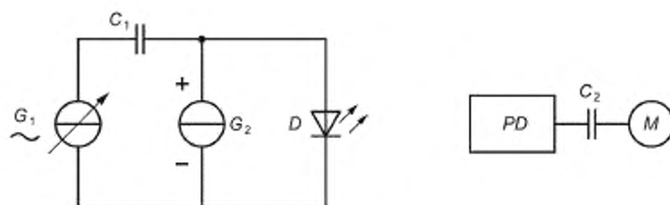
D — измерительное устройство, PD — детектор (например, фотодетектор); M — измеритель мощности переменного тока диодного лазера, G_1 — генератор переменного тока с регулируемой частотой; G_2 — генератор постоянного тока, C_1, C_2 — конденсаторы связи
