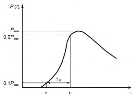
Рисунок 7 — Пример изменения времени нарастания импульса лазерного излучения при проведении измерений
