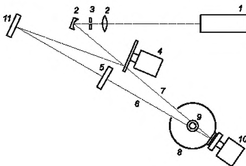
1 — источник лазерного излучения; 2 — телескоп; 3 — точечная диафрагма; 4 — прерыватель; 5 — испытуемый образец; 6 — зондирующий луч; 7 — опорный луч; 8 — интегрирующая сфера; 9 — приемник излучения, установленный сверху интегрирующей сферы; 10 — вращающаяся мишень; 11 — дополнительное зеркало
