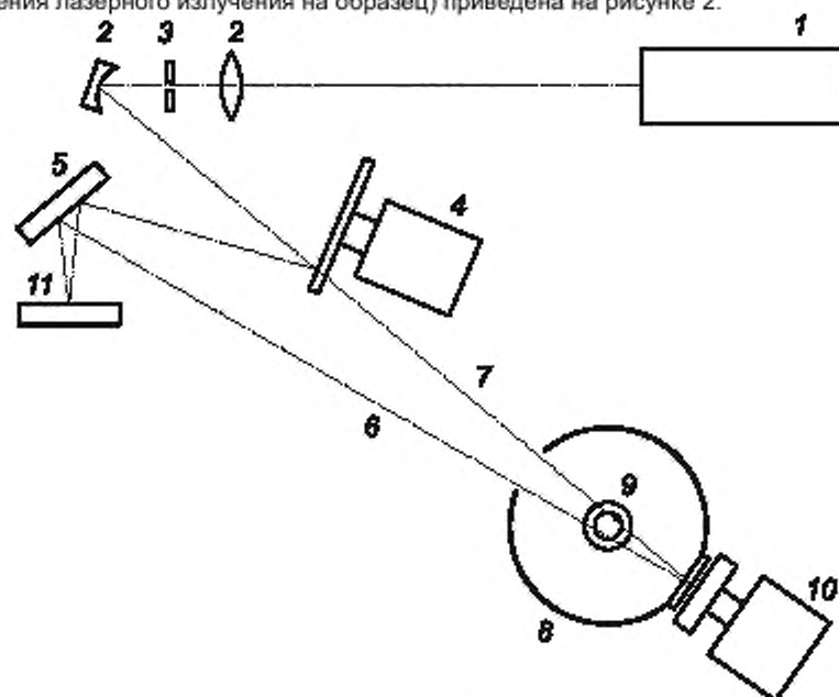
1 — источник лазерного излучения; 2 — телескоп; 3 — точечная диафрагма; 4 — прерыватель; 5 — испытуемый образец; 6 — зондирующий луч; 7 — опорный луч; 8 — интегрирующая сфера; 9 — приемник излучения, установленный сверху интегрирующей сферы; 10 — вращающаяся мишень; 11 — дополнительное зеркало
