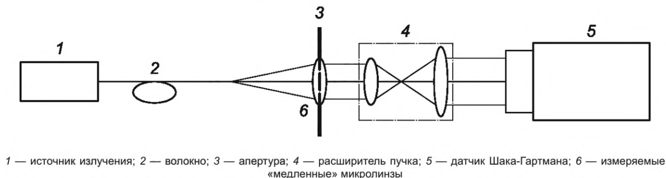
Рисунок D.2 — Схема установки для измерений aberrаций волнового фронта «медленных» микролинз
