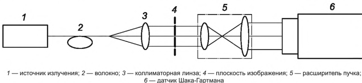
Рисунок D.1 — Схема установки для измерений опорного волнового фронта
