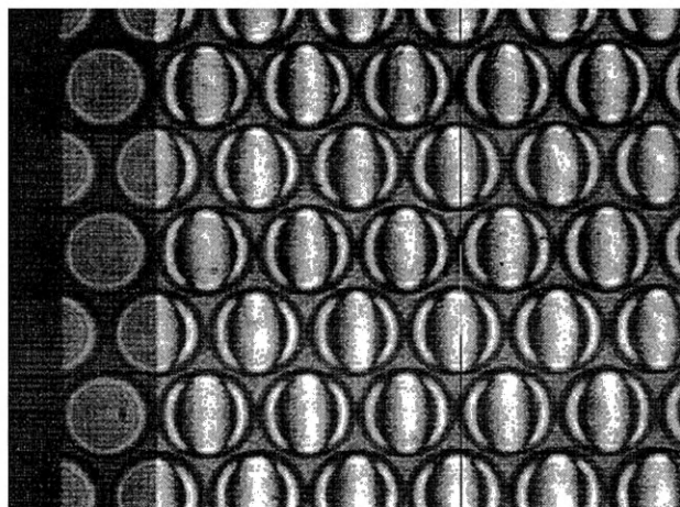
б) Сдвиг изображений микролинз на один шаг в матрице [по сравнению с рисунком а)], показывающий сферические aberrации
